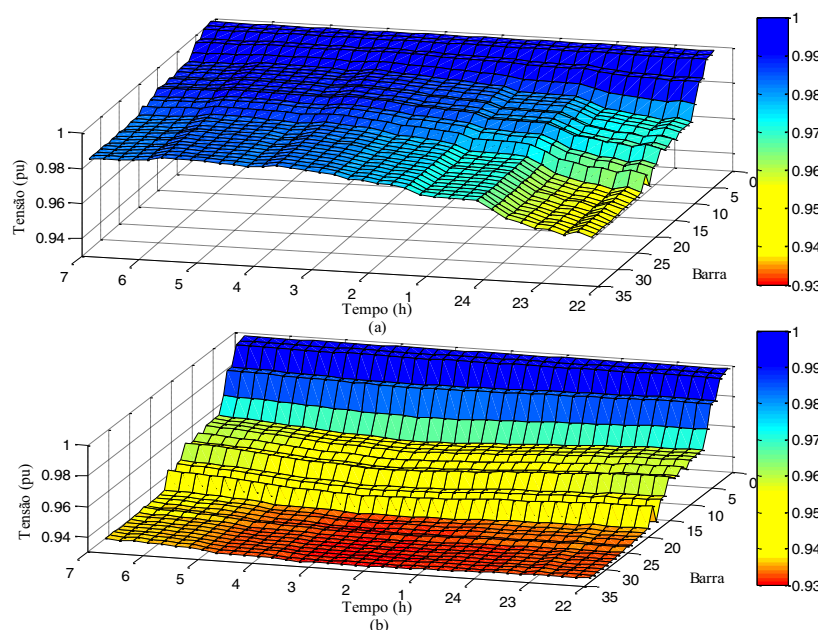
Figura 83 — Evolução da Tensão do sistema (a) sem PHEVs (b) com PHEVs
