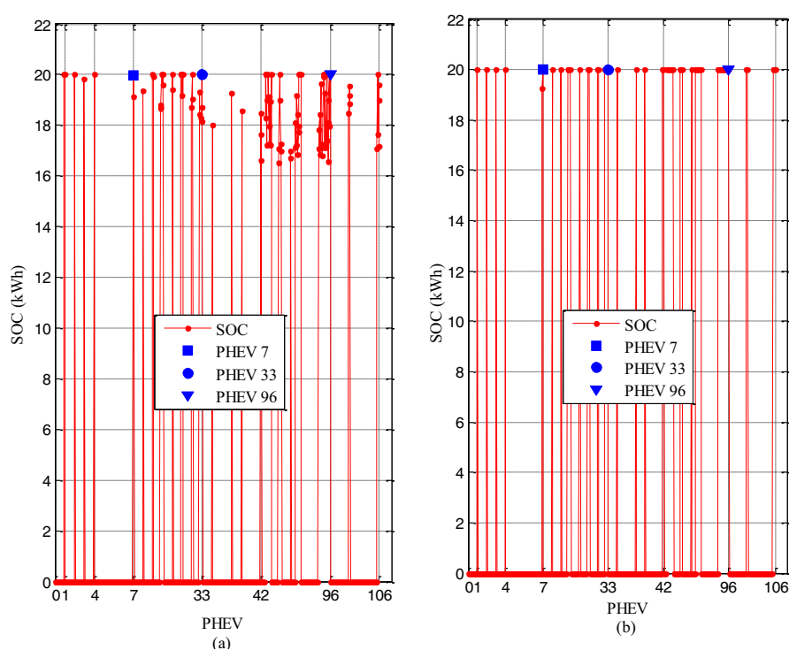
Figura 59 — SOC no final do período de recarga (a) sem aumento de 5% (b) com aumento de 5%
