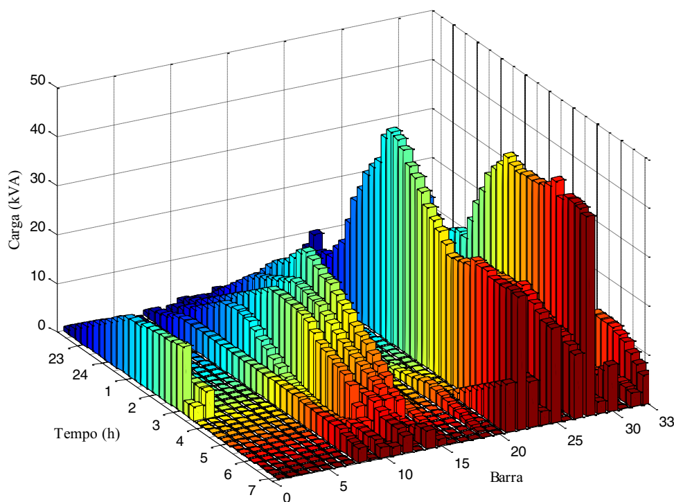
Figura 80 — Evolução de carga em transformadores de distribuição
