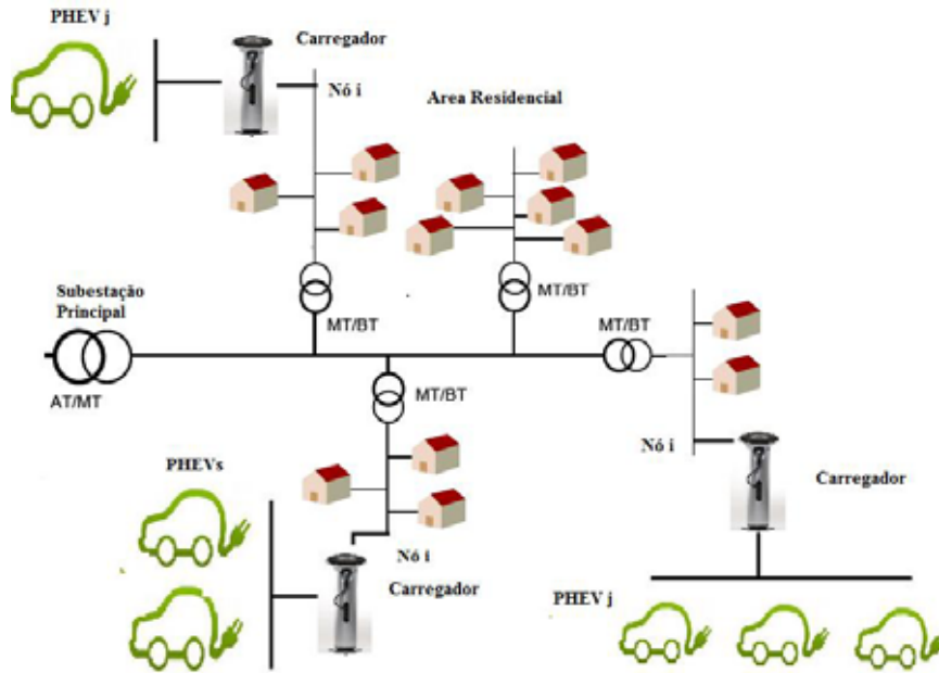
Figura 26 — Representação do sistema de média tensão com alocação de PHEVs na rede de baixa tensão
