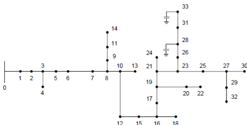
Figura 27 — Alimentador teste IEEE 34
