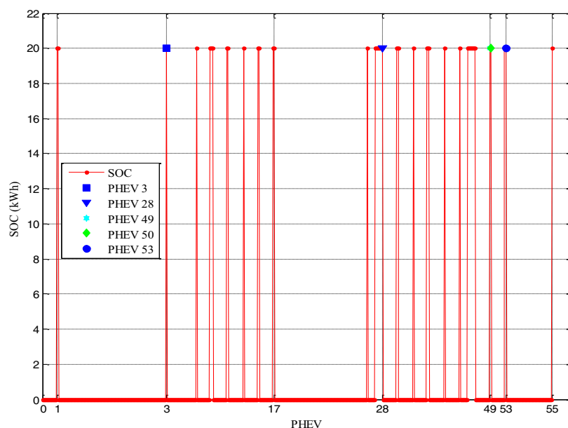
Figura 45 — SOC no final do período de recarga para um horário estendido
