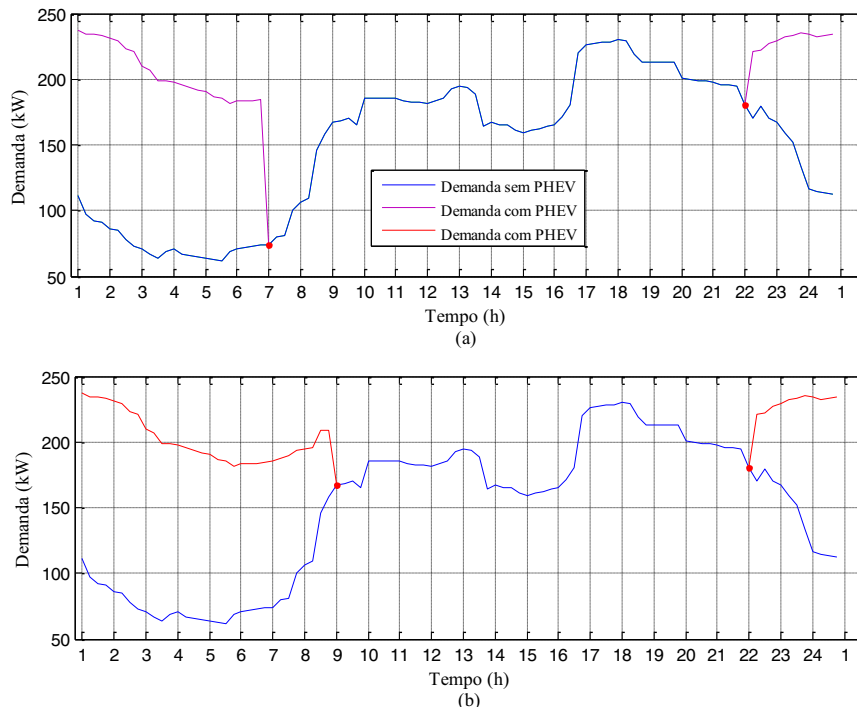
Figura 89 — Comparação demanda adicional de PHEVs (a) no horário noturno (b) no horário estendido
