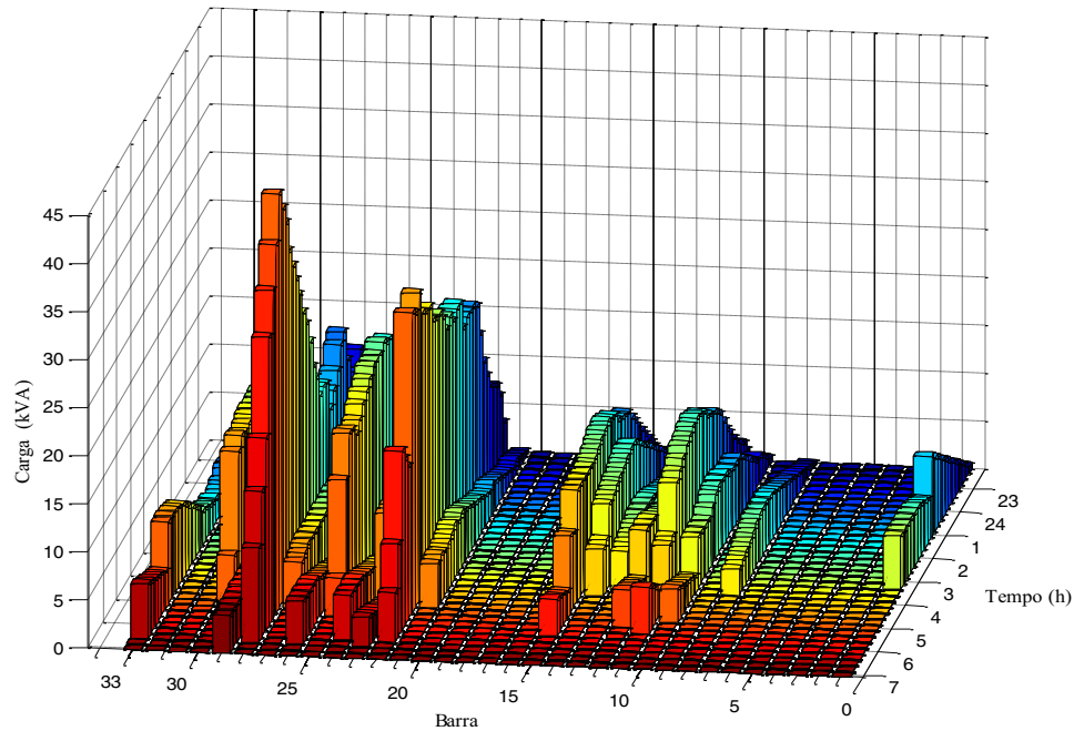
Figura 41 — Evolução da carga em transformadores
