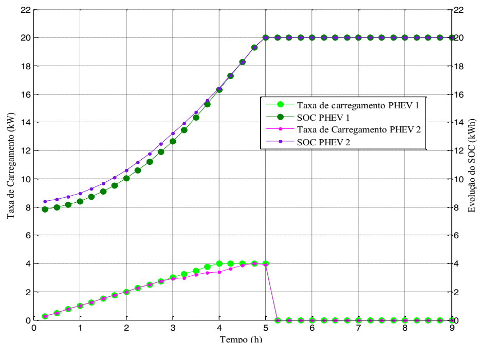
Figura 74 — Taxa de carregamento e evolução do SOC dos PHEVs 1 e 2
