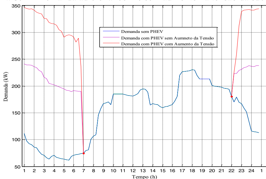
Figura 87 — Demanda adicional com e sem aumento na tensão da subestação
