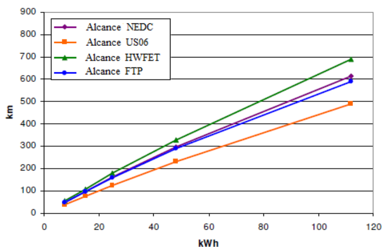
Figura 10 — Deslocamento vs capacidade da bateria de tecnologia atual
