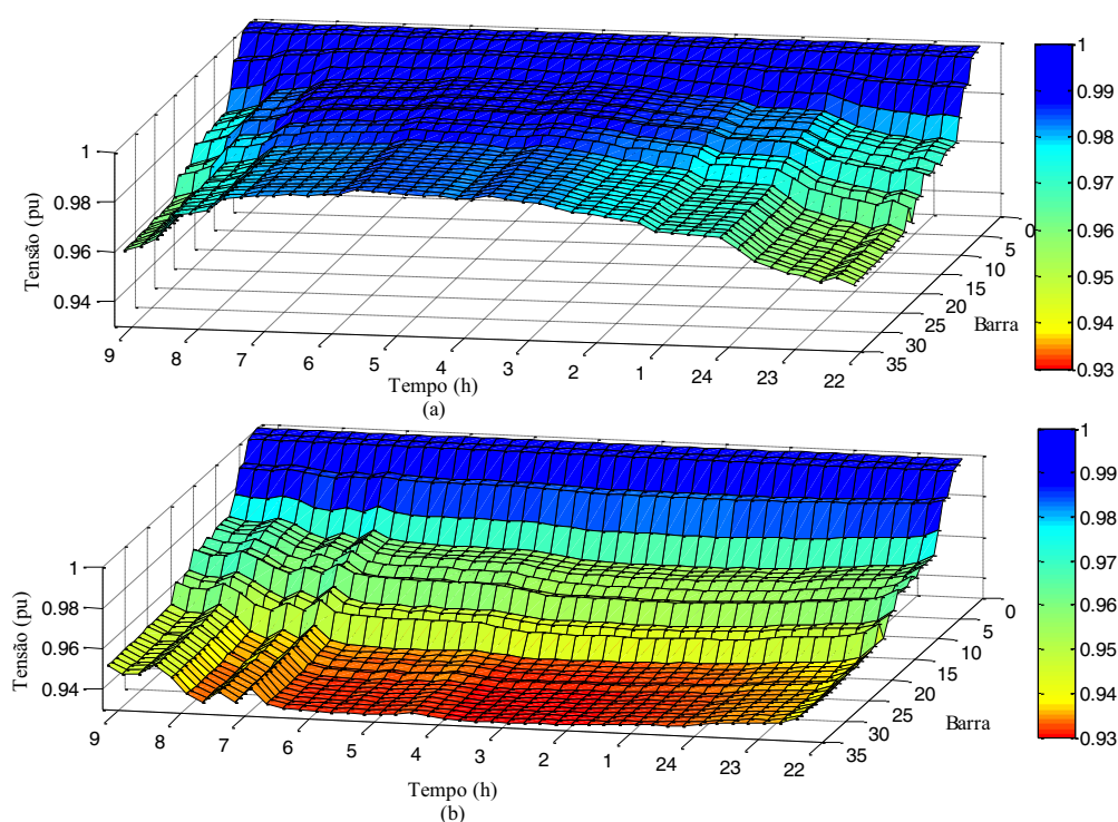
Figura 63 — Comparação da tensão (a) sem PHEVs (b) com PHEVs e horários estendido de recarga
