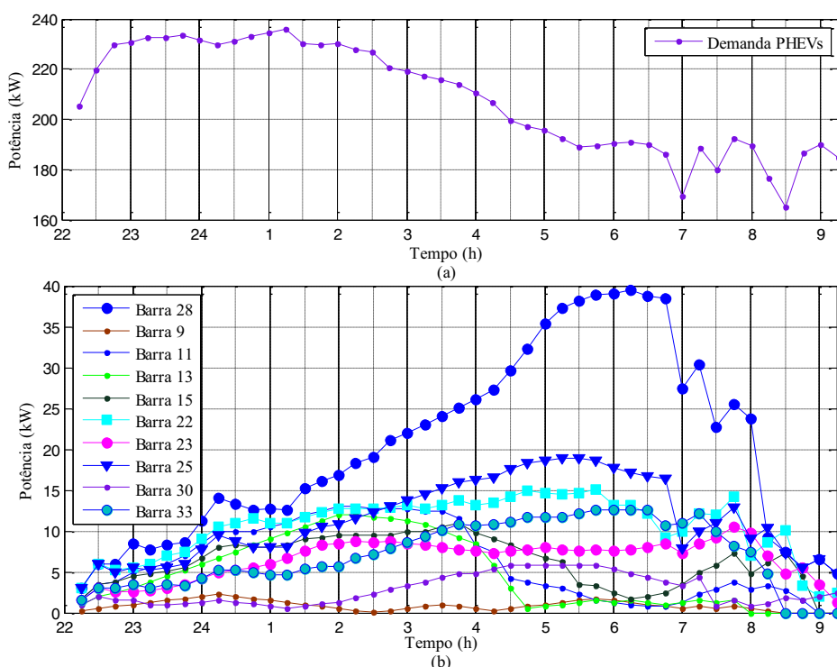
Figura 65 — (a) demanda no período estendido, (b) potências por barra após à otimização
