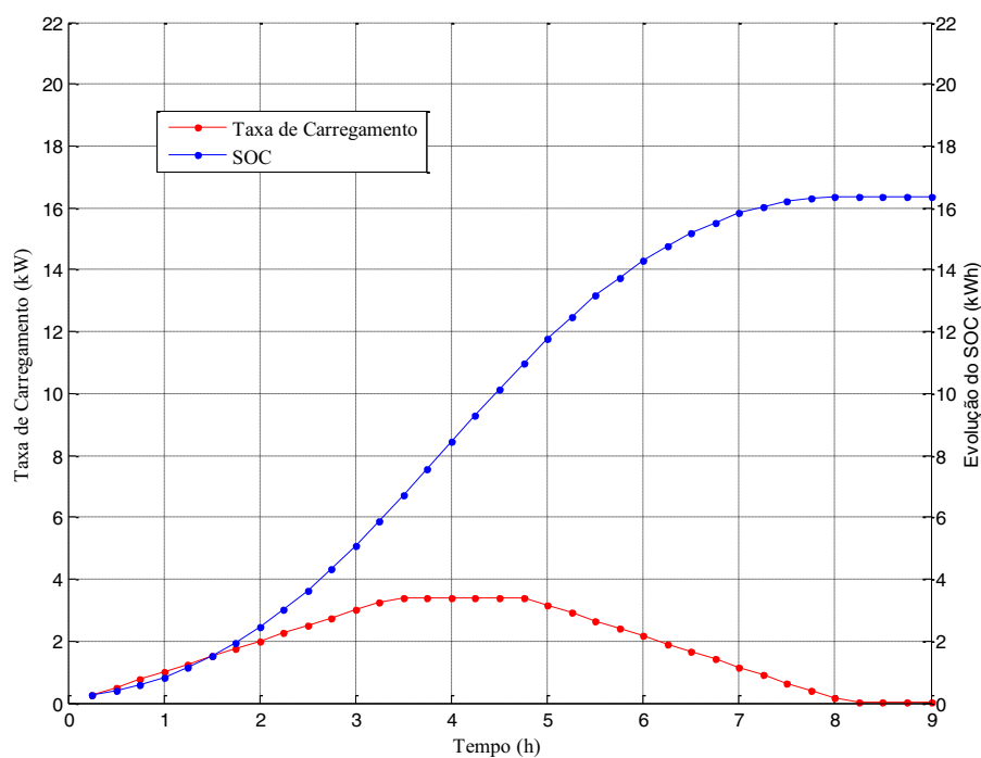
Figura 75 — Evolução do SOC e taxa de carregamento do PHEV 53
