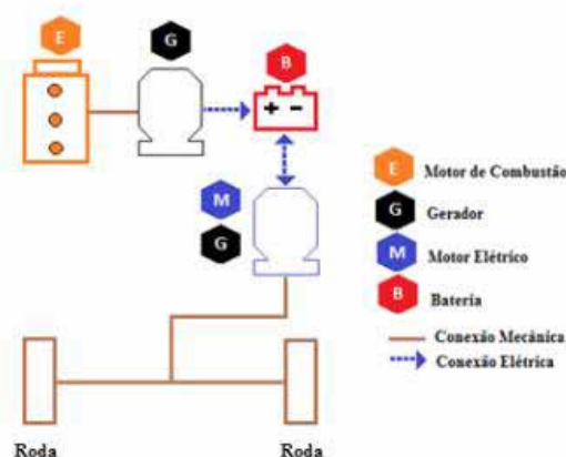
Figura 2 — Arquitetura híbrida série
