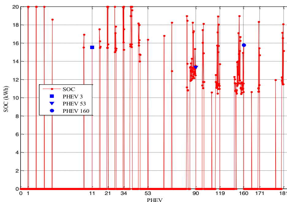
Figura 78 — Nível de SOC em todos os PHEVs no final do período de recarga
