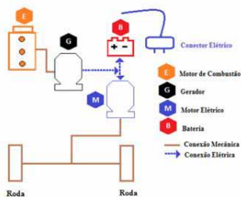
Figura 5 — Arquitetura PHEV série
