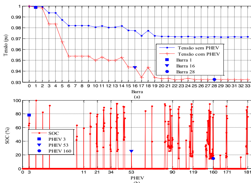
Figura 82 — Comparação (a) níveis de tensão do sistema (b) nível de SOC dos PHEVs
