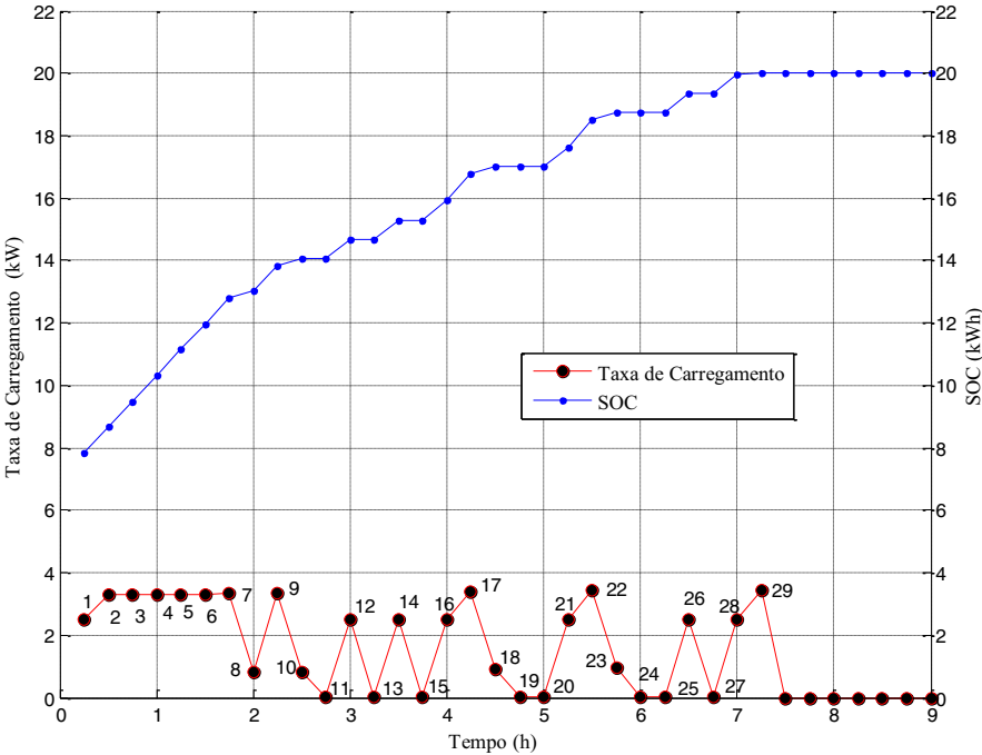
Figura 31 — Carregamento do PHEV 3 conectado na barra 8 sem considerar o \Delta_{phev}
