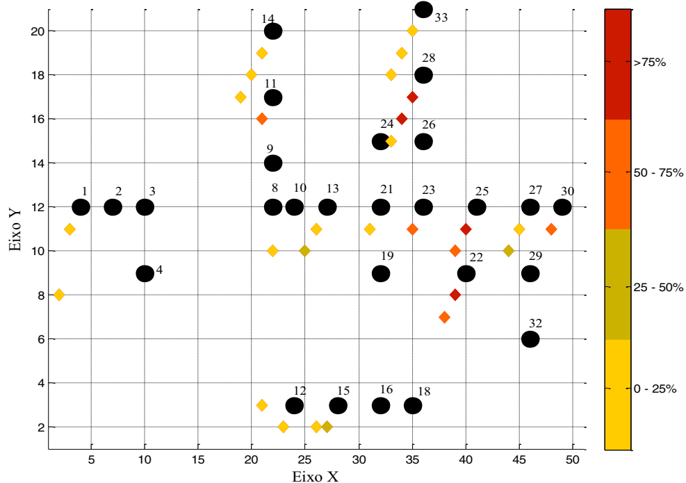
Figura 30 — Distribuição espacial dos PHEVs para 15% de penetração
