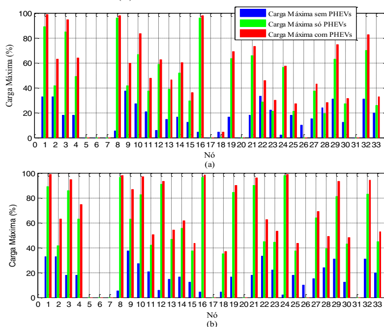
Figura 85 — Carga máxima em transformadores de distribuição (a) com aumento da tensão (b) sem aumento da tensão
