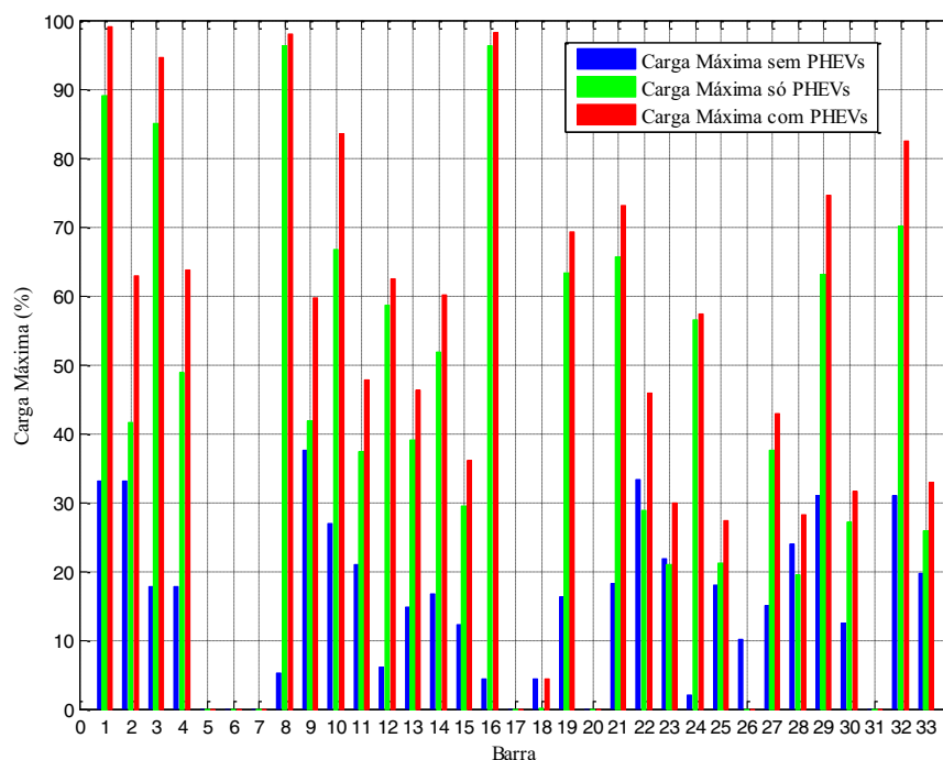
Figura 81 — Porcentagem de carga máxima em transformadores de distribuição
