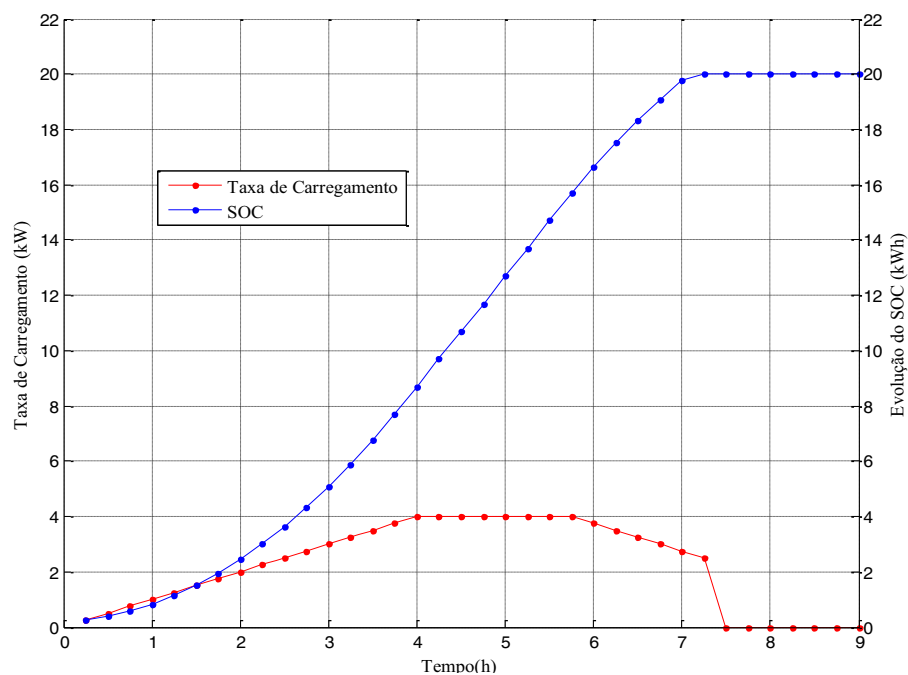
Figura 55 — Evolução do SOC e taxa de carregamento do PHEV 33
