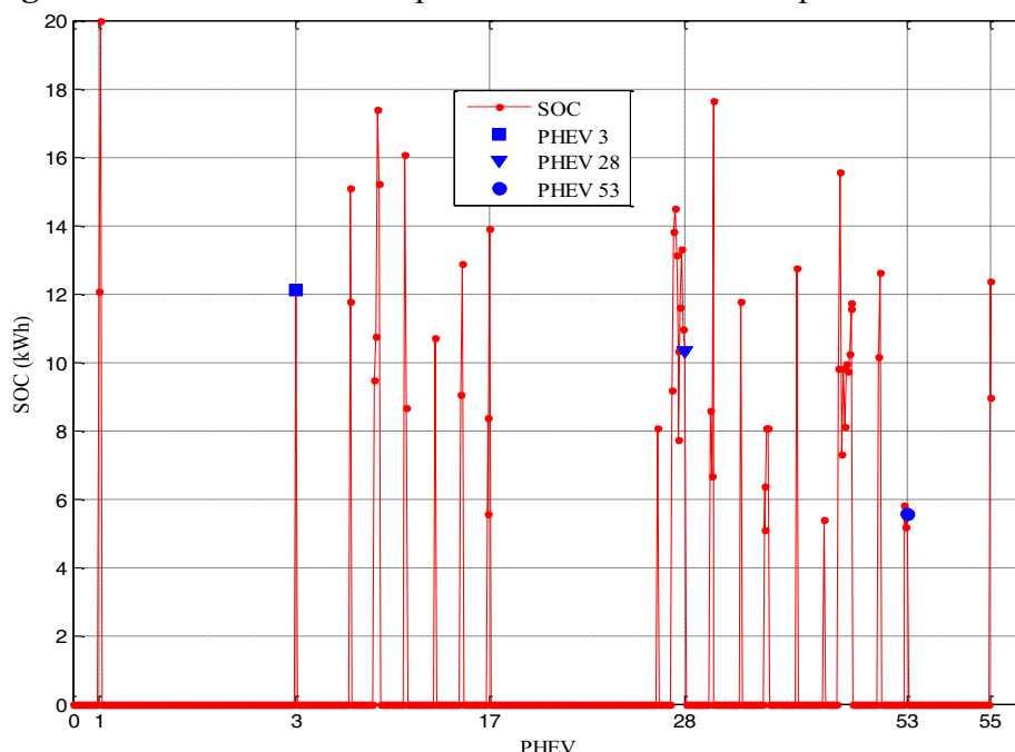
Figura 33 — Nível de SOC após três horas do início do período de recarga
