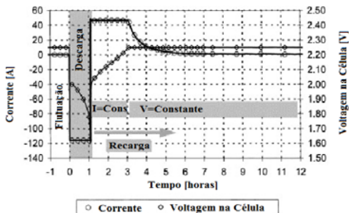
Figura 18 — Etapas de carga de uma bateria de chumbo-acido
