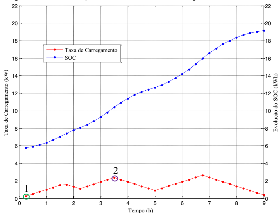
Figura 53 — Evolução do SOC e taxa de carregamento do PHEV 6
