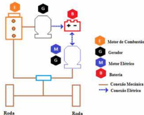
Figura 4 — Arquitetura híbrida série-paralelo
