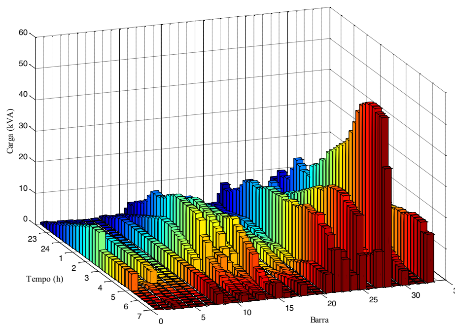
Figura 66 — Evolução da carga de transformadores em um cenário de recarga controlado
