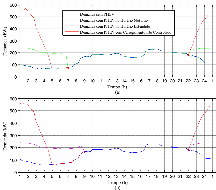
Figura 93 —Demanda adicional (a) cenário de recarga noturno controlado e não controlado (b) cenário de recarga estendido controlado e não controlado
