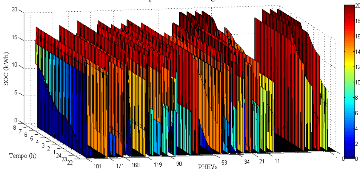
Figura 79 — Evolução do SOC em todos os PHEVs conectados para todo o período de recarga
