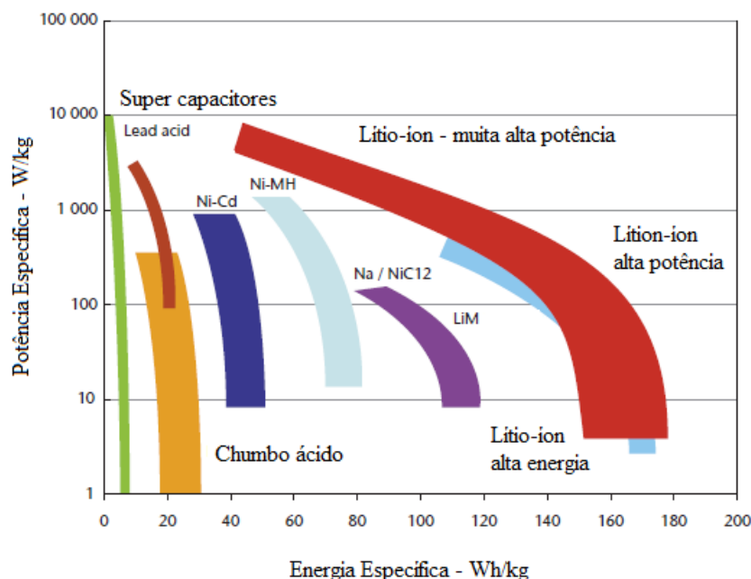
Figura 13 — Energia específica e potência específica para diferentes tipos de baterias
