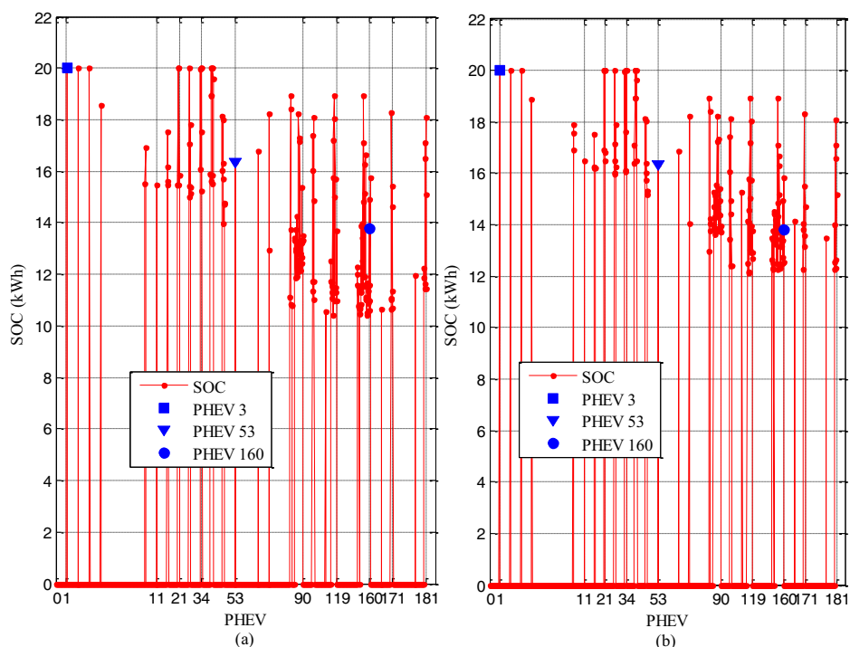
Figura 88 — Comparação do nível de SOC (a) período noturno (b) período estendido
