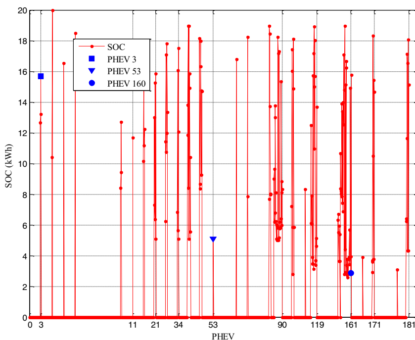
Figura 72 — Nível de SOC após três horas do início do período de recarga
