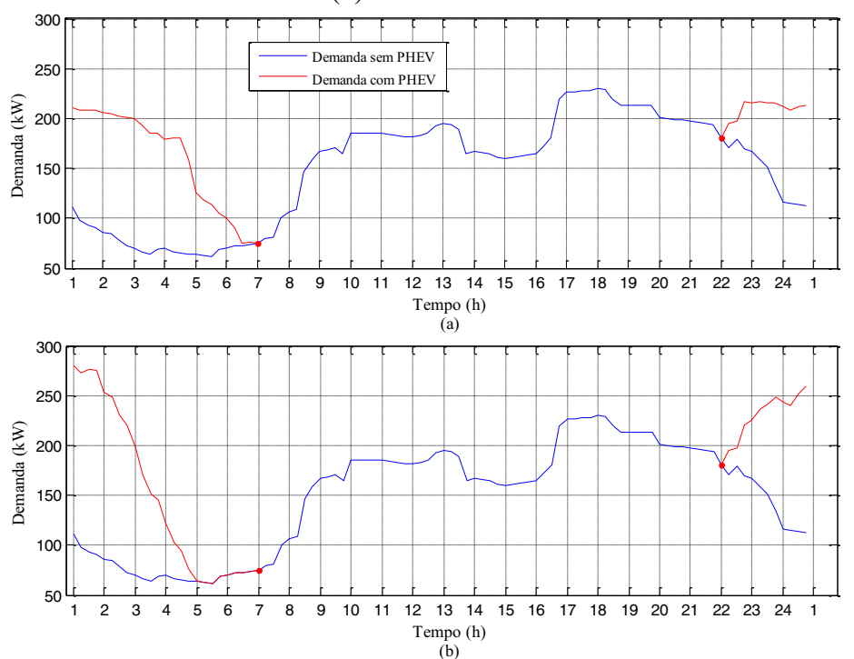
Figura 50 — Demanda adicional em um cenário de recarga (a) controlado e (b) não controlado
