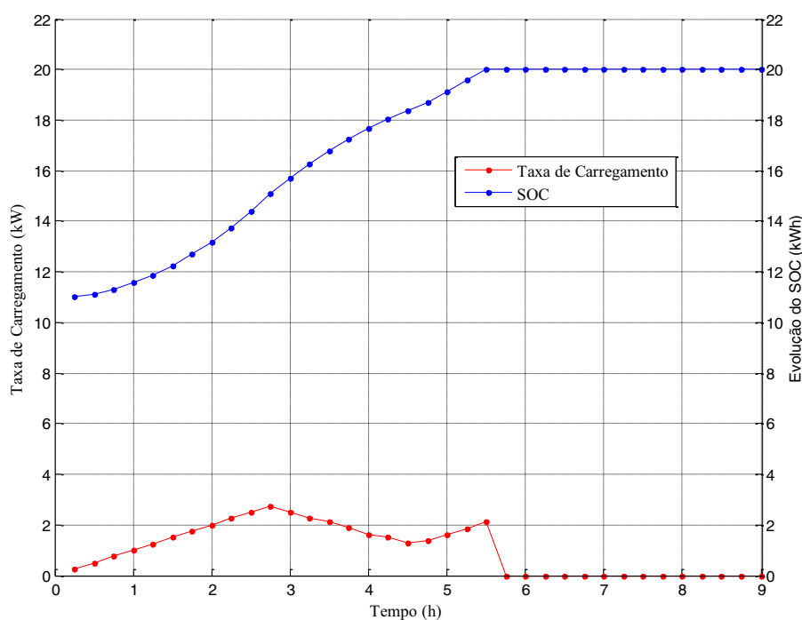
Figura 73 — Evolução do SOC e taxa de carregamento do PHEV 3
