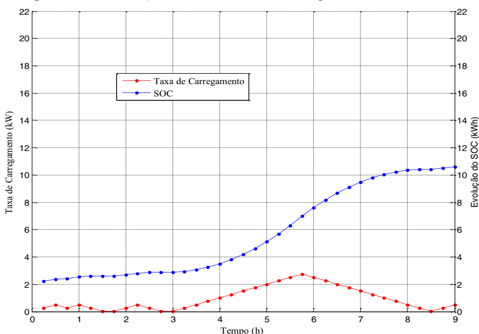
Figura 76 — Evolução do SOC e taxa de carregamento do PHEV 160
