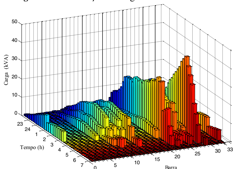
Figura 40 — Evolução da carga em transformadores.
