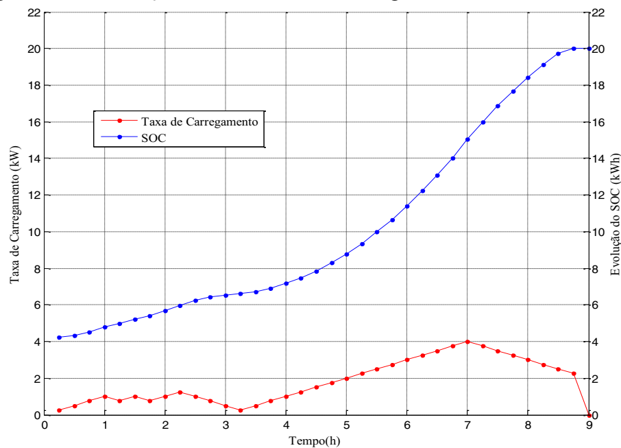
Figura 56 — Evolução do SOC e taxa de carregamento do PHEV 96
