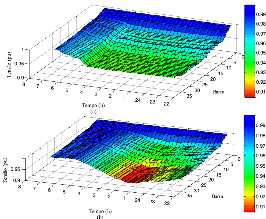
Figura 49 — Níveis de tensão para um cenário de recarga (a) controlado e (b) não controlado
