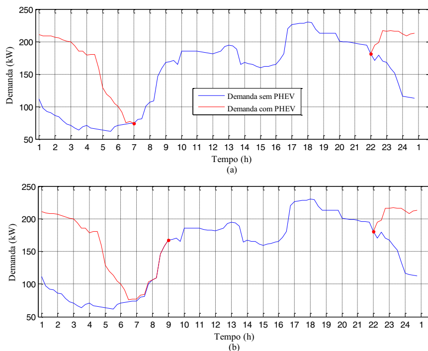
Figura 46 — Demanda adicional para dois períodos de recarga (a) noturno de 9h e (b) estendido de 11h
