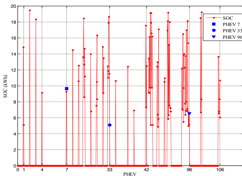
Figura 52 — Nível do SOC após três horas do início do período de recarga
