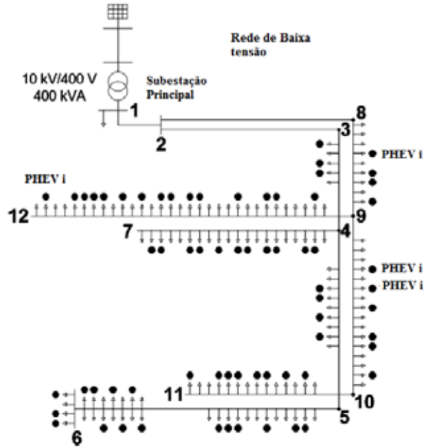
Figura 25 — Sistema de baixa tensão com conexão de PHEV considerado no modelo inicial
