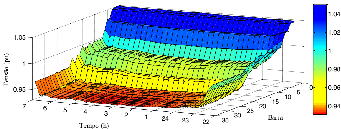
Figura 86 — Níveis de tensão considerando um aumento de tensão de 5% na tensão da subestação
