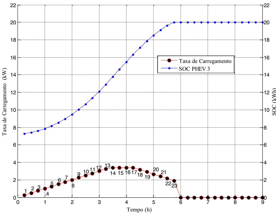
Figura 32 — Taxa de carregamento e evolução do SOC do PHEV 3 considerando o \Delta_{phev}
