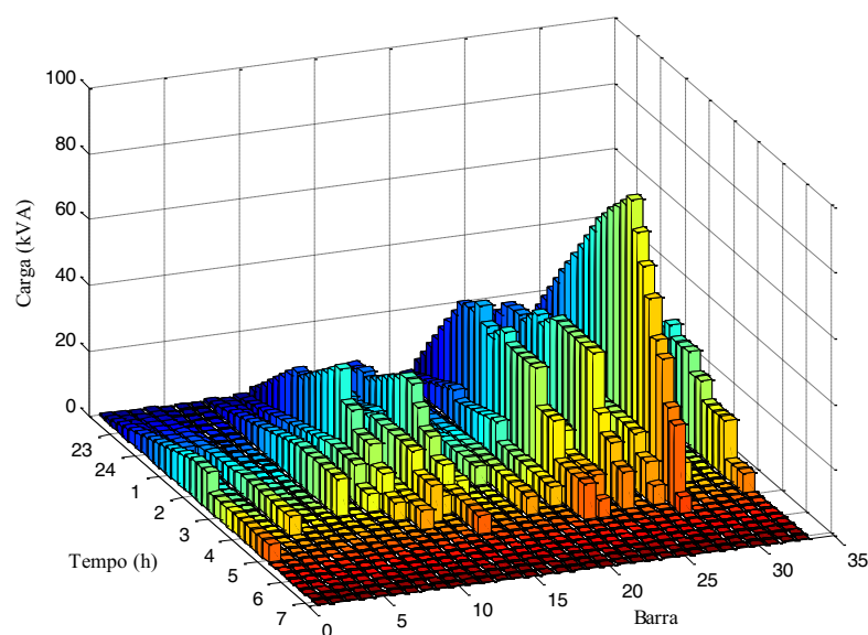
Figura 67 — Evolução de carga de transformadores em um cenário de recarga não controlado
