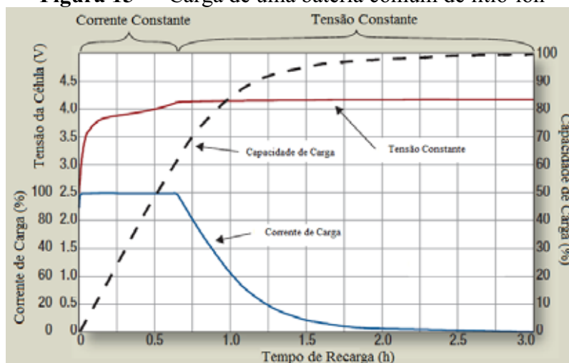
Figura 15 — Carga de uma bateria comum de lítio-íon
