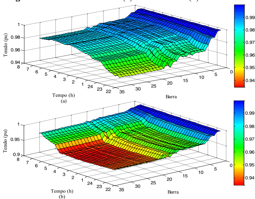
Figura 43 — Níveis de tensão (a) sem PHEVs e (b) com PHEVs
