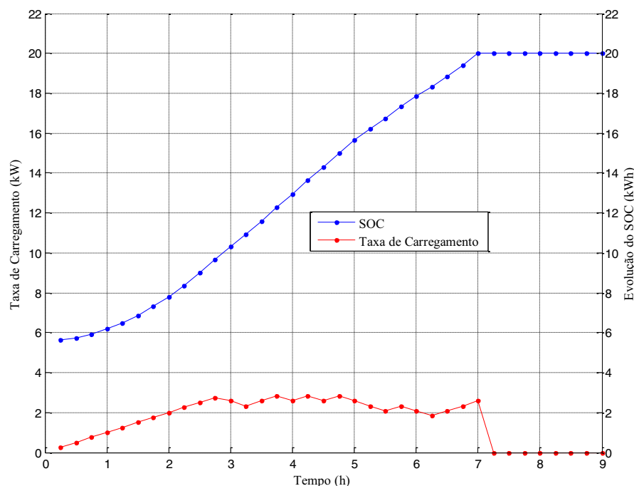
Figura 35 — Evolução do SOC e taxa de carregamento do PHEV 28
