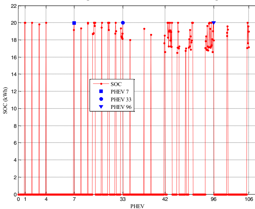
Figura 57 — Nível do SOC para todos os PHEVs no final do período de recarga
