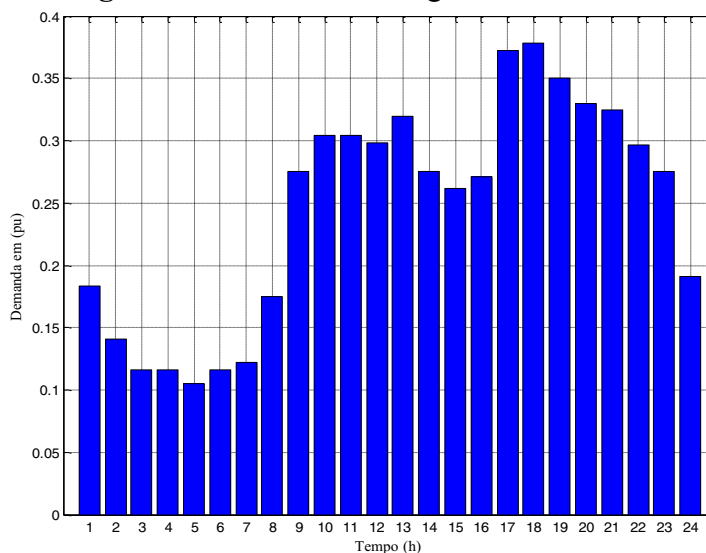
Figura 28 — Curvas de carga diárias sazonais
