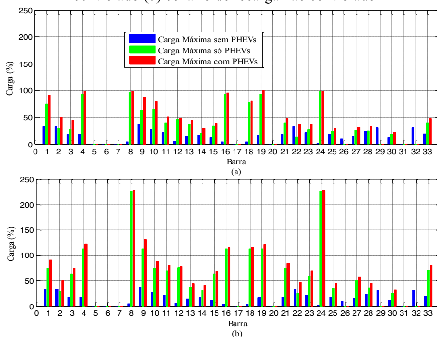
Figura 68 — Porcentagem de carga máxima em transformadores (a) cenário de recarga controlado (b) cenário de recarga não controlado
