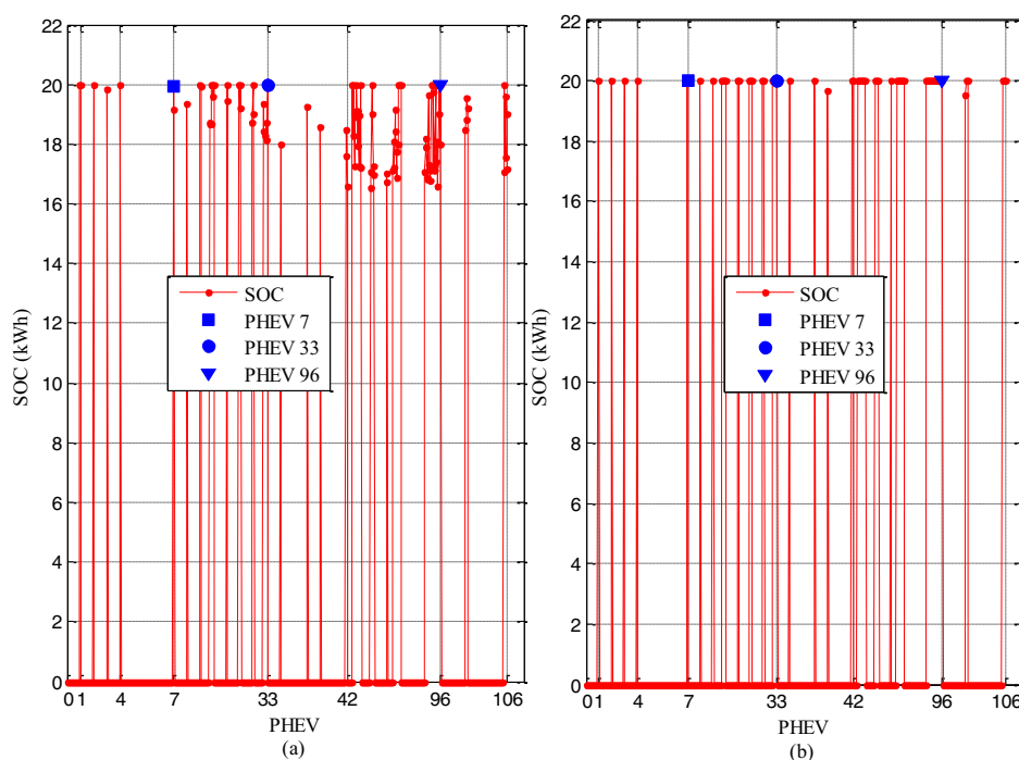
Figura 62 — Comparação do nível de SOC (a) horário normal (b) horário estendido
