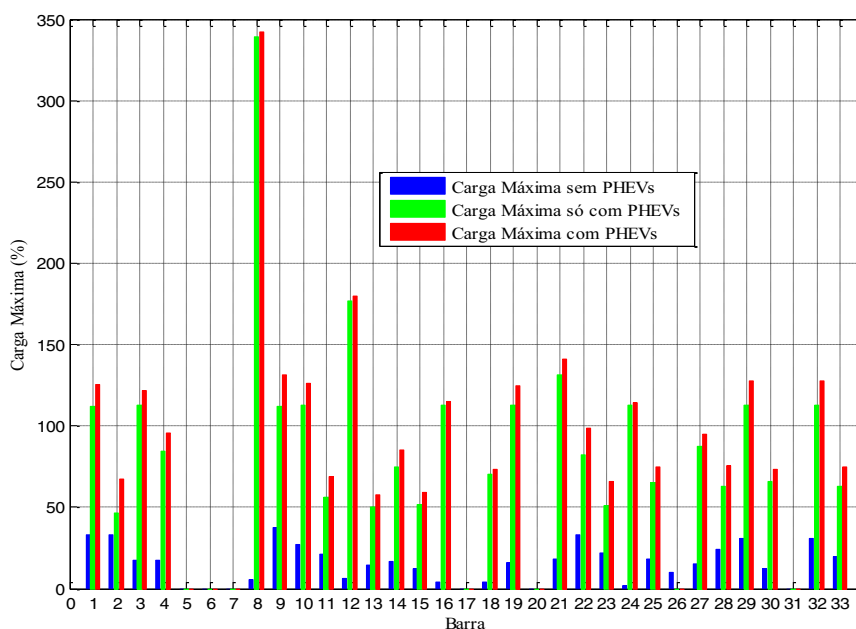
Figura 91 — Carga máxima em transformadores de distribuição
