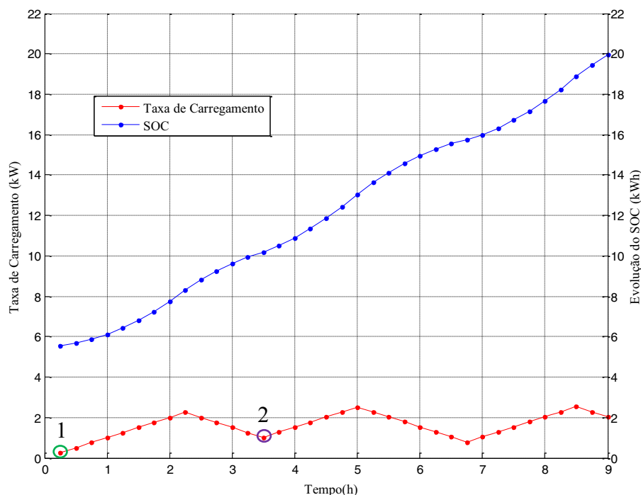
Figura 54 — Evolução do SOC e taxa de carregamento do PHEV 7
