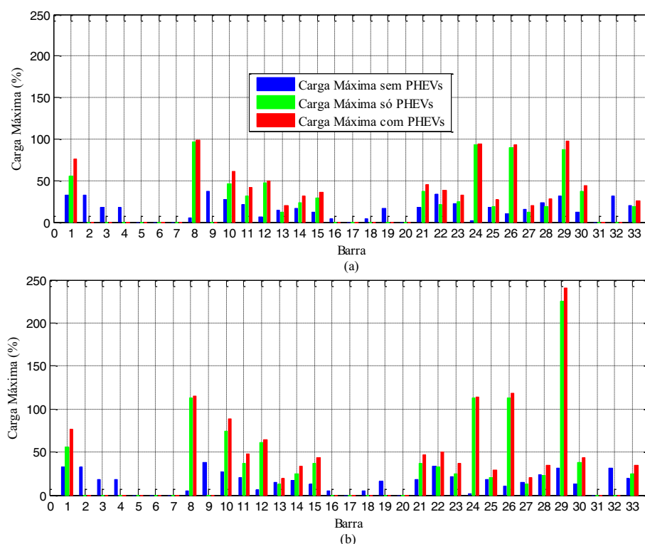
Figura 48 — Comparação de carga máxima (a) controlada e (b) não controlada
