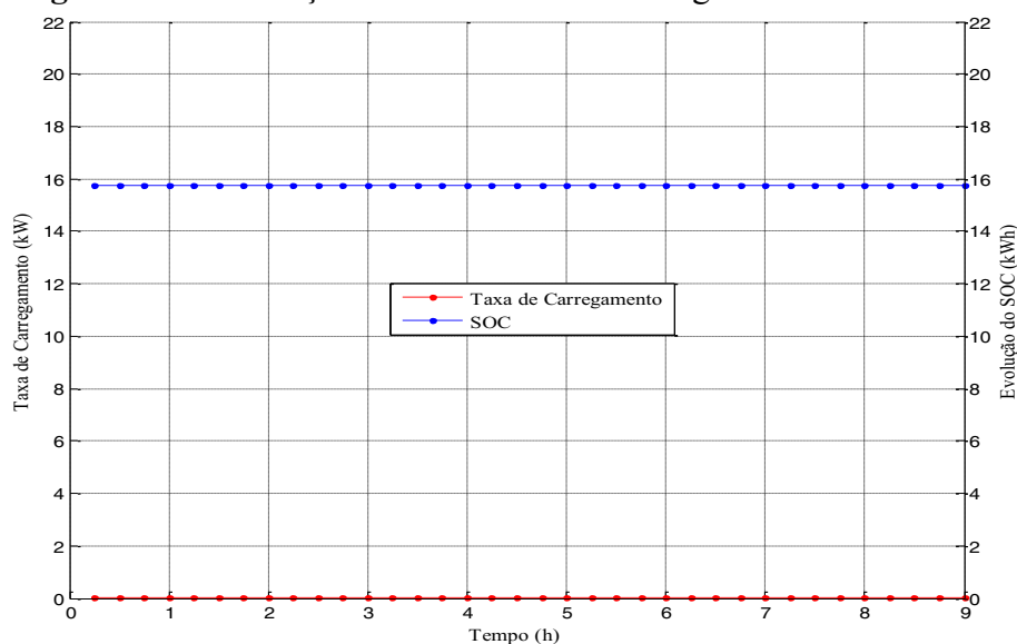
Figura 77 — Evolução do SOC e taxa de carregamento do PHEV 162
