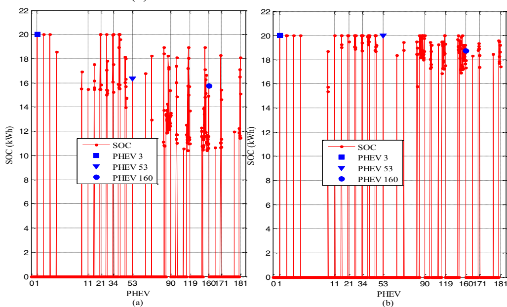
Figura 84 — Comparação do nível de SOC (a) sem aumento na tensão de referência (b) com aumento na tensão de referência
