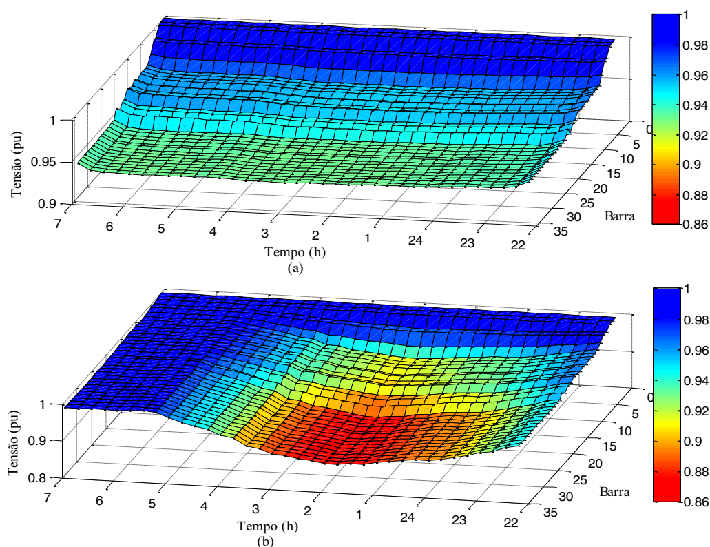
Figura 69 — Evolução da tensão no cenário de (a) recarga controlada (b) não controlada
