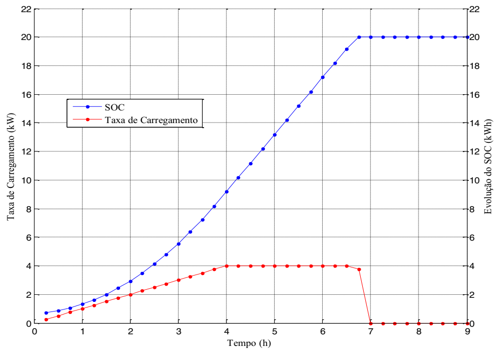
Figura 37 — Evolução do SOC e taxa de carregamento do PHEV 53
