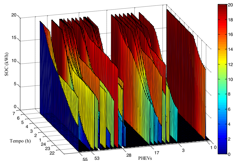
Figura 39 — Evolução do SOC para todo o período de recarga de todos os PHEVs
