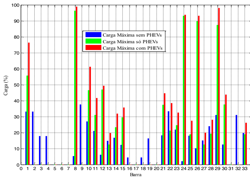
Figura 42 — Porcentagem de carga máxima em transformadores
