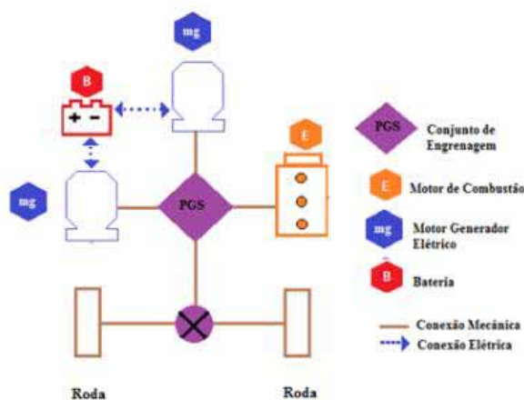
Figura 7 — Arquitetura PHEV com potência dividida
