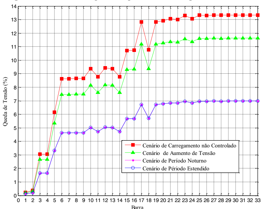
Figura 70 — Porcentagens de queda de tensão para cada cenário
