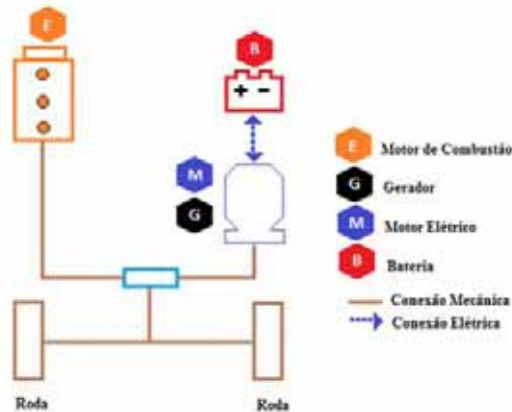
Figura 3 — Arquitetura híbrido paralelo
