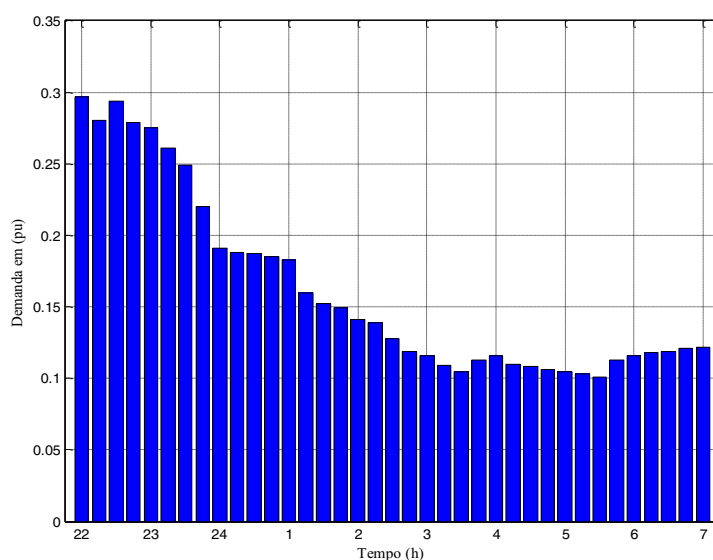
Figura 29 — Curva de carga no horário de carregamento dos PHEVs
