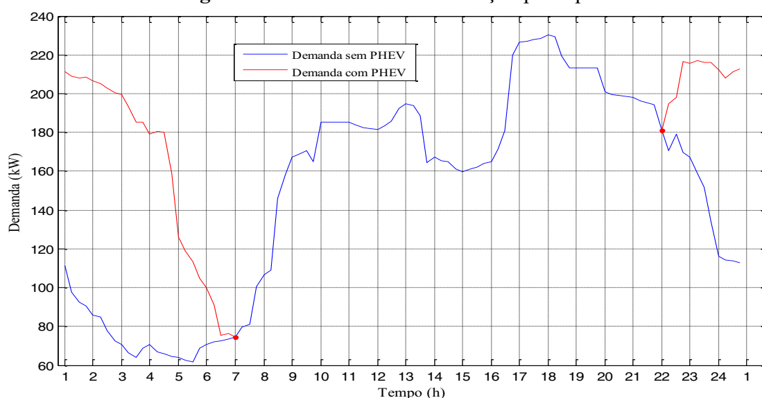
Figura 44 — Demanda na subestação principal
