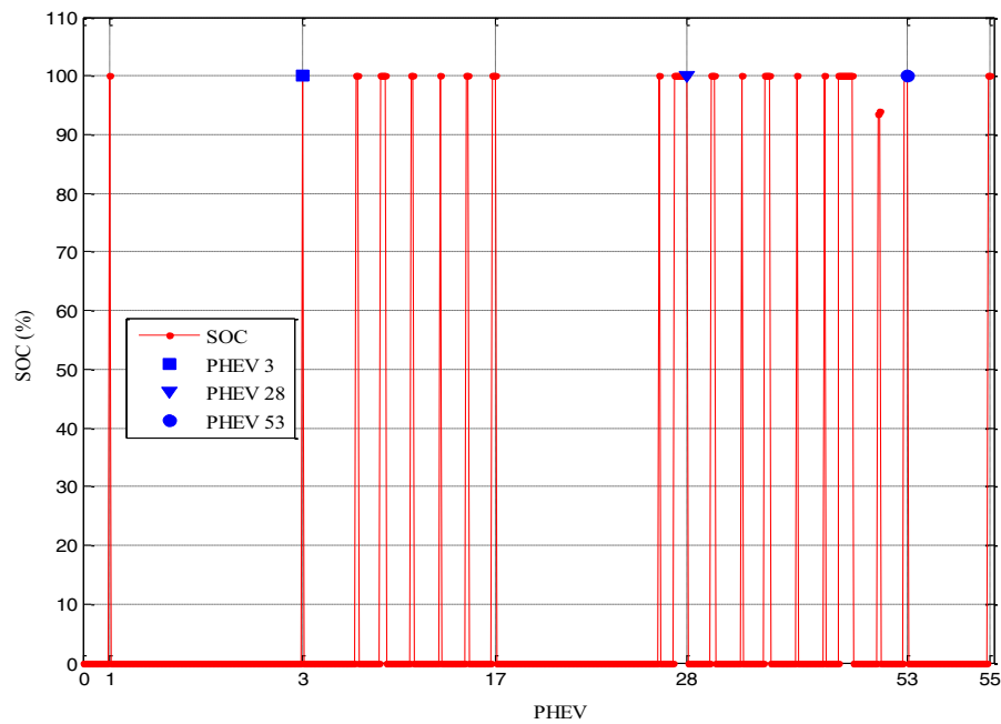
Figura 38 — Nível de SOC no final do período de recarga
