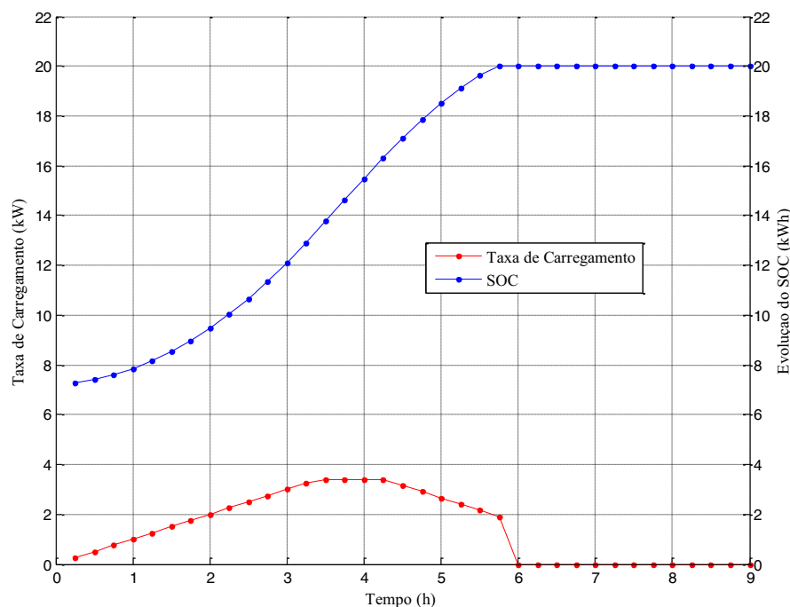
Figura 34 — Evolução do SOC e taxa de carregamento do PHEV 3
