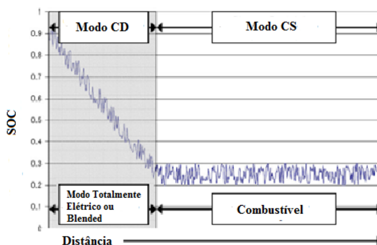
Figura 8 — Operação do PHEV
