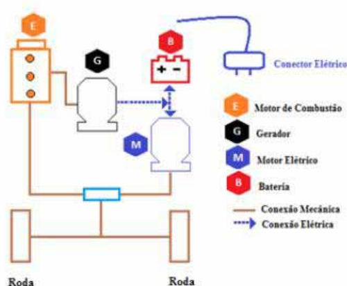
Figura 6 — Arquitetura PHEV paralelo
