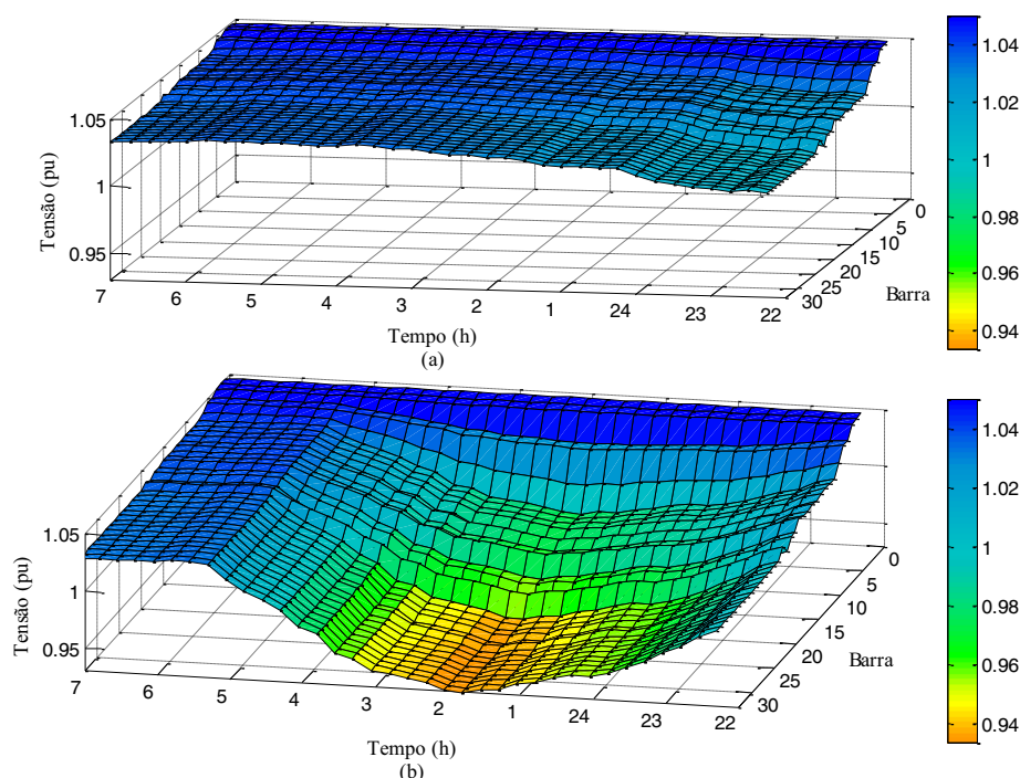
Figura 60 — Níveis e tensão com um aumento de 5% na tensão da subestação principal (a) sem presença de PHEVs (b) com presença de PHEVs
