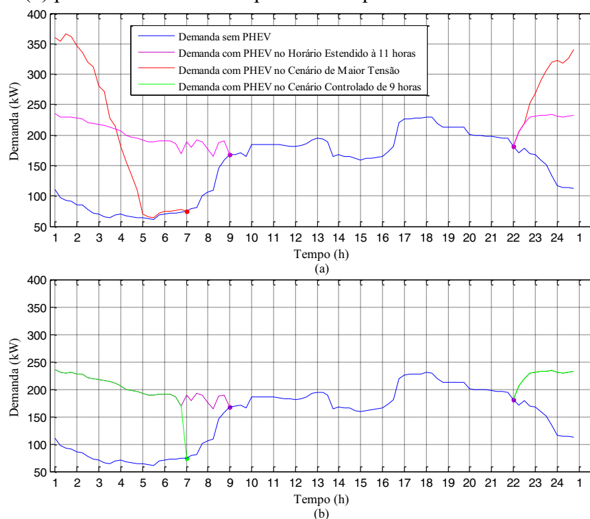
Figura 64 — Demanda adicional (a) período estendido comparado com o aumento da tensão (b) período estendido comparado com período controlado de 9 h
