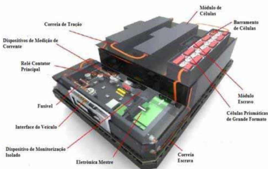
Figura 12 — Exemplo de uma bateria
