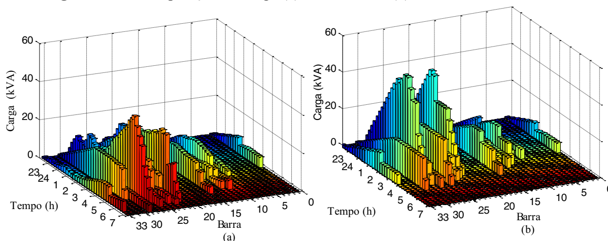
Figura 47 — Comparação de carga (a) Controlada e (b) Não controlada
