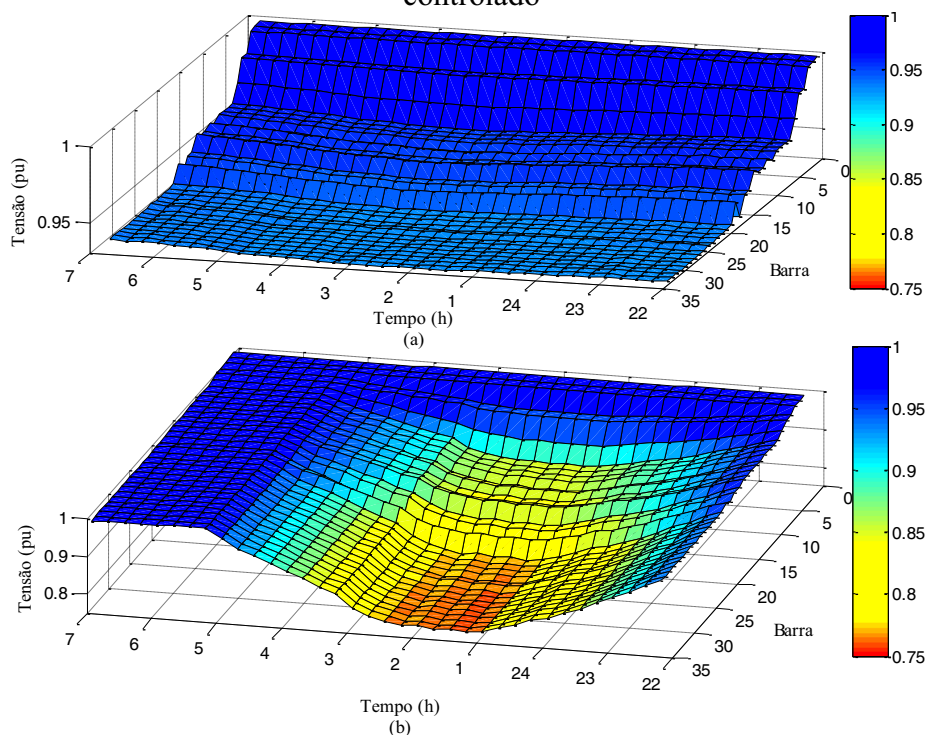
Figura 92 — Níveis de tensão em um cenário de recarga (a) controlado (b) não controlado
