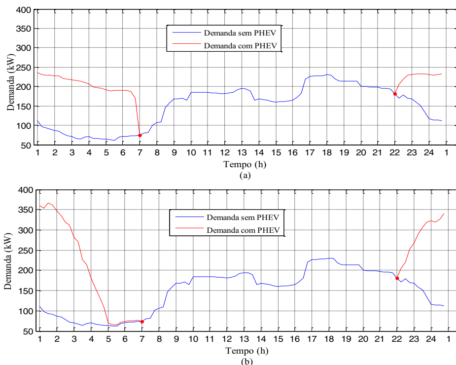
Figura 61 — (a) demanda adicional na presença de PHEVs (b) demanda adicional na presença de PHEVs e aumento da tensão na subestação
