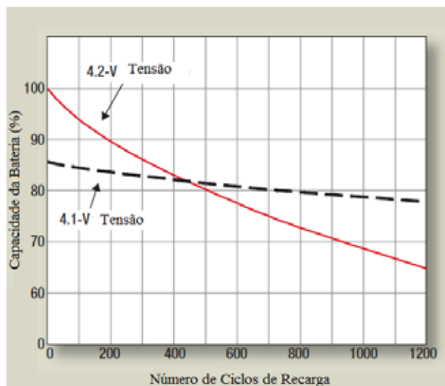
Figura 14 — Diminuição da capacidade da bateria de lítio-íon
