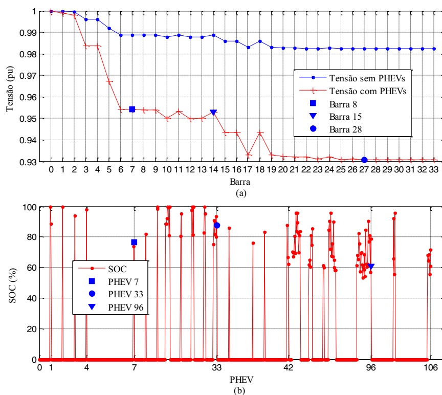
Figura 58 — (a) Níveis de Tensão (b) nível de SOC
