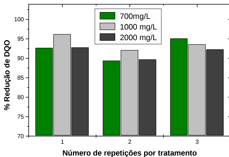
Figura 01. Eficiências de redução de DQO para o reator sem agitação.
