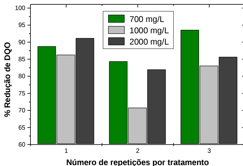
Figura 02. Eficiências de redução de DQO para o reator com agitação.
