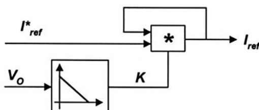
Figura 2.21 – Diagrama de blocos simplificado do controle proposto.
