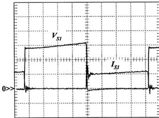
Escala vertical: V_{S1} : 100 V/div; I_{S1} : 5 A/div Escala horizontal: 3,5 ms/div; (a) V_{S1} e I_{S1}
