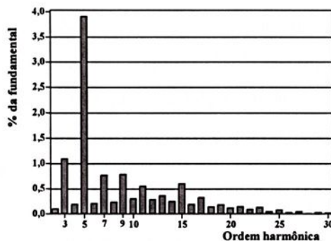
Figura 4.24 – Espectro harmônico da tensão de saída.
