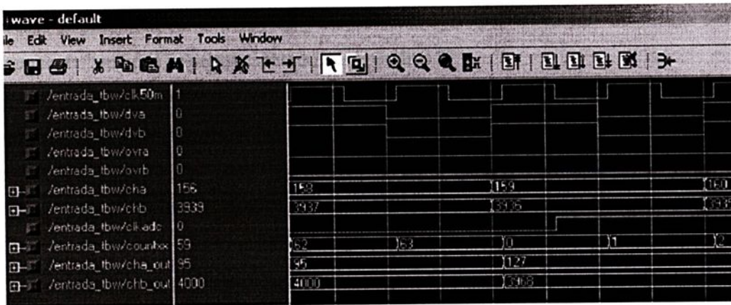
Figura 3.5 – Resultado de simulação da descrição VHDL do componente “entrada” através do simulador ModelSim 5.7g XE II.
