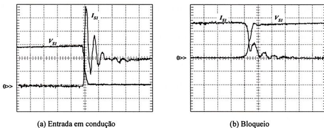
Figura 4.19 – Detalhe das comutações do interruptor Mosfet S_1 .
