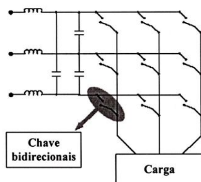
Figura 1.5 – Diagrama do conversor em matriz (CM).
