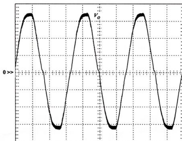
Figura 4.23 – Tensão de saída considerando 95 % da carga nominal.
