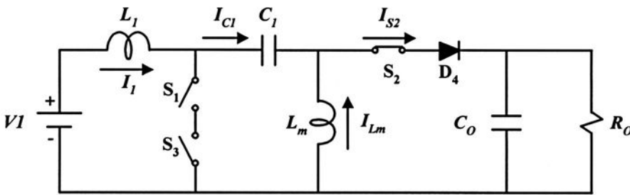
Figura 2.5 - Topologia para a 2ª etapa de funcionamento.
