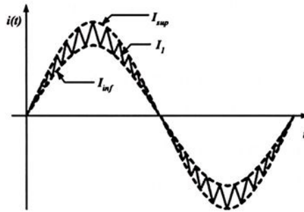
Figura 2.15 – Detalhe da modulação (controle) por histerese variável.
