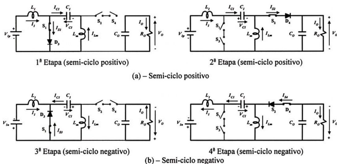
Figura 2.6 – Etapas de funcionamento para o conversor proposto durante a evolução dos dois semi-ciclos da tensão de alimentação CA.
