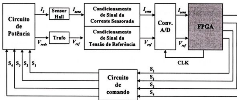
Figura 3.1 - Diagrama de blocos simplificado incluindo: Circuito de potência, Sensor “Hall”, Trafo (sensor de tensão), Condicionamento de sinais para o conversor A/D, FPGA e Circuito de comando.
