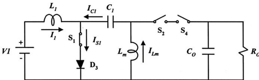
Figura 2.4 - Topologia para a 1ª etapa de funcionamento.
