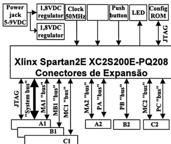
Figura 4.4 – Diagrama de blocos do D2SB.
