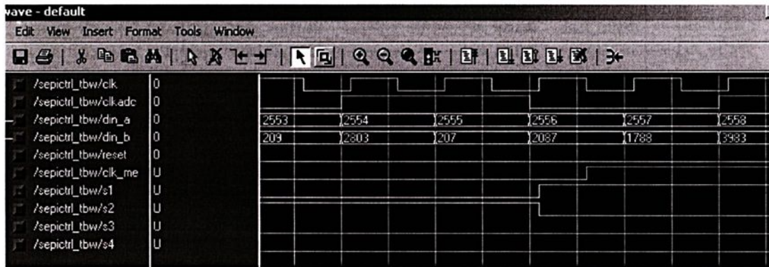
Figura 3.7 – Resultado de simulação do funcionamento do componente “sepictl” através do simulador ModelSim 5.7g XE II.
