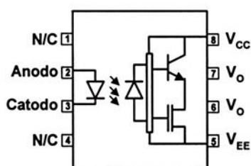
Figura 4.8 – Diagrama do HCPL-3180 da Agilent.
