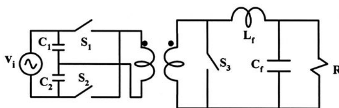
Figura 1.4 - Conversor Half-Bridge para operação CA/CA, proposto em [10].
