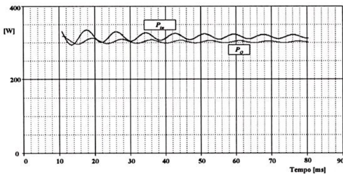
Figura 2.33 - Potência de entrada e potência de saída para o conversor proposto.
