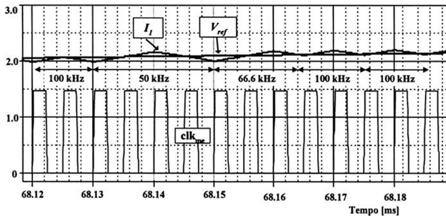
Figura 2.19 - Verificação da variação da frequência de chaveamento em função do evento de "clock" ( clk_{me} ) no semi-ciclo positivo.
