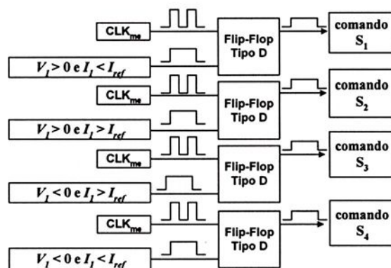
Figura 2.18 – Diagrama lógico simplificado do controle proposto.
