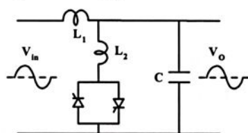
Figura 1.2 - Regulador de tensão CA à SCRs, usando técnica de impedância variável.
