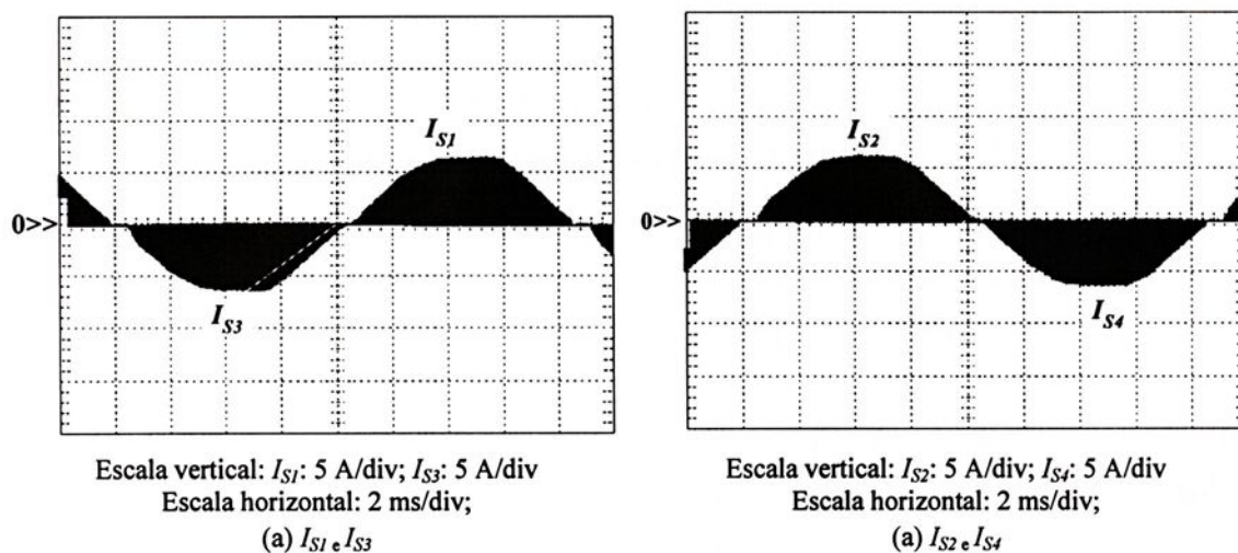
Figura 4.26 – Correntes através dos interruptores S_1 , S_2 , S_3 e S_4 .
