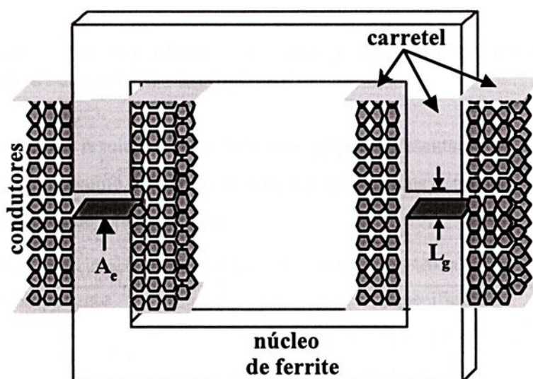
Figura 4.10 - Núcleo tipo UU com seus principais parâmetros.
