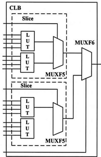
Figura N.3 – Multiplexadores F5 e F6 nos CLBs.
