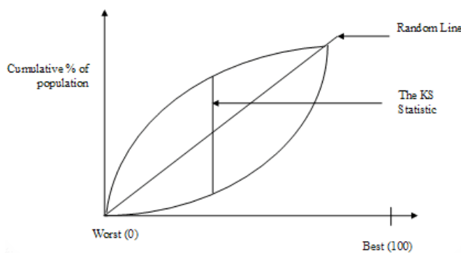
Figura 15 – Kolgomorov-Smirnov (KS)
