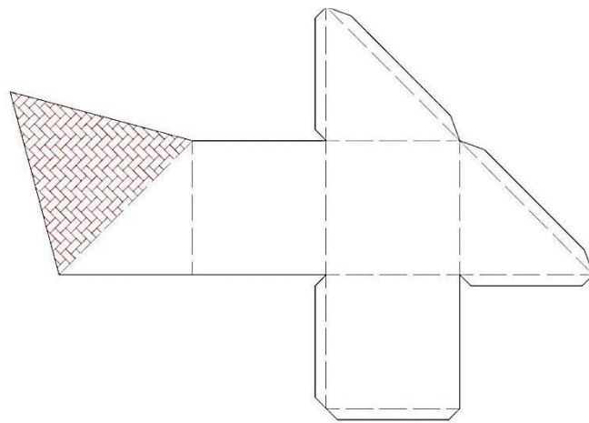
Figura 77 – Planificação da peça maior seccionada do hexaedro regular.
