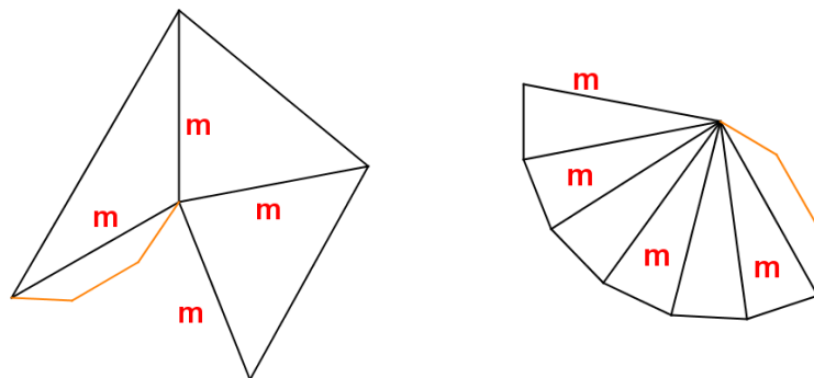
Figura 52 – Planificação das peças representativas dos vértices da base (seis peças, à esquerda) e do ápice (uma peça, à direita) da pirâmide hexagonal reta.
