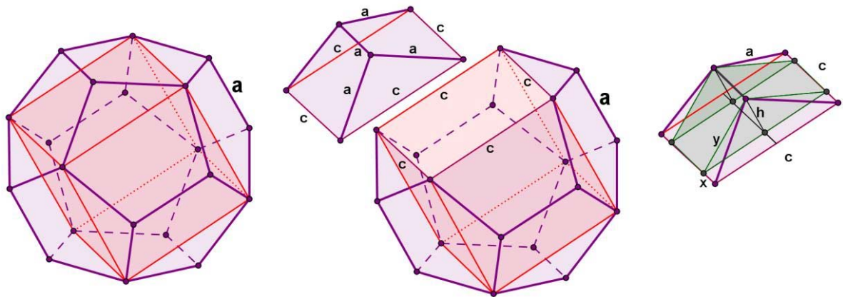
Figura 10 – Decomposição do dodecaedro regular para o cálculo de seu volume.
