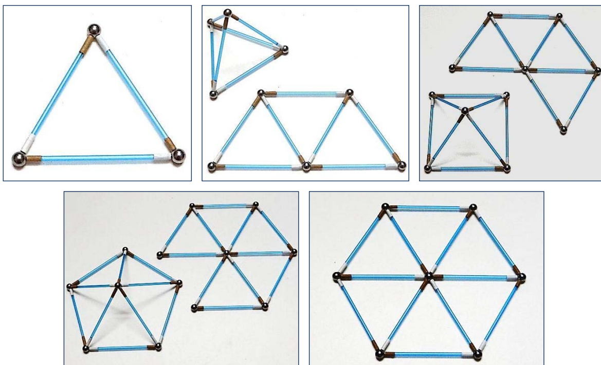
Figura 113 – Fotografias mostrando estruturas com triângulos para representações dos ângulos poliédricos dos sólidos regulares.
