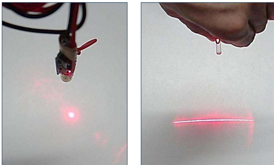
Figura 120 – Fotografias mostrando a conversão de um feixe cilíndrico de laser em um plano de luz, através do acoplamento de um pequeno bastão de vidro.
