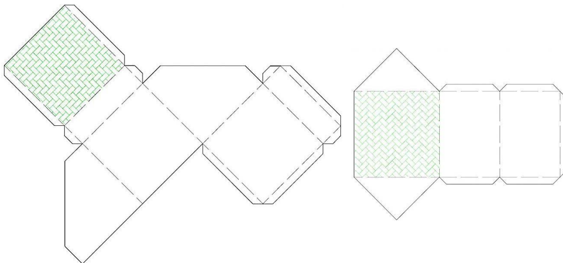
Figura 85 – Planificações das peças geradas do seccionamento do cubo mostradas na Figura 84. À esquerda, um prisma pentagonal irregular e à direita, um prisma triangular.
