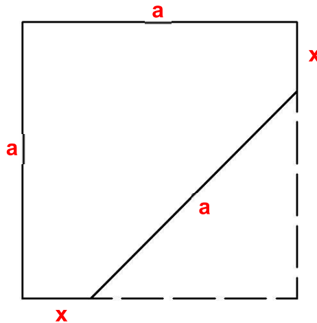
Figura 83 – Figura que auxilia na determinação dos pontos em que o plano paralelo a quatro arestas deve passar para se obter uma seção quadrada no cubo de aresta a .
