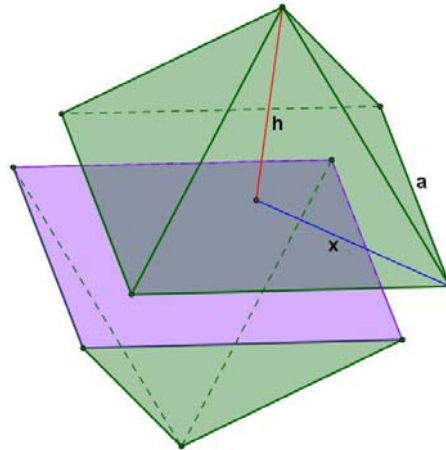
Figura 8 – Octaedro regular e seus principais elementos para a determinação de seu volume.
