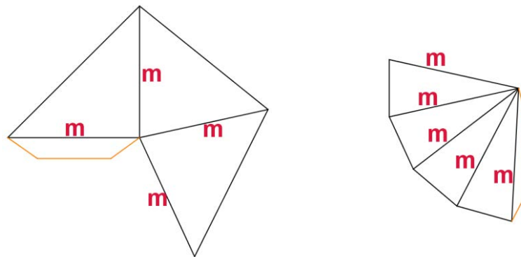
Figura 47 – Planificação das peças representativas dos vértices da base (quatro peças, à esquerda) e do ápice (uma peça, à direita) da pirâmide quadrangular reta.
