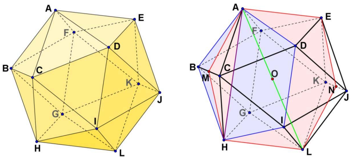
Figura 12 – Representação de pontos, segmentos e planos para o auxílio na determinação do volume de um icosaedro regular.
