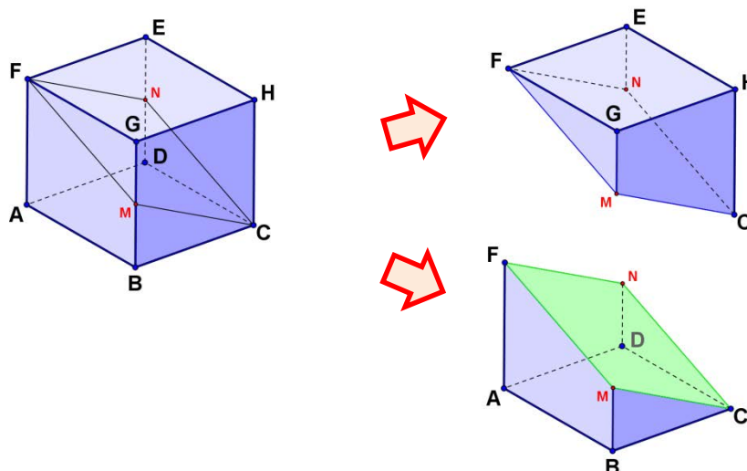
Figura 22 – Processo de planificação de um cubo seccionado por um plano contendo dois vértices diagonalmente opostos e pontos médios de duas arestas.
