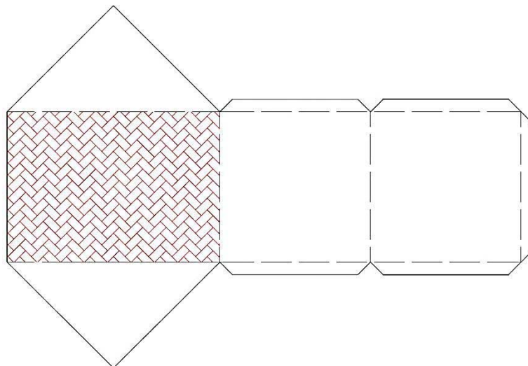
Figura 86 – Planificação de uma das peças de um cubo seccionado por um plano que contém duas arestas paralelas opostas. É um prisma triangular.
