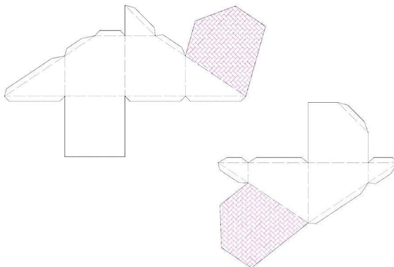
Figura 91 – Planificações das peças originadas do seccionamento do cubo, cuja seção é um pentágono.
