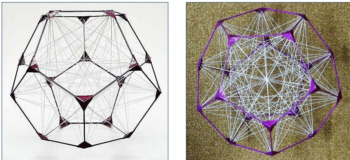
Figura 44 – Fotografias mostrando o dodecaedro regular montado com arame de aço e a representação de suas 100 diagonais internas.
