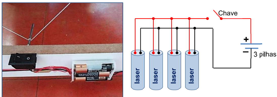
Figura 126 – Interruptor, pilhas e esquema elétrico para a alimentação das fontes de luz laser .
