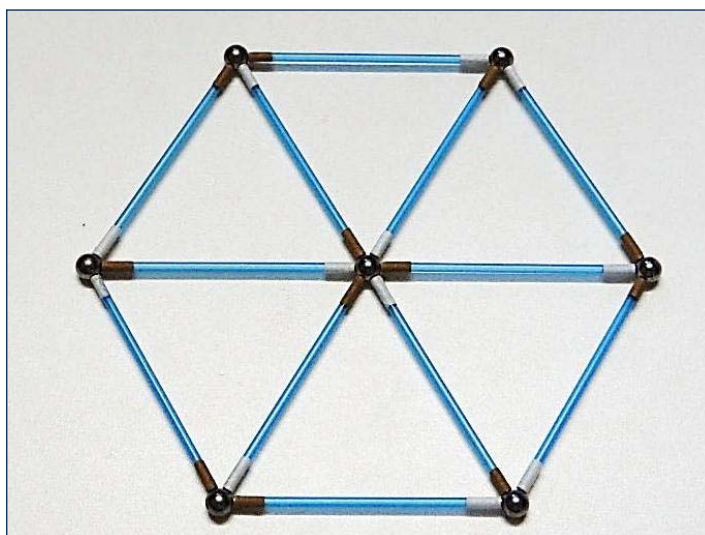
Figura 112 – Fotografia mostrando uma estrutura com triângulos em que é possível observar a permutação entre os polos magnéticos nas junções.
