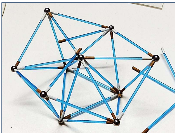
Figura 118 – Fotografia mostrando a tentativa frustrada de montar um icosaedro regular com tetraedros regulares.
