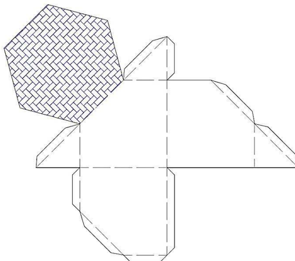
Figura 94 – Planificação de uma das peças do seccionamento do cubo, originando um hexágono regular como uma das faces.
