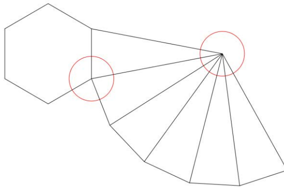
Figura 51 – Planificação da pirâmide hexagonal reta, destacando as peças representativas dos vértices.
