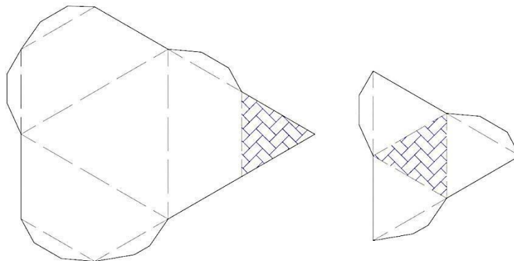
Figura 74 – Planificação das peças seccionadas do tetraedro regular. No processo, foi formado um pequeno tetraedro regular (direita) e um tronco-tetraedro (esquerda).
