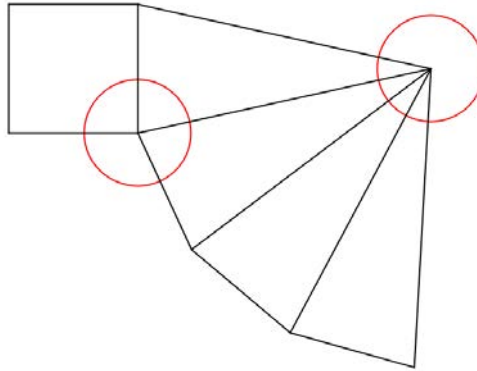
Figura 46 – Planificação de uma pirâmide quadrangular destacando os pontos de interesse para a construção das peças representativas dos vértices.
