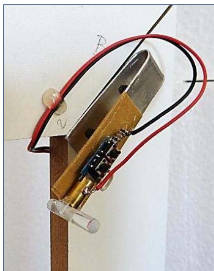
Figura 122 – Partes do apontador laser utilizado na montagem.
