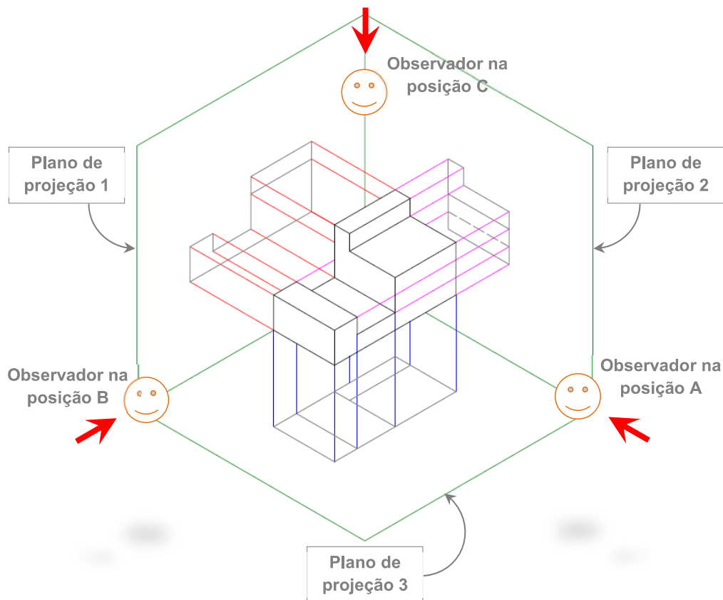
Figura 18 – Projeções do objeto em três planos ortogonais.
