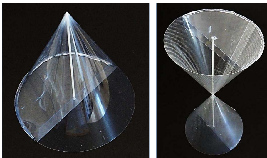
Figura 135 – Fotografias do cone e duplo cone montados com folhas plásticas para visualização de seções.
