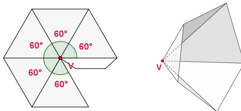
Figura 39 – Planificação da peça representativa do vértice de um icosaedro regular (esquerda) e a peça montada (direita).
