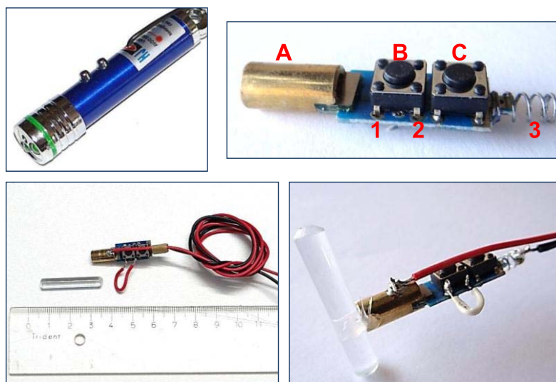
Figura 121 – Fotografias mostrando partes do apontador laser utilizado na montagem.
