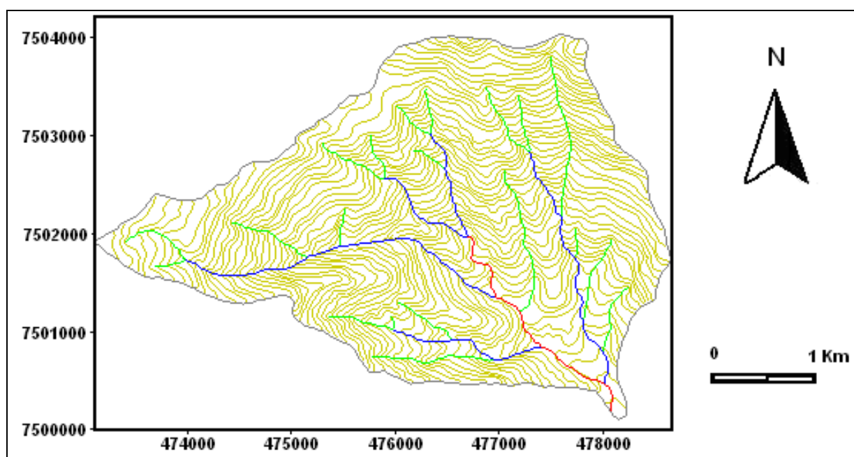
Figura 1. Hierarquização da microbacia do Córrego Tabuleta – Piquete (SP), conforme Strahler (1952).
