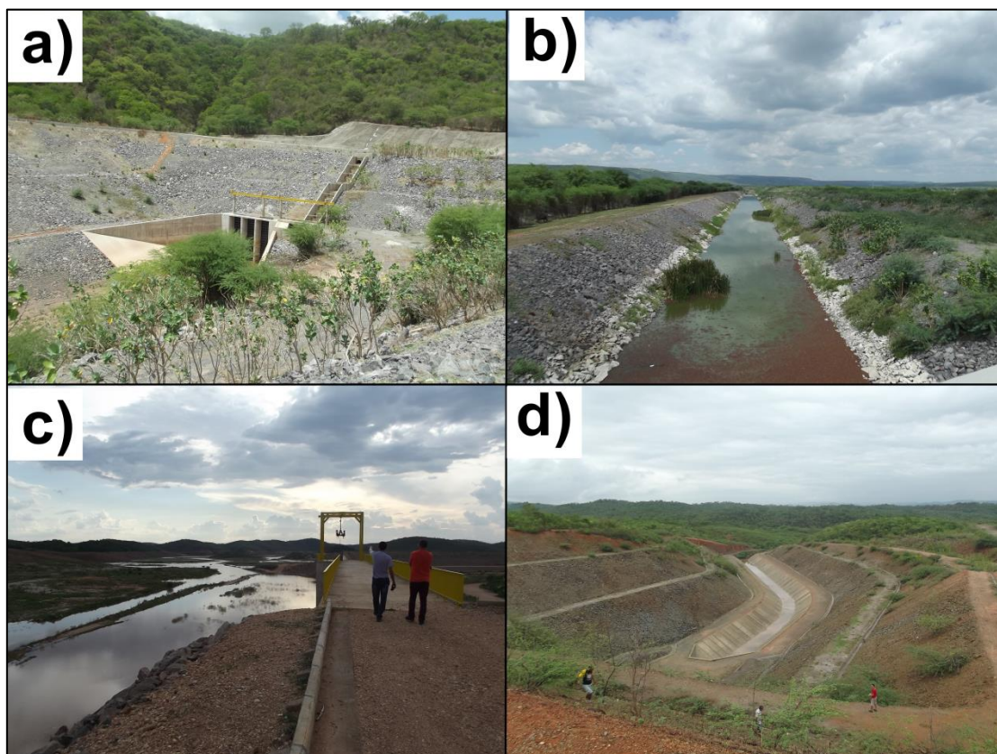
Figura 27. Obras do PISF e CAC na Comunidade São Miguel (a e b), Riacho dos Porcos (c) 50 e Assentamento 10 de Abril (d)
