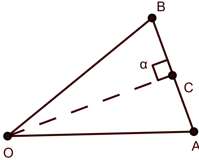
Figura 2.5: Lema 2.6
