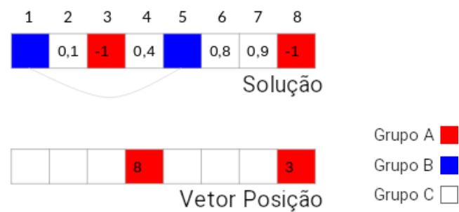
Figura 16 – Algoritmo de Criação de Indivíduos - Passo 3
