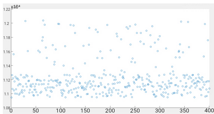
Figura 35 – Valor Dos Indivíduos Resultantes (5000 indivíduos, Valor Ótimo (y) x Experimento (x), Desvio padrão: 261,2)
