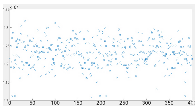
Figura 25 – Valor Dos Indivíduos Resultantes (500 indivíduos, Valor Ótimo (y) x Experimento (x), Desvio padrão: 395,5)
