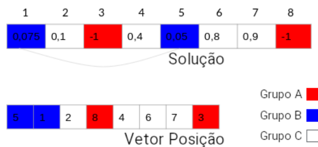
Figura 19 – Algoritmo de Criação de Indivíduos - Passo 6
