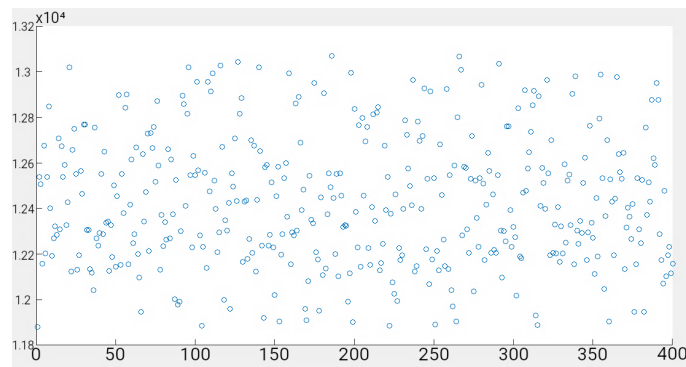
Figura 33 – Valor Dos Indivíduos Resultantes (500 indivíduos, Valor Ótimo (y) × Experimento (x), Desvio padrão: 284,2)
