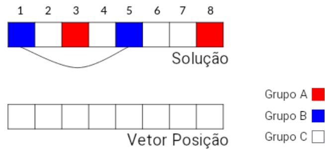
Figura 14 – Início do Algoritmo de Criação de Indivíduos
