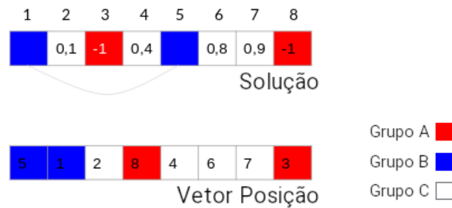
Figura 18 – Algoritmo de Criação de Indivíduos - Passo 5
