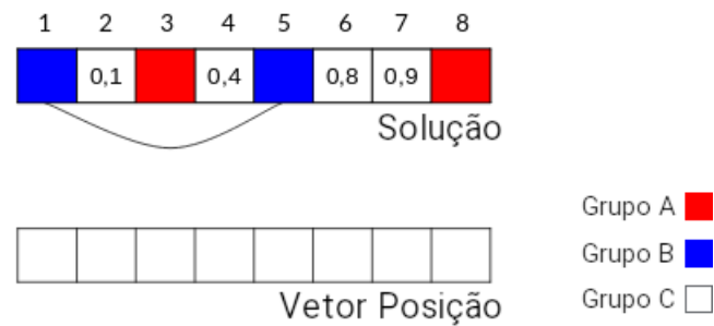
Figura 15 – Algoritmo de Criação de Indivíduos - Passo 2
