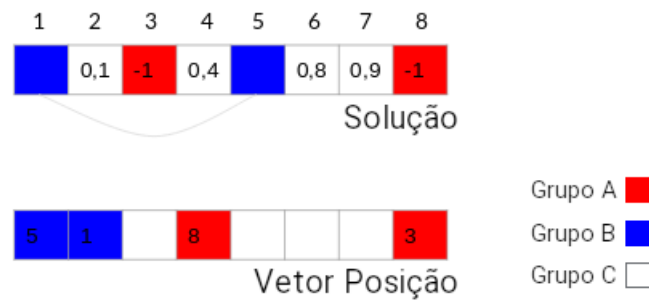
Figura 17 – Algoritmo de Criação de Indivíduos - Passo 4
