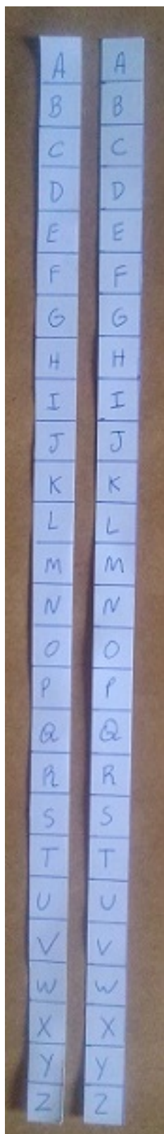
Figura 5.2: Alfabeto
