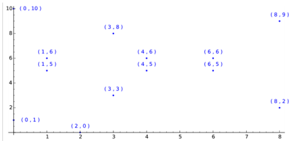
Figura 3.1: Exemplo de curva elíptica y^2 = x^3 + 1x + 1 , imagem elaborada pelo próprio autor.
