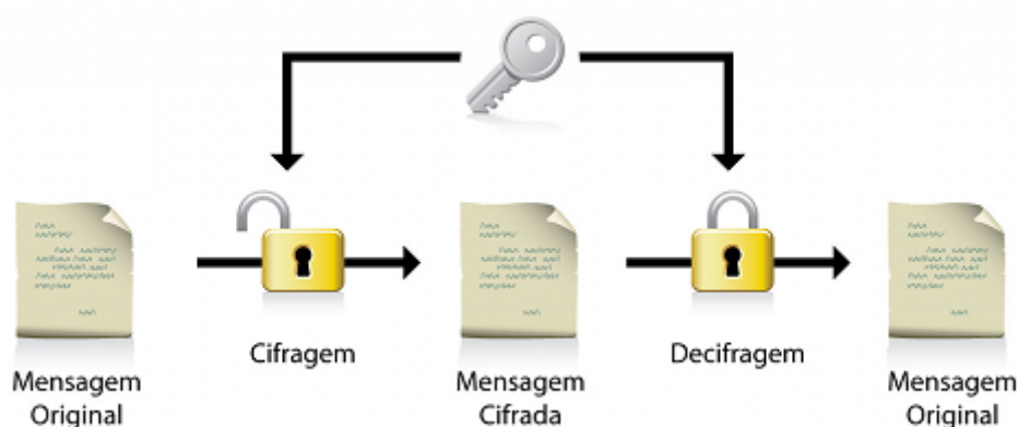
Figura 4.4: Criptografia de chave simétrica. Fonte: http://biblioo.info/certificacao-digital/ . Acesso em 12/02/2016.
