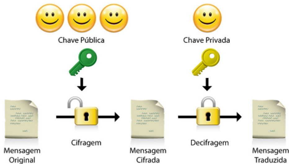
Figura 4.5: Criptografia de chave assimétrica. Fonte: http://biblioo.info/certificacao-digital/ . Acesso em 12/02/2016.
