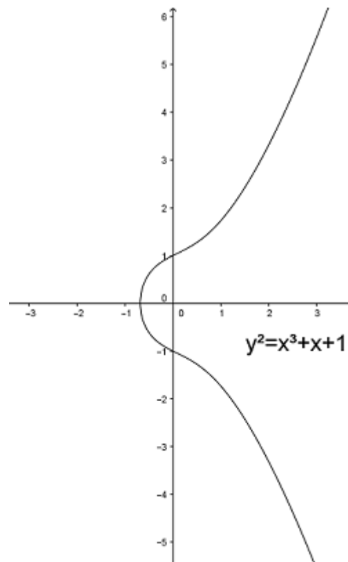
Figura 3.1: Exemplo de curva elíptica y^2 = x^3 + 1x + 1 , imagem elaborada pelo próprio autor.
