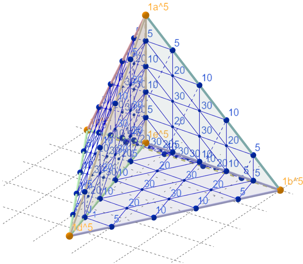
Figura 5.14: Uma representação parcial do Hipertetraedro da expansão de (a + b + c + d + e)^5 .
