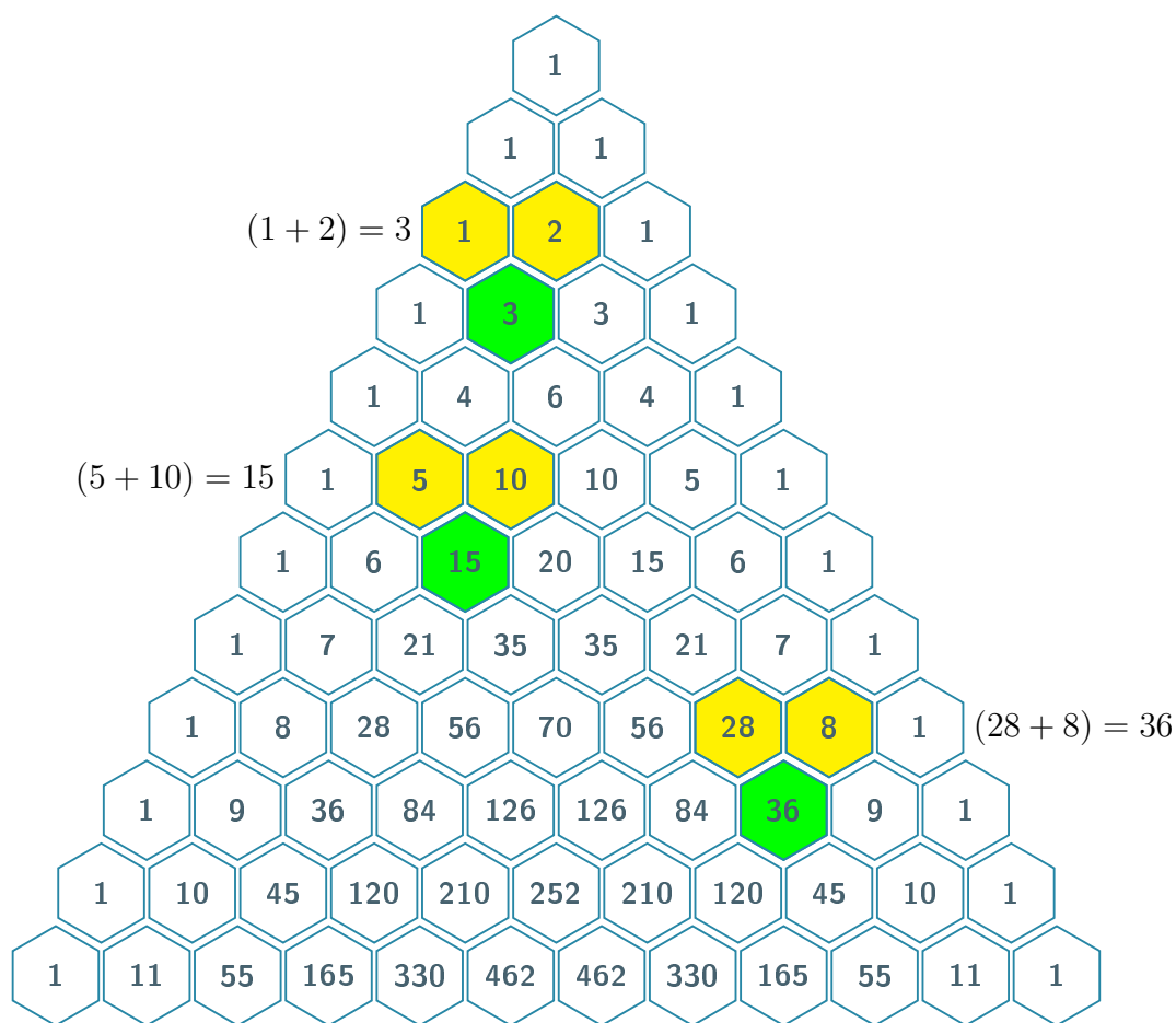
Figura 2.1: Triângulo de Pascal
