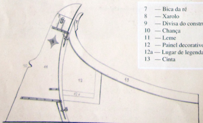
BARCO MOLICEIRO — NOMENCLATURA
