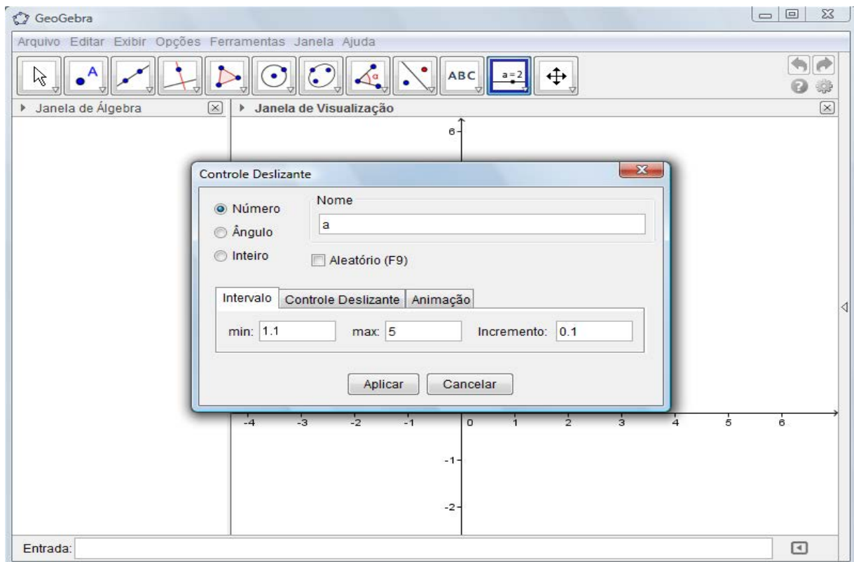
Figura 6: Controle deslizante.
