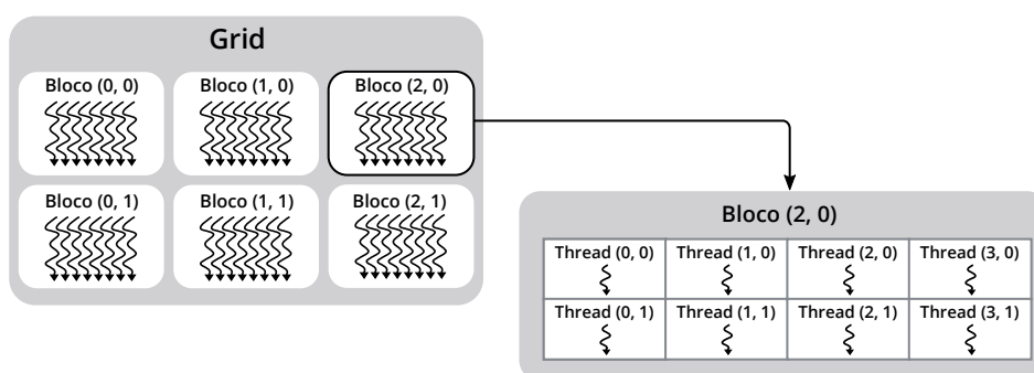
Figura 2.2: Organização das threads na GPU (adaptado de (1))
