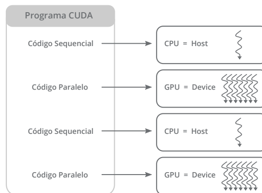
Figura 2.5: Estrutura de um programa CUDA (adaptação de (1))
