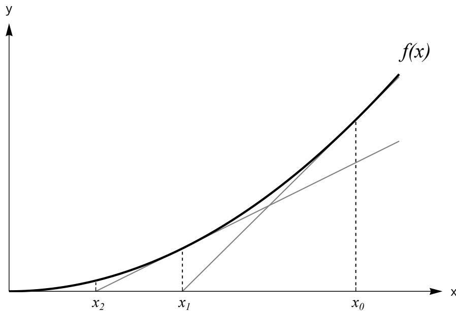
Figura 4.3: Iterações do método de Newton-Raphson
