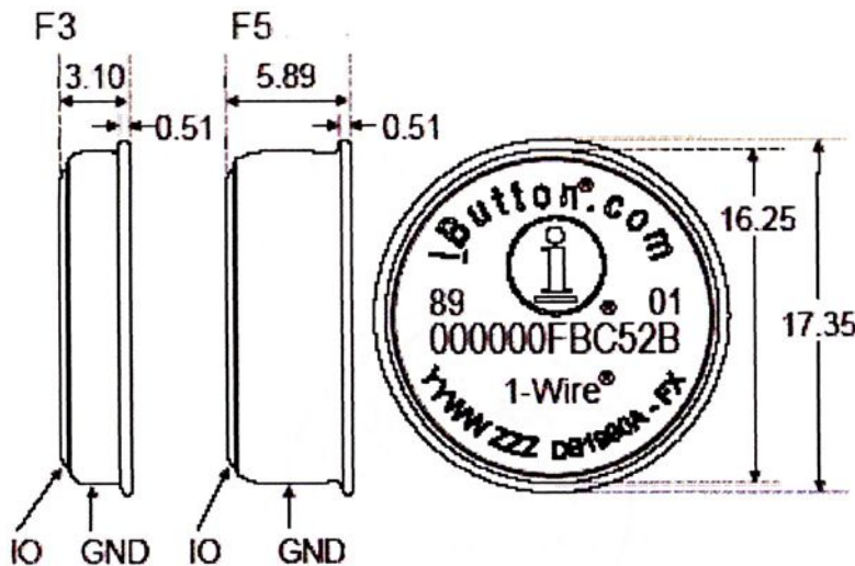
Figura 2.3: Medidas dos iButton 's.
