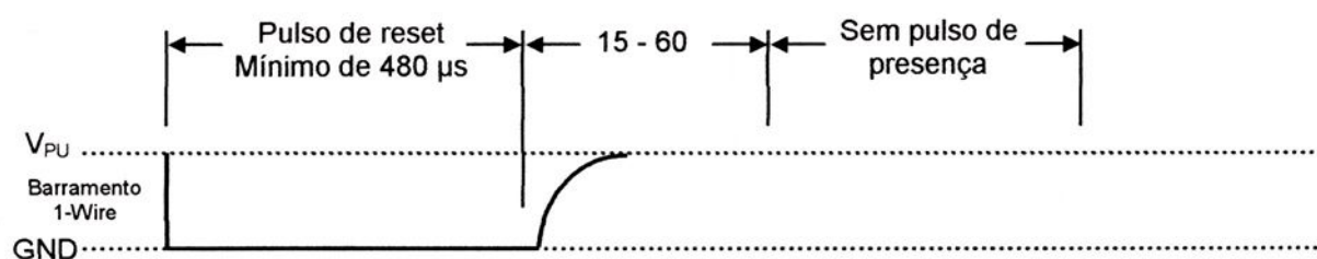
Figura 3.2: Tempo do pulso de reset sem a detecção de dispositivo.
