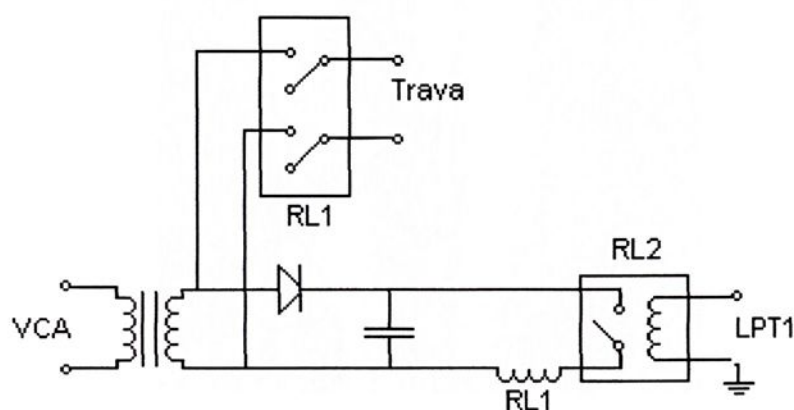
Figura 4.27 : Esquemático circuito de potência.
