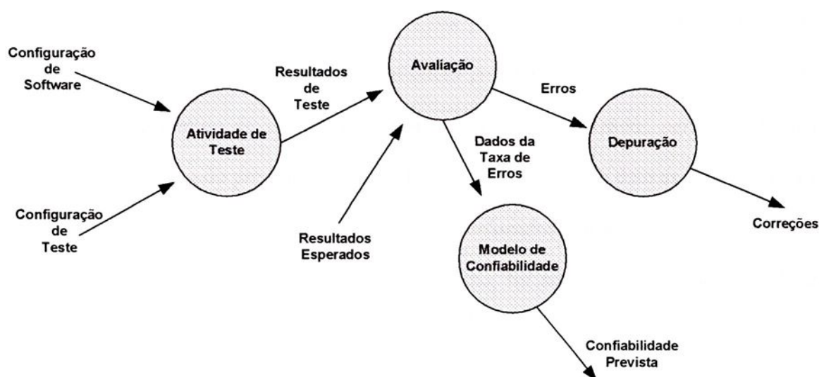
Figura 5.1 : Fluxo de informações da atividade de teste de software .
