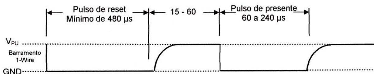
Figura 3.1: Tempos do pulso de reset e pulso de presença.
