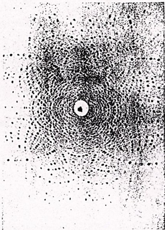
FIG. 163. Lauediagrama del berilo, tallado paralelamente a una cara del prisma hexagonal de primera especie, mostrando dos planos de simetría cuya intersección corresponde a la traza de un eje binario. (Fot. Dr. W. M. Lehmann)
