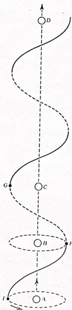
FIG. 219. Línea helicoidal que describe la Tierra a consecuencia del movimiento de traslación del sistema solar en el espacio
