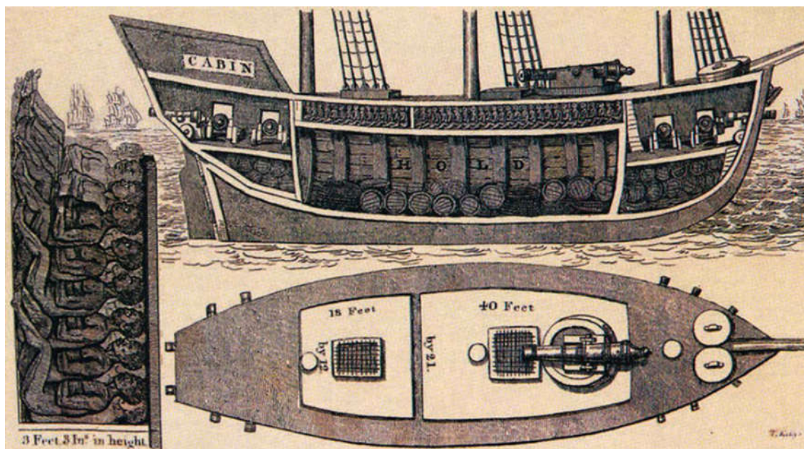
Imagem 4: Planta baixa; corte longitudinal e destaque das acomodações dos escravizados no navio negreiro Veloz de bandeira portuguesa que iria para o Brasil, desenho efetuado pelo Reverendo Robert Walsh e publicado em 1835 (Detalhe). Fonte: WALSH, Robert. Notícias do Brasil (1828-1829). Tradução de Regina Régis Junqueira. Belo Horizonte: Editora Itatiaia, São Paulo: Editora da Universidade de São Paulo, 1985, p. 214.
