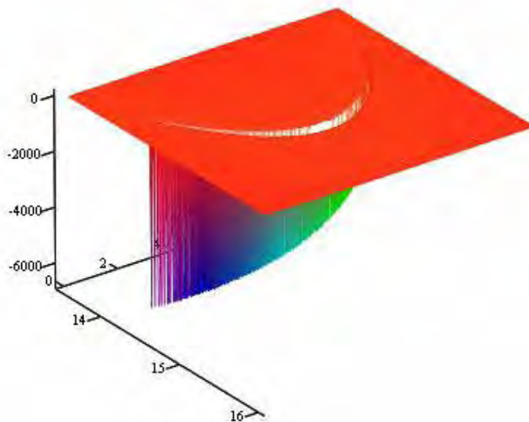
Figura 8.7: Representação de G6(\bar{x}) e as restrições g_1(x_1, x_2) e g_2(x_1, x_2) .
