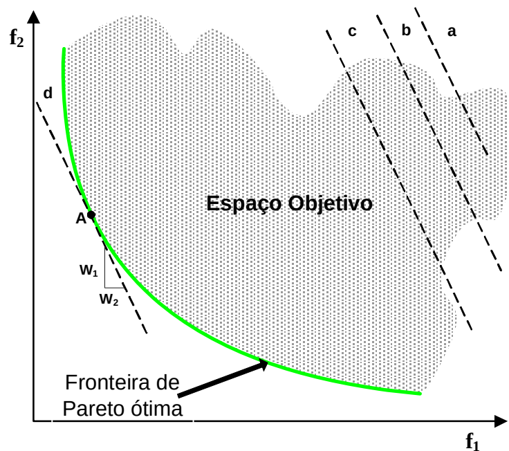
Figura 3.14: Interpretação gráfica do método da soma ponderada.
