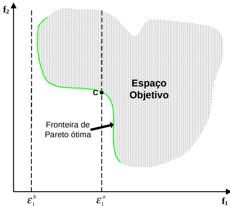
Figura 3.16: Representação do método da restrição- \varepsilon .
