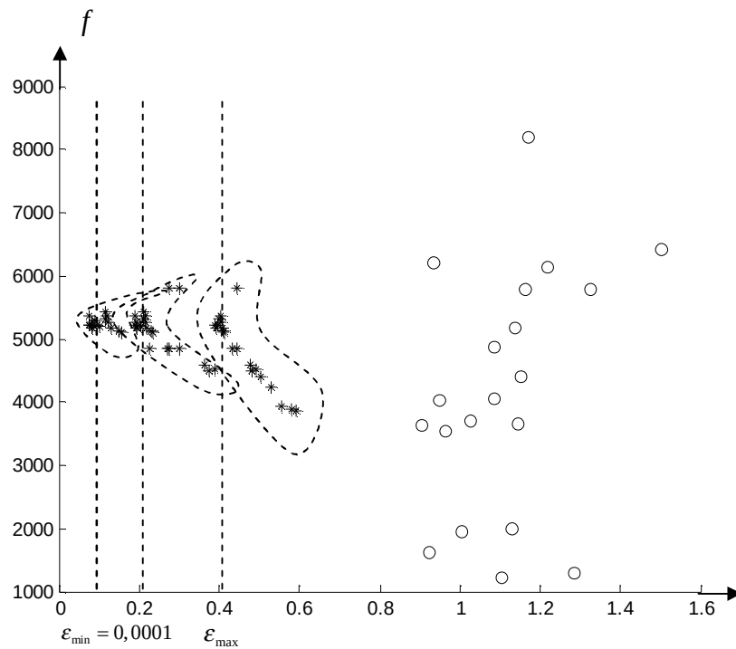
Figura 7.1: Processo de busca por soluções factíveis. Evolução para diferentes valores de \varepsilon .
