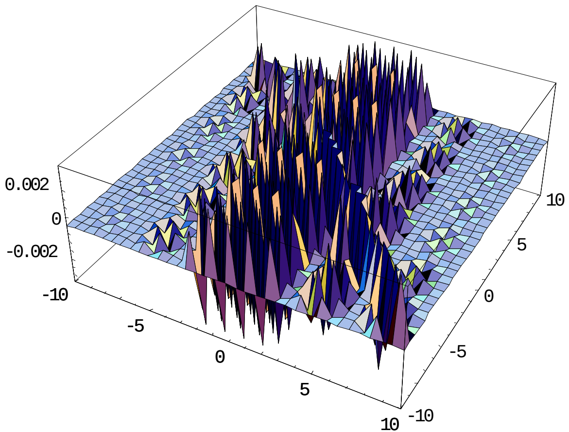
Figura 8.8: Gráfico da função G8(\bar{x}) .
