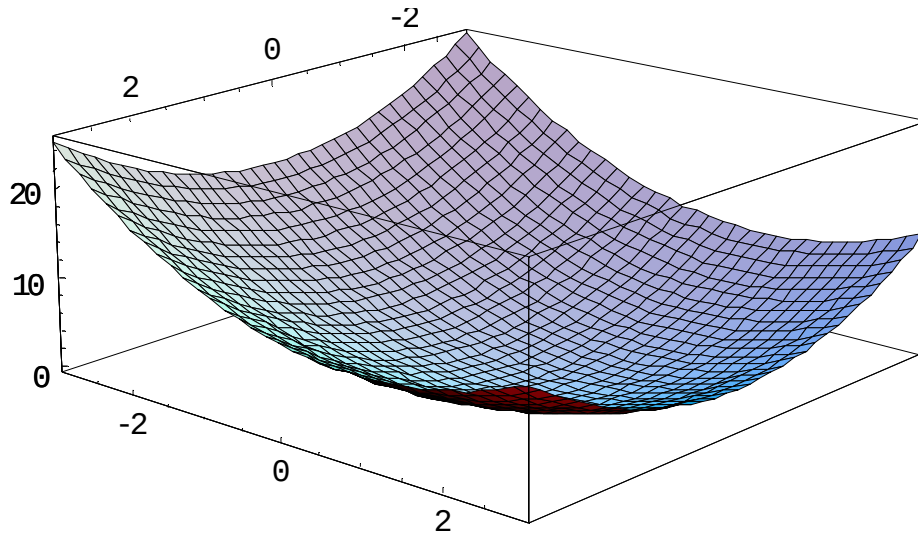
Figura 8.10: Gráfico da função G11(\bar{x}) .
