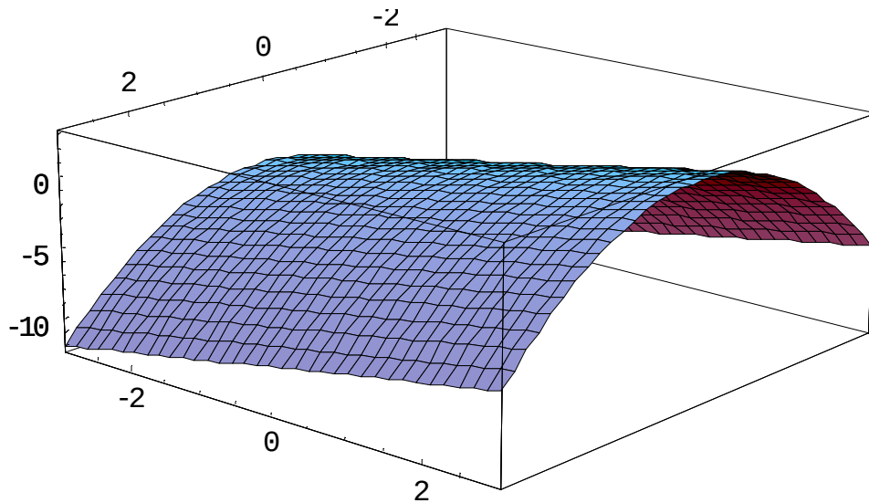
Figura 8.11: Gráfico tridimensional de h(\bar{x}) = x_2 - x_1^2 .
