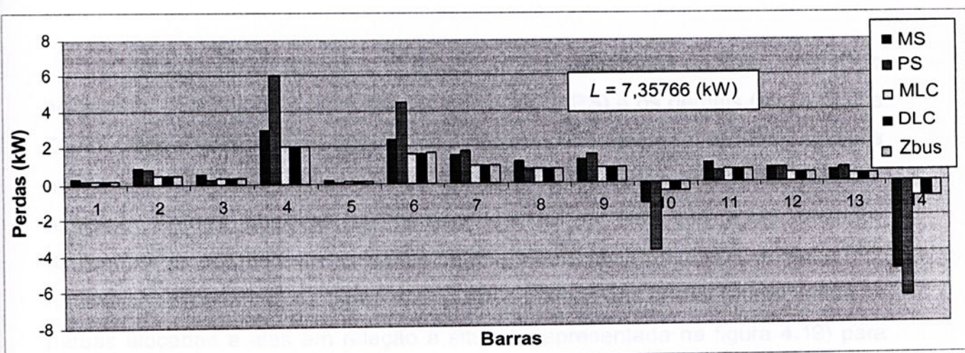
Figura 4.17: Alocação de perdas dos 5 métodos apresentados para o sistema de 15 barras com geradores nas barras 10 ( P_{ger}=3000\text{kW} e Q_{ger}=2000\text{kVAr} ) e 14 ( P_{ger}=400\text{kW} e Q_{ger}=10\text{kVAr} ).
