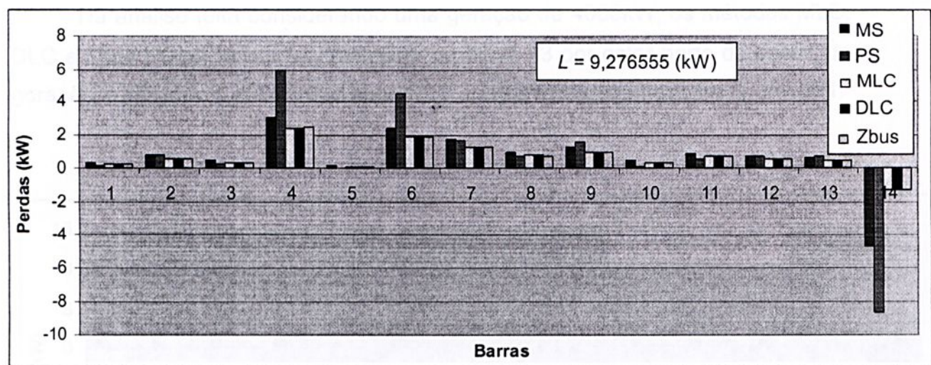
Figura 4.19: Alocação de perdas dos 5 métodos apresentados para o sistema de 15 barras com gerador 1 ( P_{ger}=3000\text{kW} e Q_{ger}=2000\text{kVAr} ) e sem o gerador 2.
