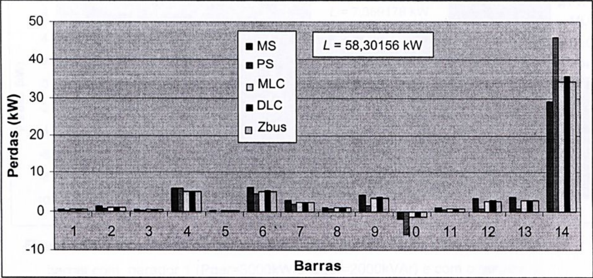
Figura 4.26: Alocação de perdas dos 5 métodos apresentados para o sistema de 15 barras com gerador 1 ( P_{\text{ger}}=0\text{kW} e Q_{\text{ger}}=2000\text{kVAr} ) e com o gerador 2.
