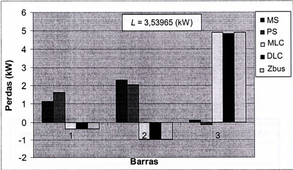
Figura 4.13: Alocação de perdas dos diferentes métodos para o sistema de 4 barras com geração de 500kW na barra 3.
