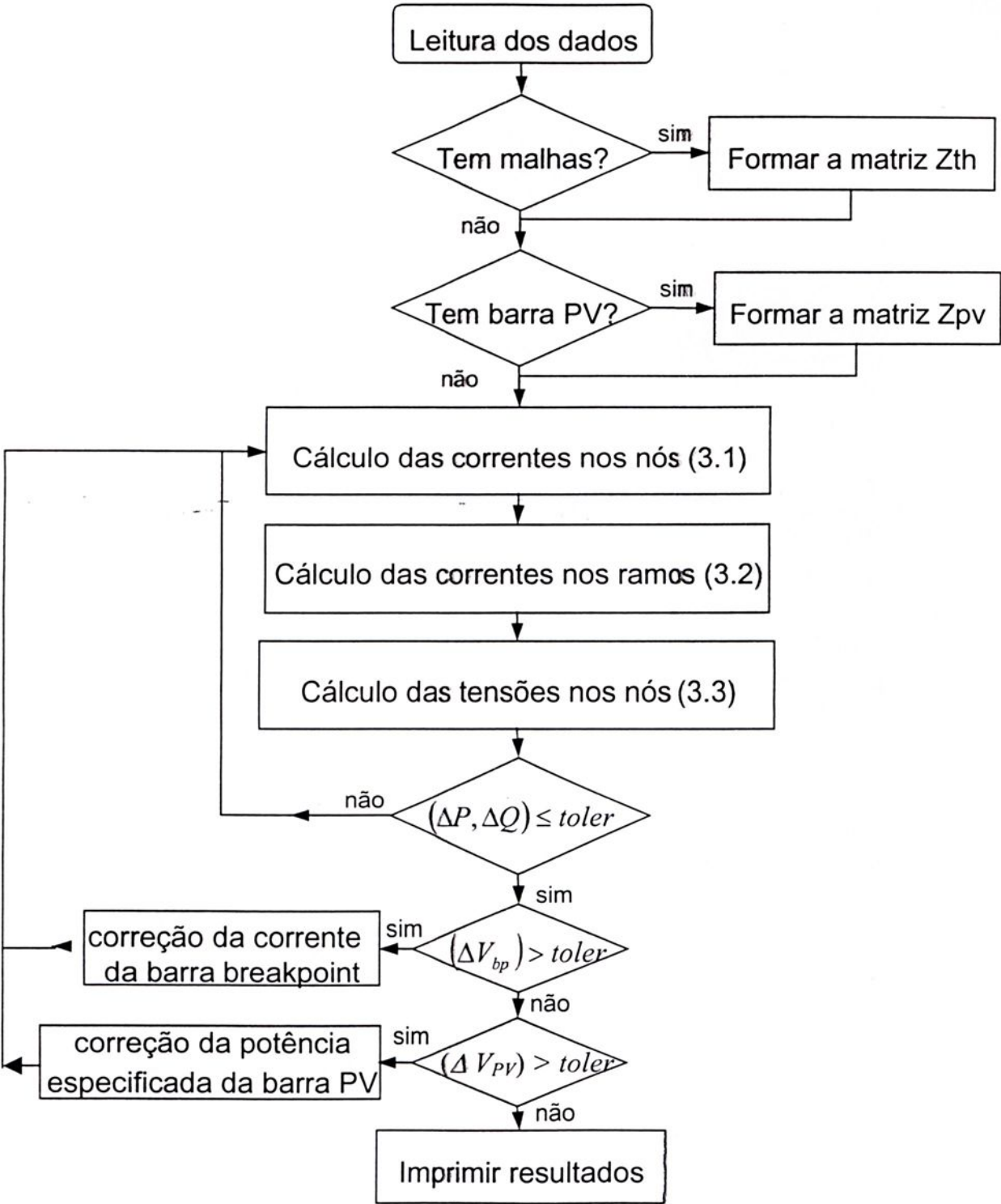
Figura A.3: Fluxograma para o cálculo do fluxo de potência [26].
