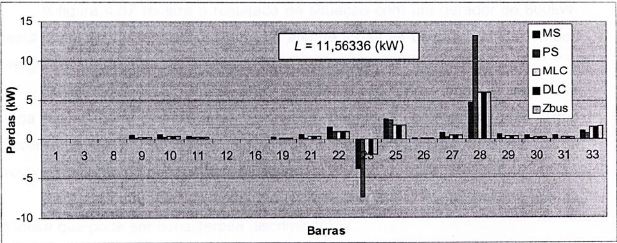
Figura 4.35: Alocação para as barras com carga do sistema IEEE 34 com gerador na barra 23 ( P_{ger}=100\text{kW} ).
