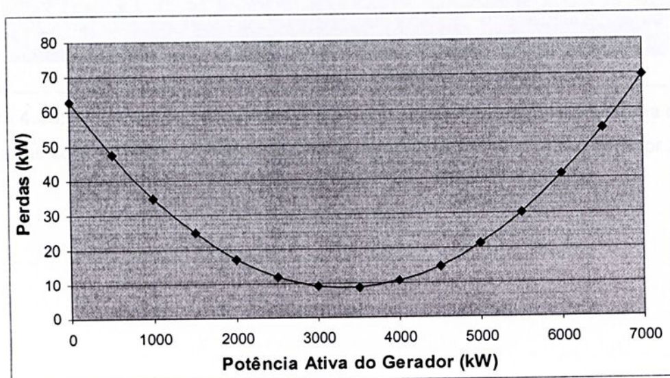
Figura 4.18: Curva das perdas elétricas do sistema, variação da potência ativa do gerador 1 e com o gerador 2 desconectado.
