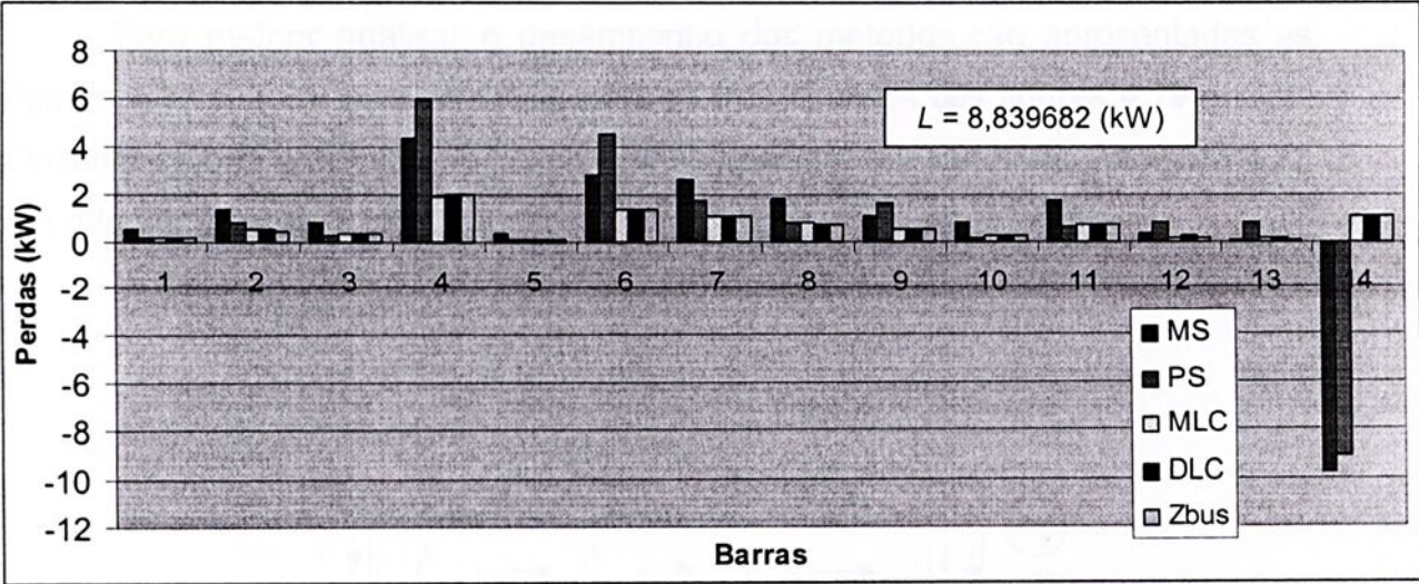
Figura 4.20: Alocação de perdas dos 5 métodos apresentados para o sistema de 15 barras com gerador 1 ( P_{ger}=3500\text{kW} e Q_{ger}=2000\text{kVAr} ) e sem o gerador 2.
