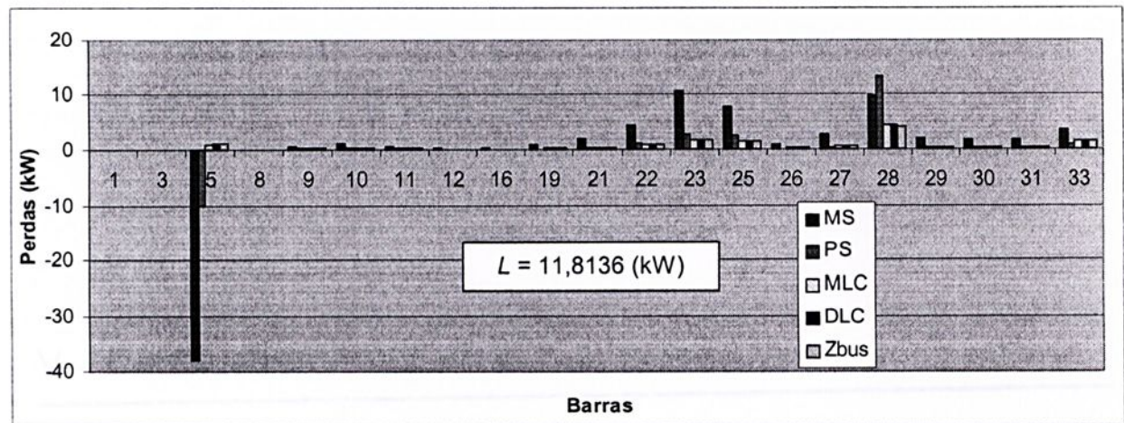
Figura 4.40: Alocação para as barras com carga do sistema IEEE 34 com gerador na barra 5 (Pger=450kW).
