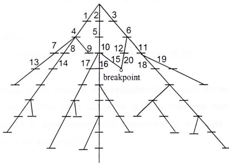
Figura A.2: Rede de distribuição fracamente malhada
