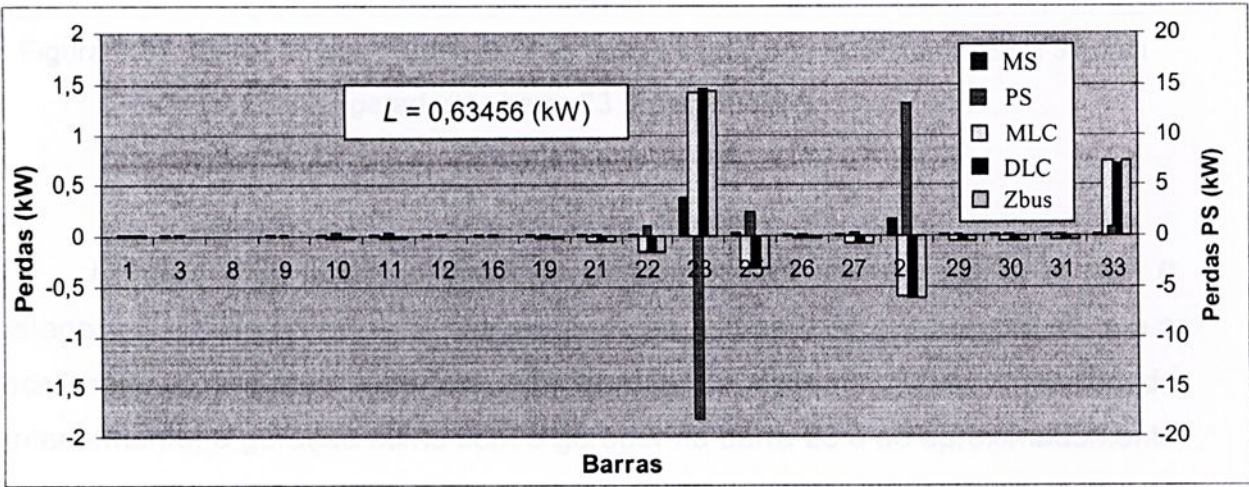
Figura 4.36: Alocação das perdas para as barras com carga do sistema IEEE 34 com gerador na barra 23 ( P_{ger}=400\text{kW} ).
