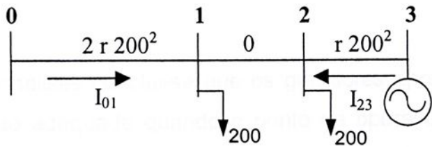
Figura 4.7: Fluxos e perdas com gerador de 200kW.
