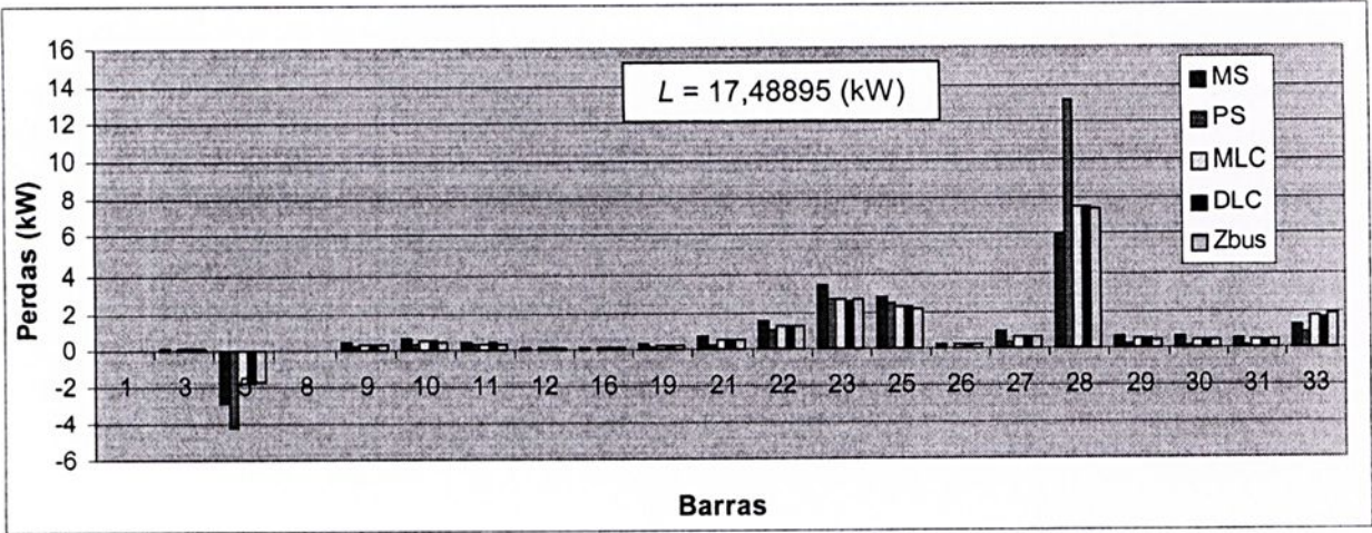
Figura 4.39: Alocação para as barras com carga do sistema IEEE 34 com gerador na barra 5 ( P_{ger}=100\text{kW} ).
