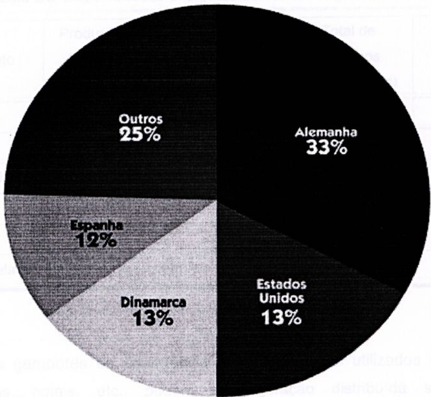
Figura 2.1: Energia eólica – distribuição da capacidade instalada no mundo até outubro de 2000 [11].
