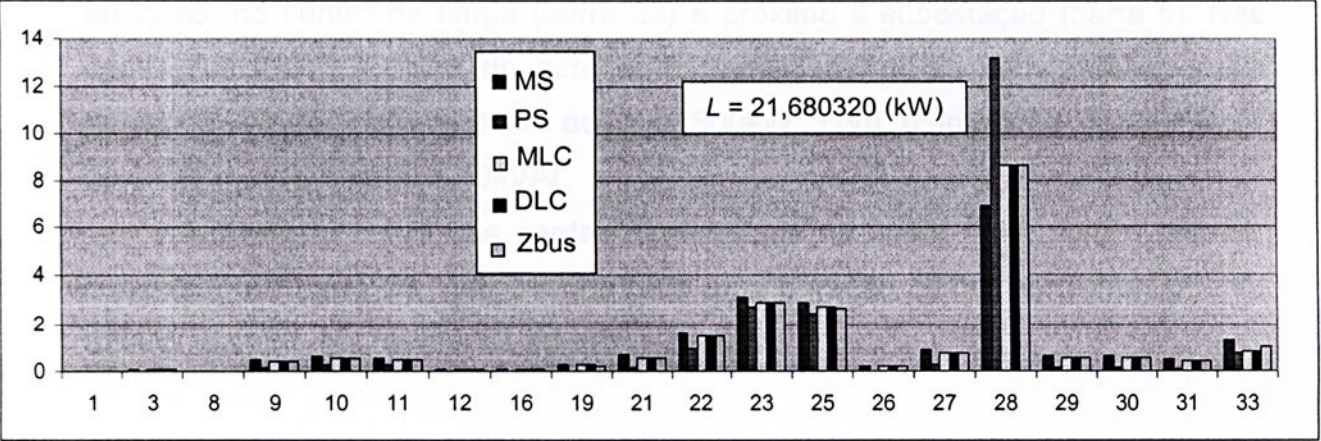
Figura 4.32: Alocação as barras com carga do sistema IEEE 34 sem a presença de gerador.
