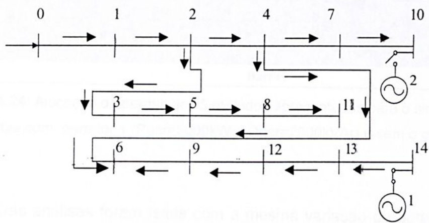
Figura 4.22: Fluxo nas ligações com geração de 300kW na barra 14.
