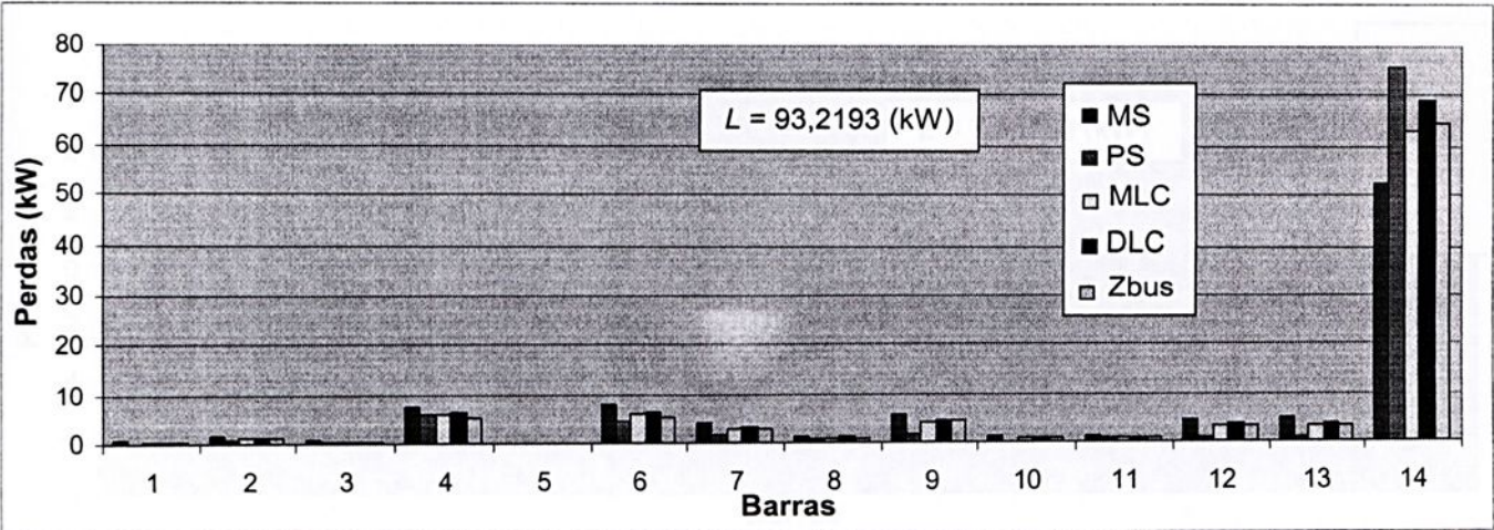
Figura 4.15: Alocação de perdas dos 5 métodos apresentados para o sistema de 15 barras sem gerador.
