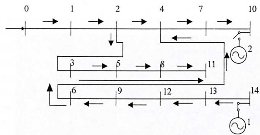
Figura 4.23: Fluxo nas ligações com geração de 400kW na barra 14.
