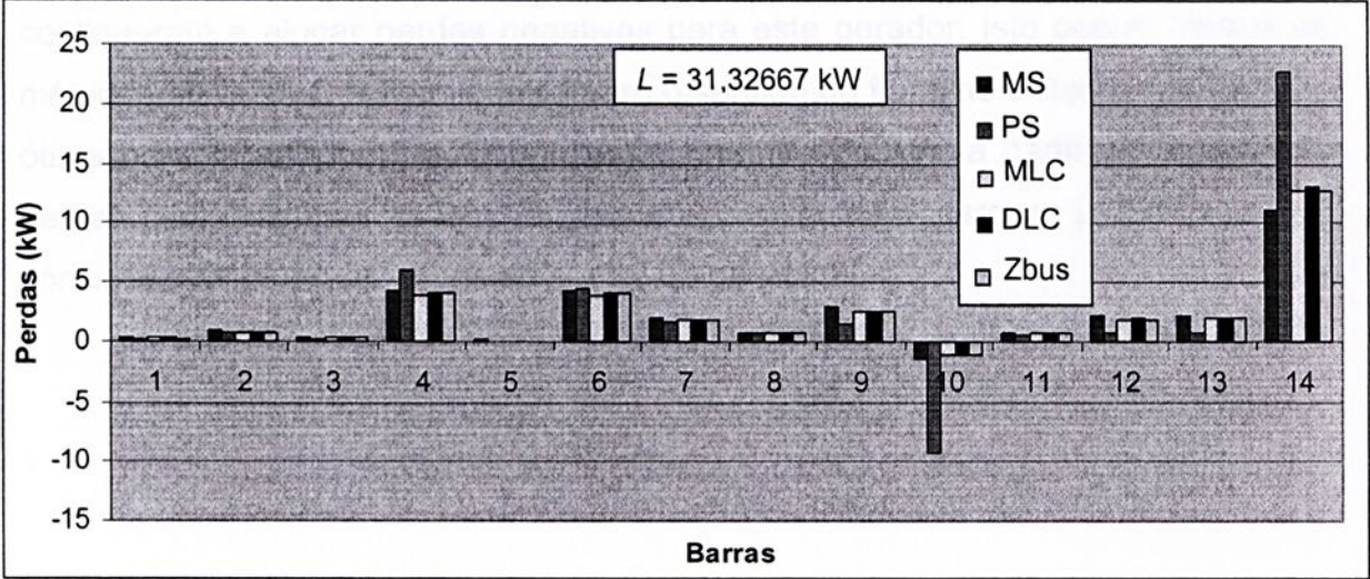
Figura 4.27: Alocação de perdas dos 5 métodos apresentados para o sistema de 15 barras com gerador 1 ( P_{\text{ger}}=1000\text{kW} e Q_{\text{ger}}=2000\text{kVAr} ) e com o gerador 2.
