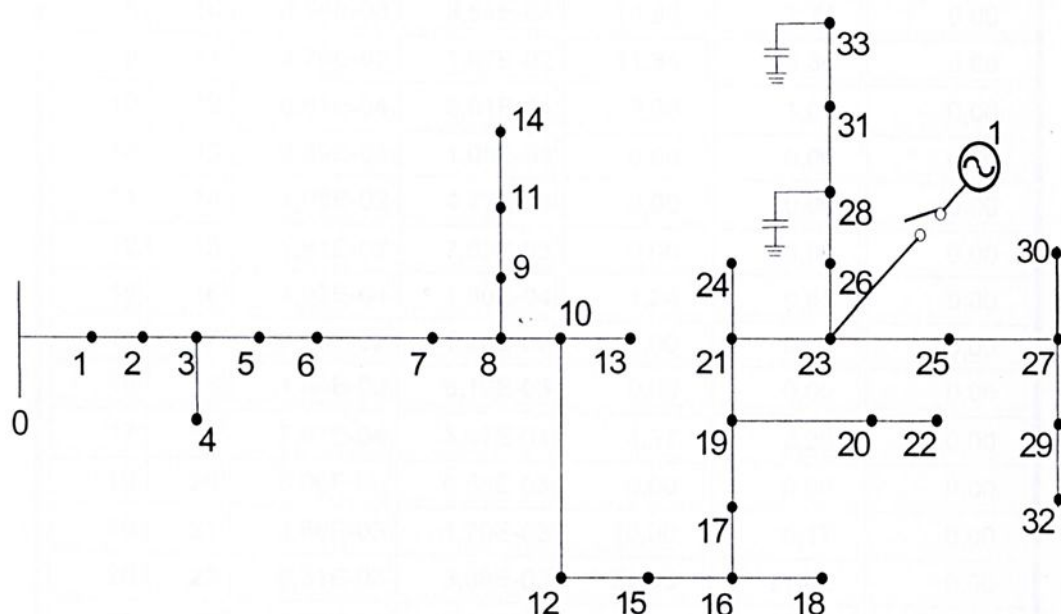
Figura 4.31: Sistema IEEE 34.
