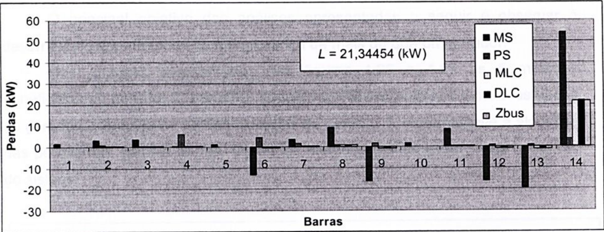
Figura 4.24: Alocação de perdas dos 5 métodos apresentados para o sistema de 15 barras com gerador 1 ( P_{ger}=5000\text{kW} e Q_{ger}=2000\text{kVAr} ) e sem o gerador.
