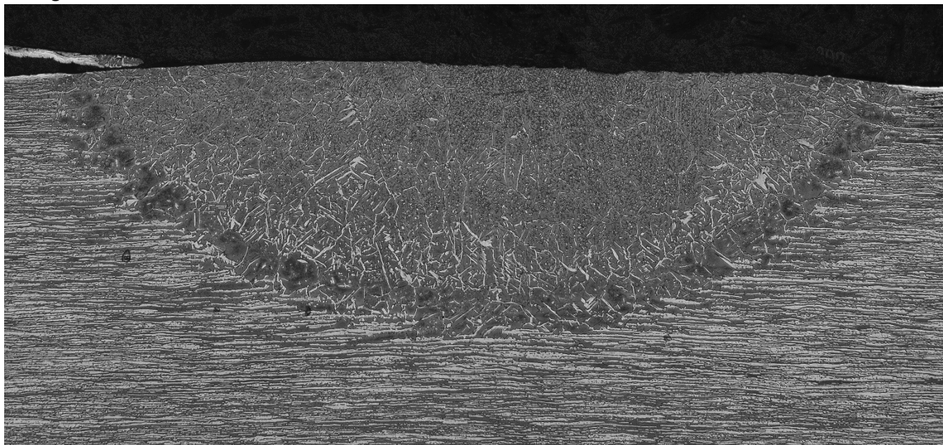
Soldagem GTAW
