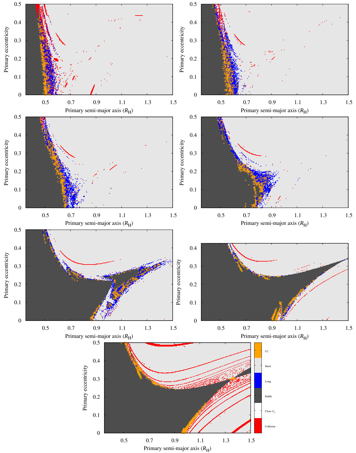
Figura A.2: Mapeamento das condições iniciais primárias tri-dimensionais retrógradas. Analogamente à Figura (A.1), estes mapas correspondem as seguintes inclinações primárias 120^\circ , 130^\circ , 140^\circ , 150^\circ , 160^\circ , 170^\circ , 180^\circ .
