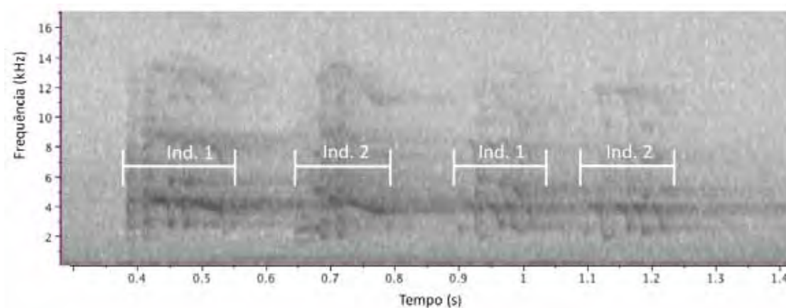
Figura 19. Duetto de quatro notas, onde Ind. 1= Indivíduo 1 e Ind 2= Indivíduo 2. Nota-se o padrão semelhante de notas, com frequência e duração bastante similares.
