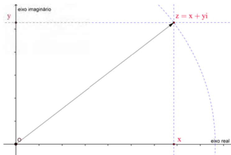
Figura 1.1: Imagem de z
