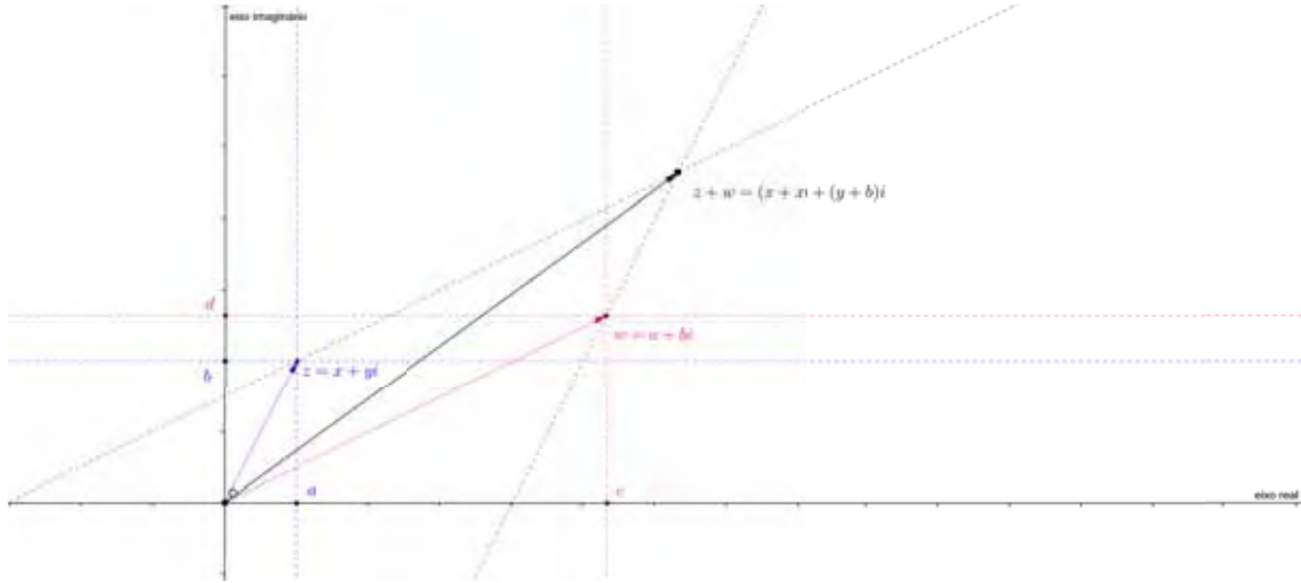
Figura 1.3: Soma de dois números complexos
