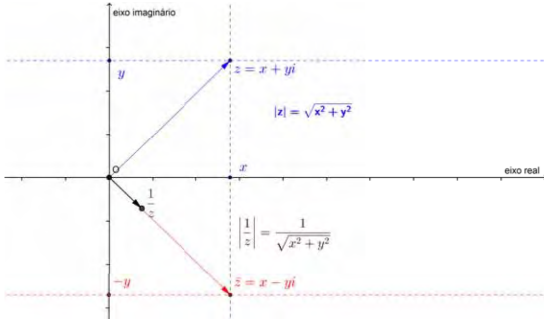
Figura 1.4: Imagem do inverso de um número complexo
