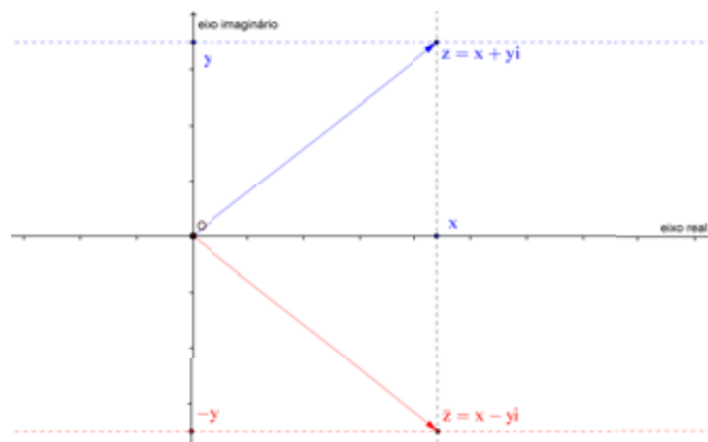
Figura 1.2: Imagem do conjugado
