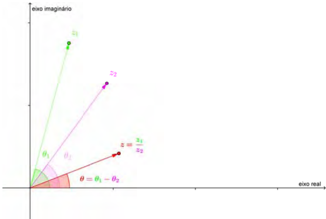
Figura 1.7: Quociente de dois números complexos
