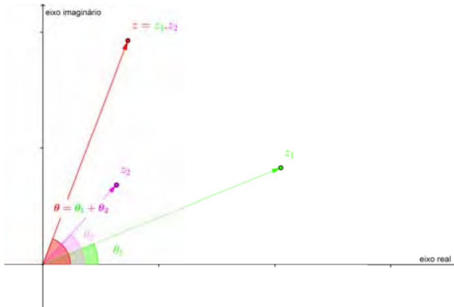
Figura 1.6: Produto de dois números complexos
