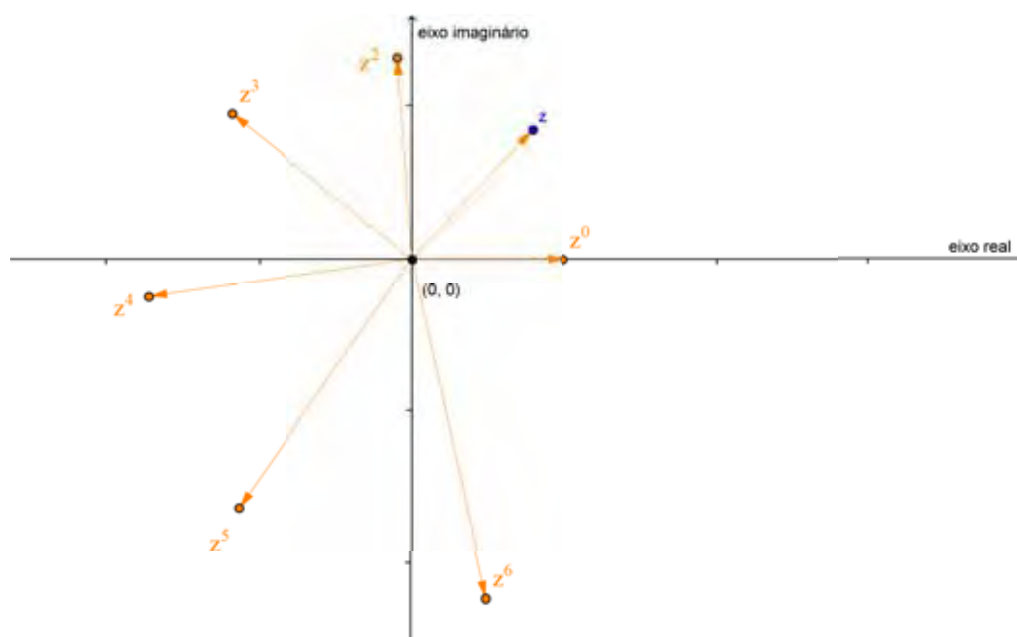
Figura 1.8: Potências de z , |z| = 1 .
