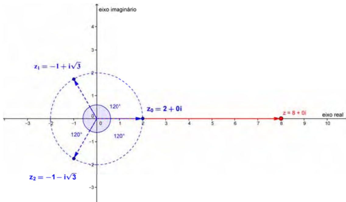
Figura 1.9: Raízes cúbicas de 8.
