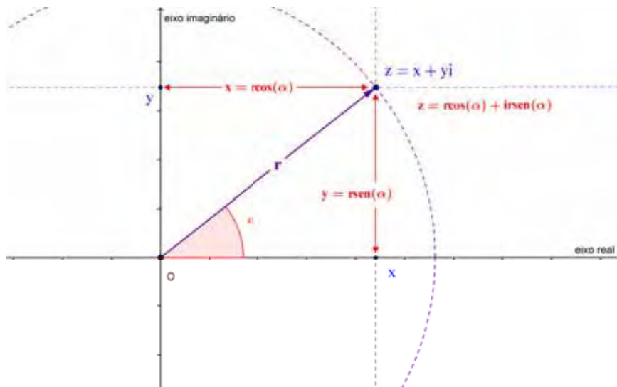
Figura 1.5: Forma polar de número complexo
