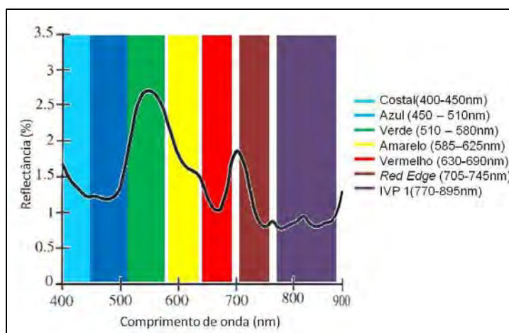
Figura 19 - Comportamento espectral de água com presença de algas e faixas espectrais imageadas pelo sensor World View-2.
