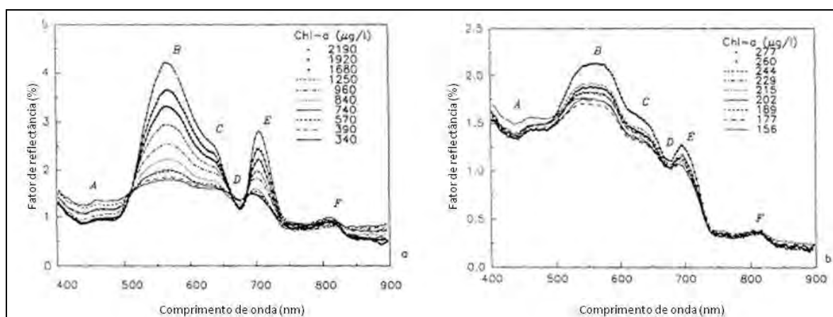
Figura 4 – Curvas de reflectância com diferentes concentrações de clorofila.
