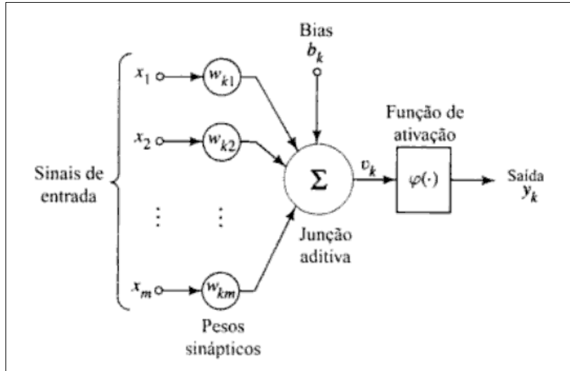
Figura 12 - Modelo de um neurônio não linear.
