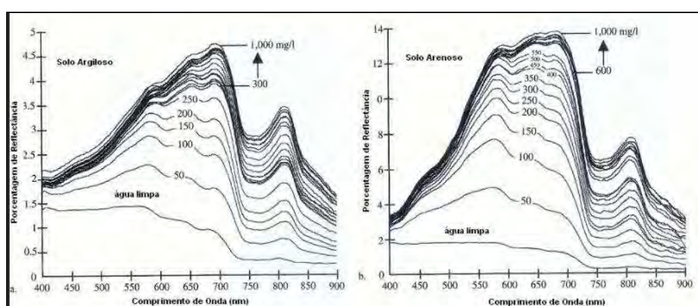
Figura 5 – Medidas in situ de reflectância da água com diferentes concentrações de argila e areia. Fonte: Jensen, 2009.
