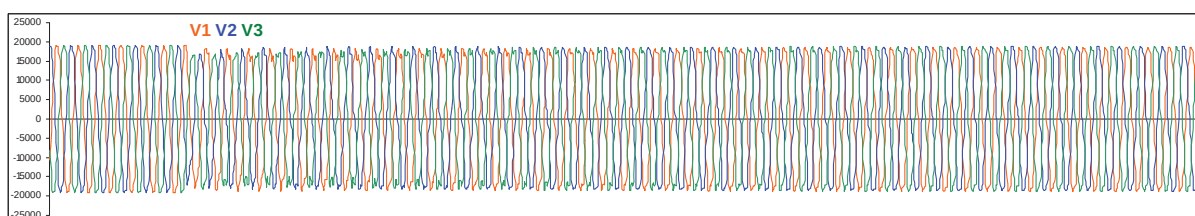
Figura 4.9. Forma de Onda das Tensões – Evento Ocorrido em 2009-set-20 08:48:43,513.
