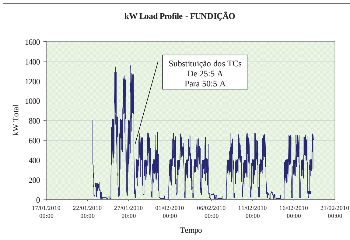
Figura 4.22. Registros de Demanda Total (kW).
