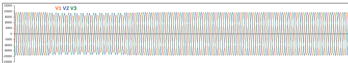
Figura 4.10. Forma de Onda das Tensões – Evento Ocorrido em 2009-set-22 19:15:40,896.
