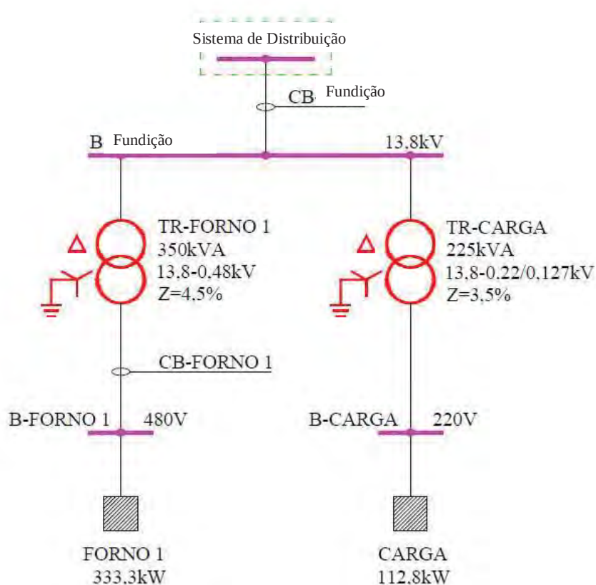
Figura 3.2. Diagrama Unifilar das Instalações do Acessante – Configuração Atual.
