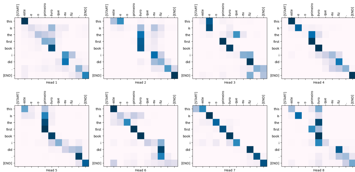
Figura 12 – Mapa de Calor de Atenção espalhado por oito Heads
