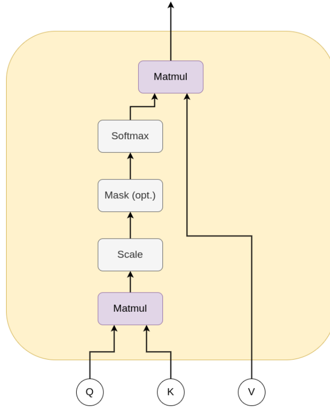
Figura 13 – Função Scaled Dot-Product Attention
