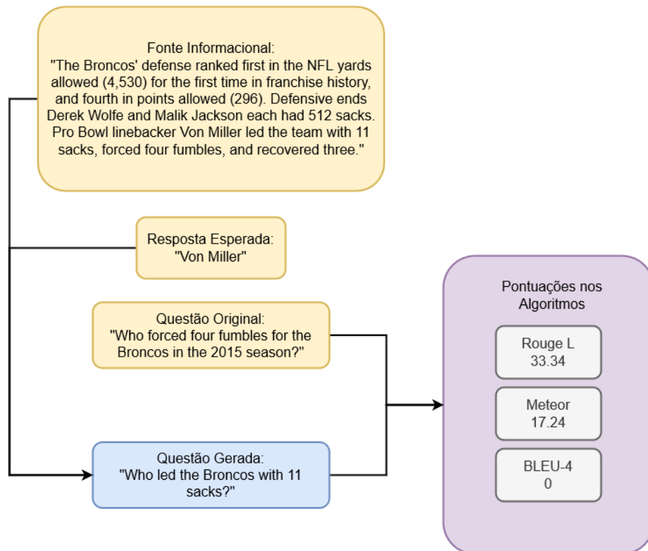
Figura 27 – Pontuações dos algoritmos comparando questões diferentes
