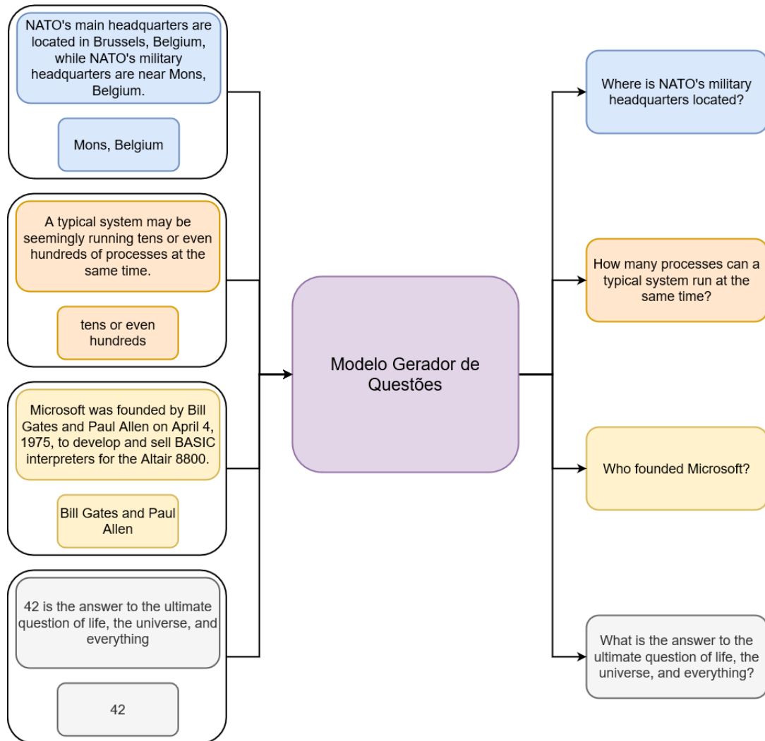
Figura 22 – Processamento do Modelo Gerador de Questões
