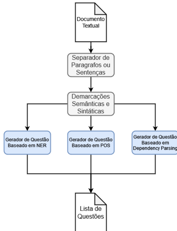
Figura 5 – Exemplo de Arquitetura Utilizando Técnicas Semânticas e Sintáticas
