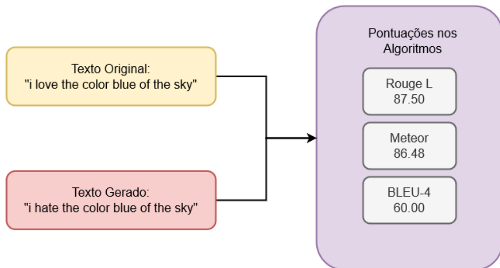
Figura 26 – Pontuações dos algoritmos comparando resultado com palavra de sentido contrário
