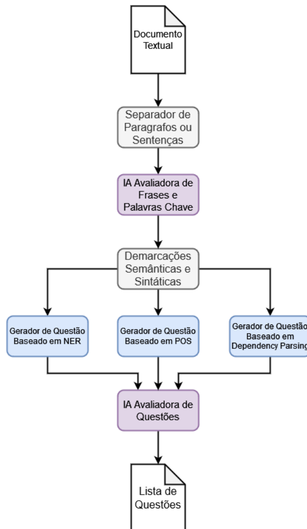
Figura 6 – Exemplo de Arquitetura Utilizando Técnicas Semânticas e Sintáticas Apoiada por IA
