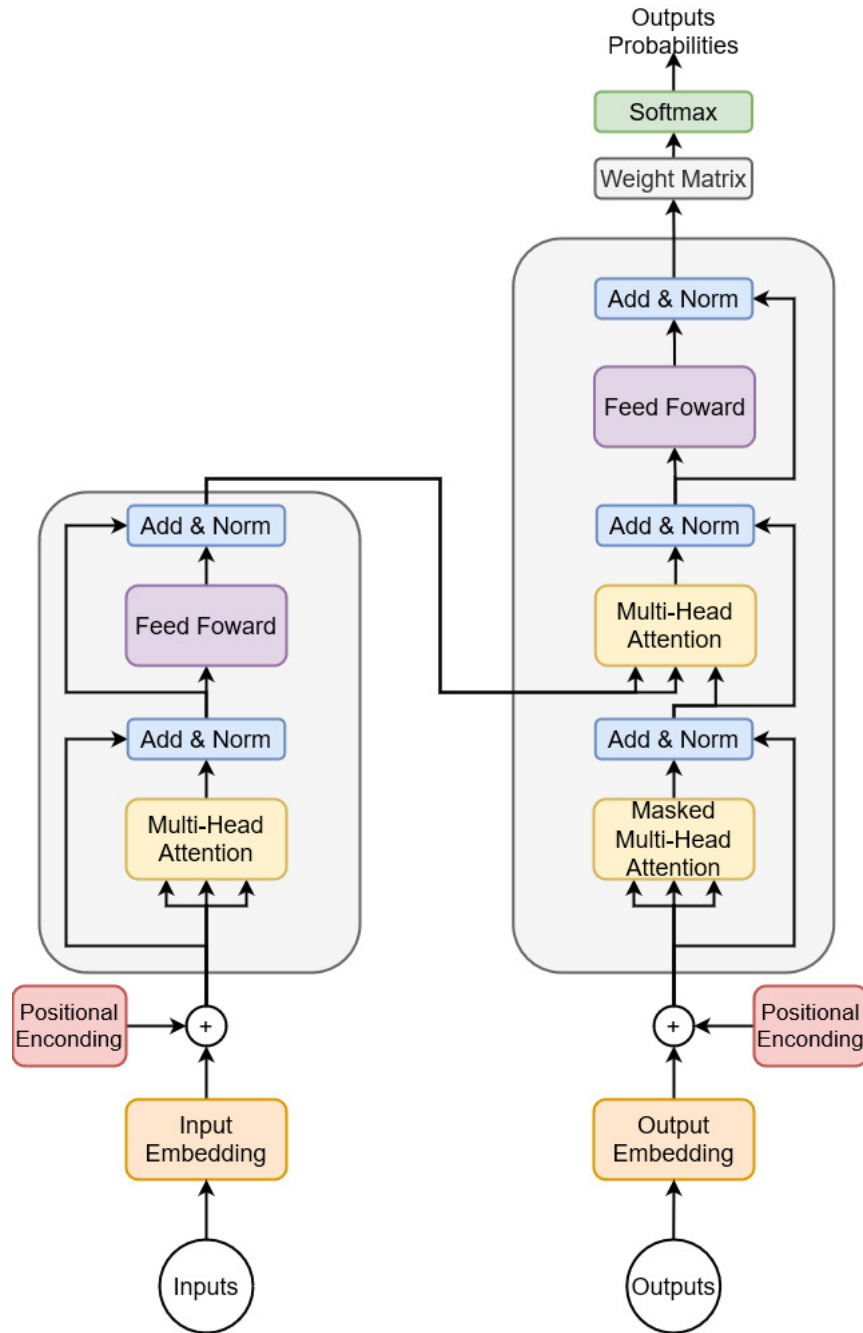
Figura 9 – Arquitetura de Redes transformers
