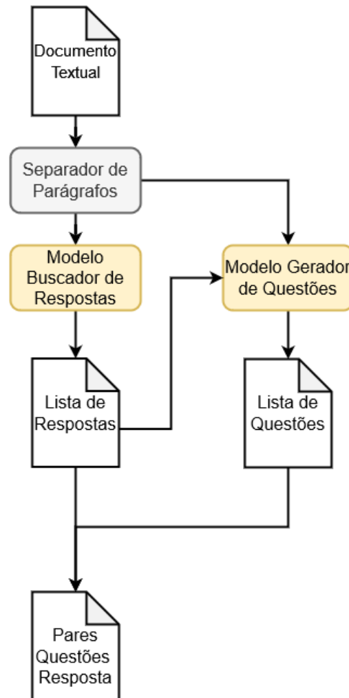
Figura 18 – Arquitetura Multi-Modelo
