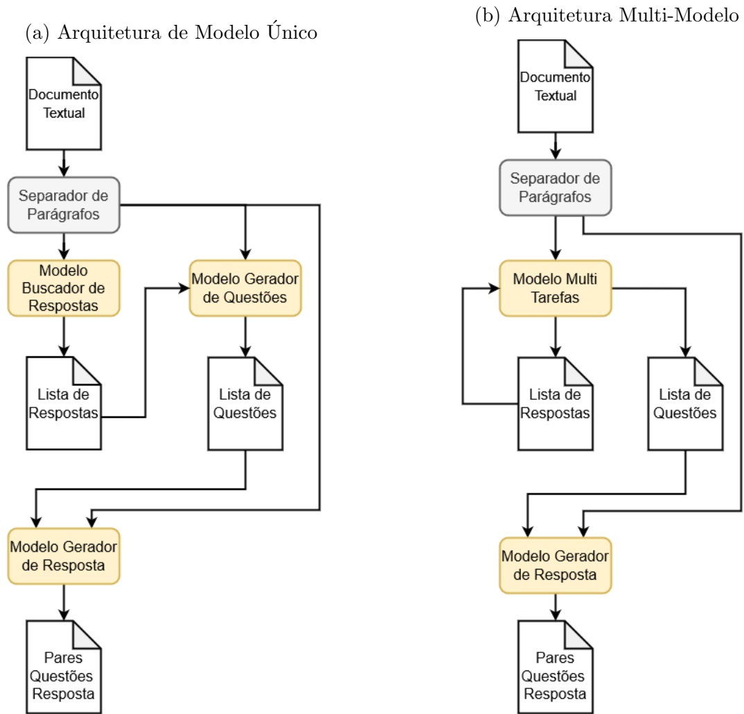
Figura 20 – Arquiteturas com Gerador de Resposta
