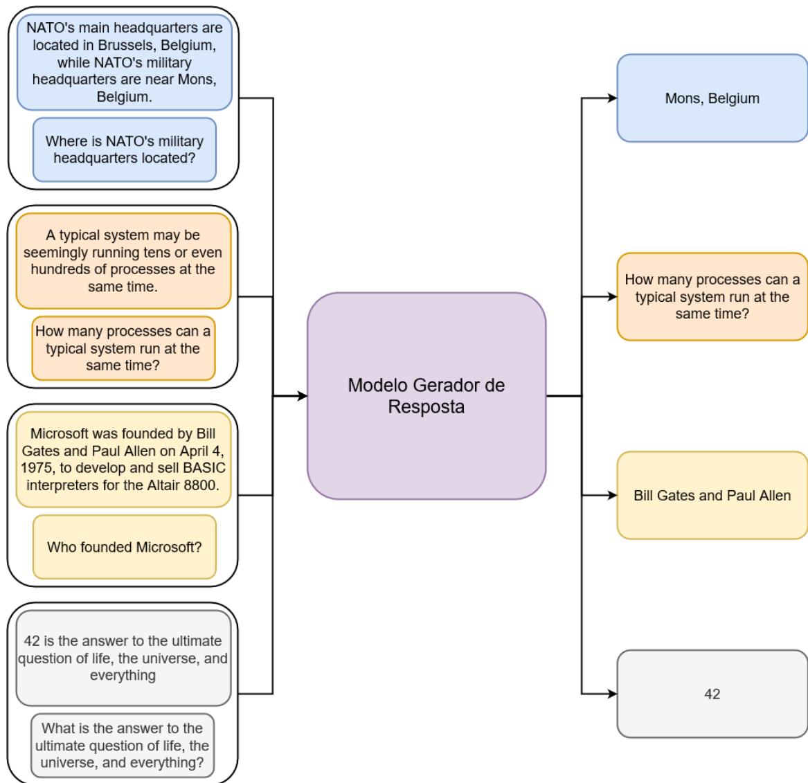
Figura 23 – Processamento do Modelo Gerador de Respostas
