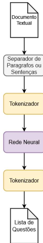
Figura 8 – Exemplo de Arquitetura Utilizando Técnicas de Deep Learning
