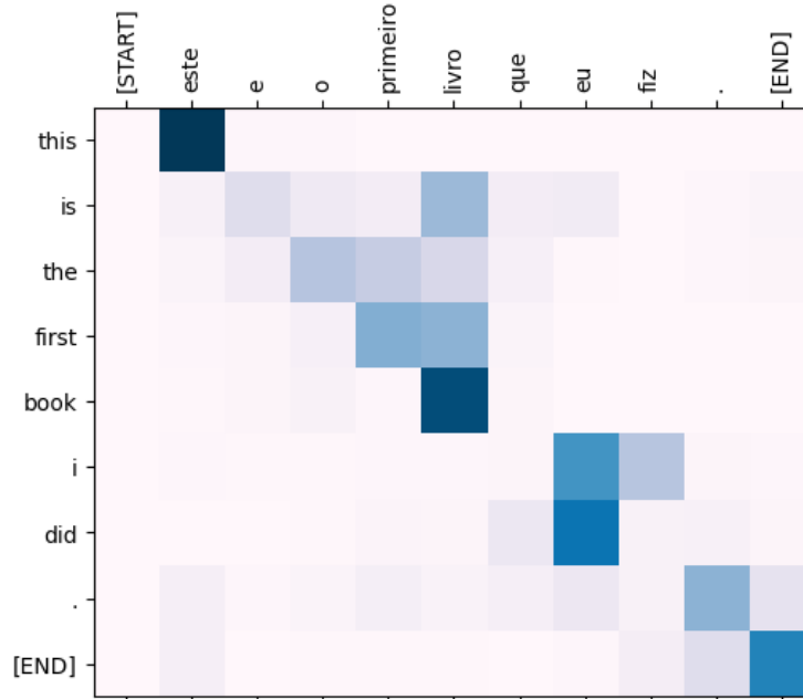
Figura 10 – Mapa de Calor da Atenção
