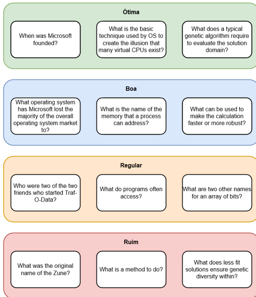
Figura 28 – Exemplos de Questões de Acordo com sua Classificação
