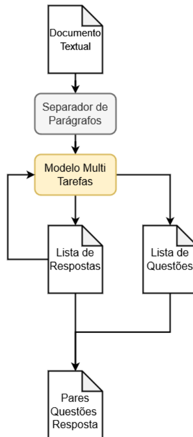
Figura 19 – Arquitetura de Modelo Único
