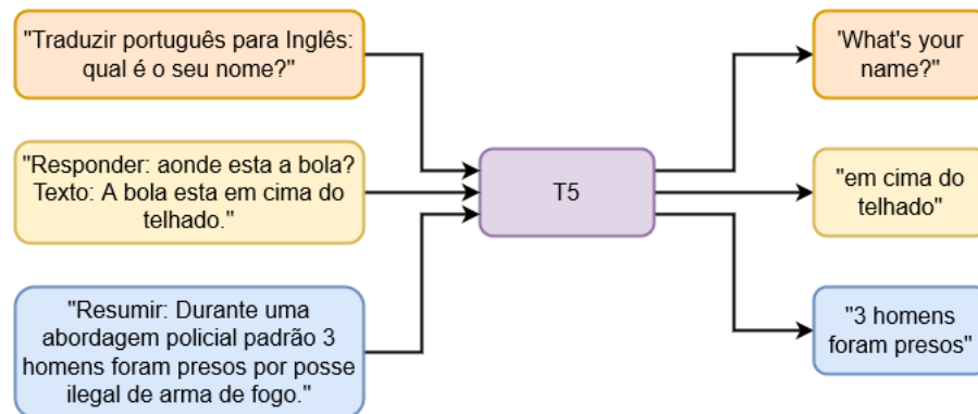
Figura 16 – Modelo de Treinamento T5
