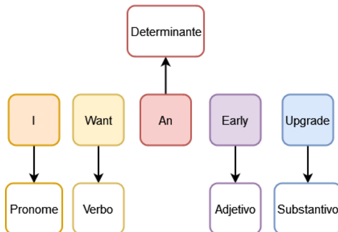
Figura 2 – Demarcação POS
