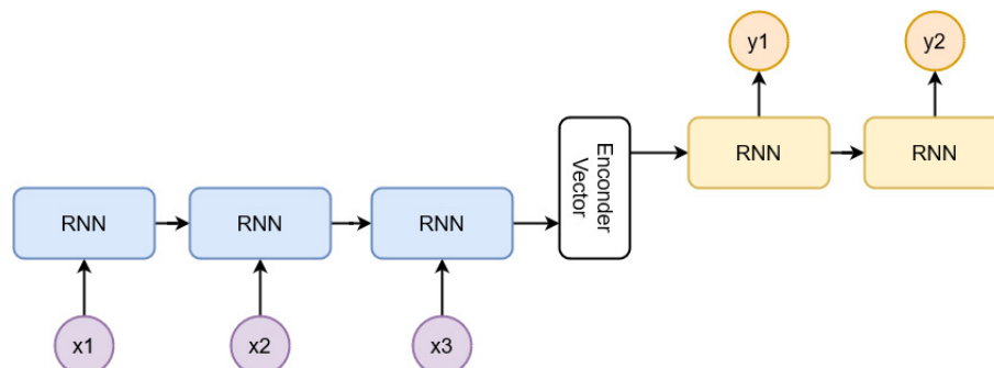
Figura 7 – Modelo Encoder-Decoder
