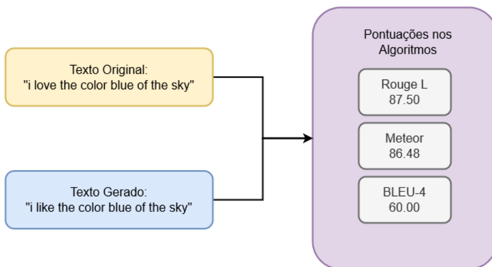
Figura 24 – Pontuações dos algoritmos comparando resultado semelhante
