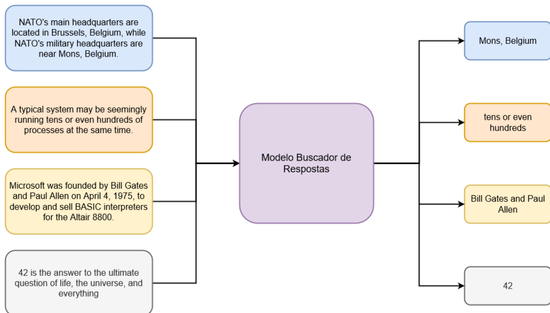
Figura 21 – Processamento do Modelo Buscador de Respostas
