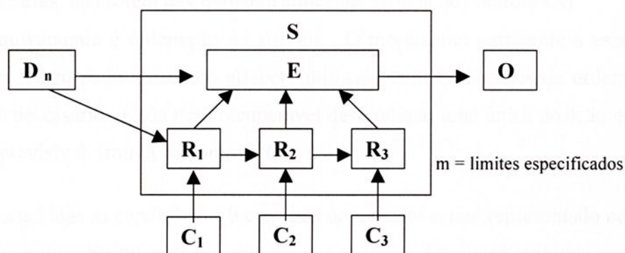
Figura 3: Controle e regulação das características descritivas de um Sistema de CB
