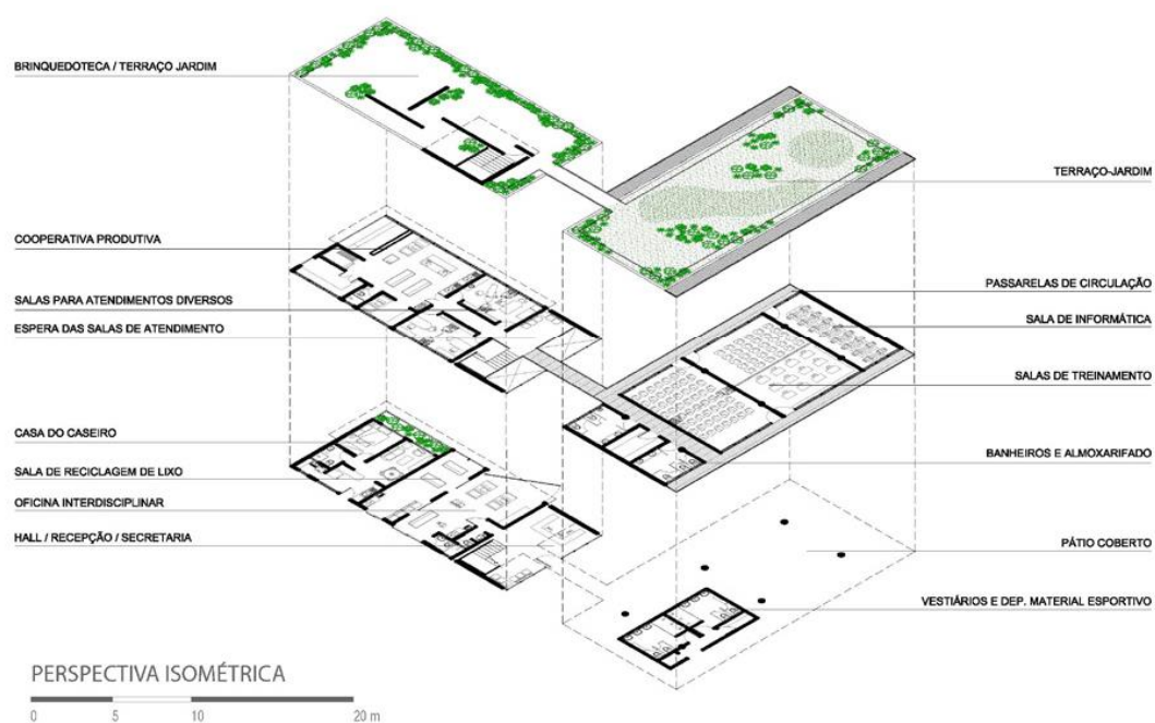
Figura 12: Perspectiva Isométrica Fonte: Rogelio Salmona (ArchDaily)
