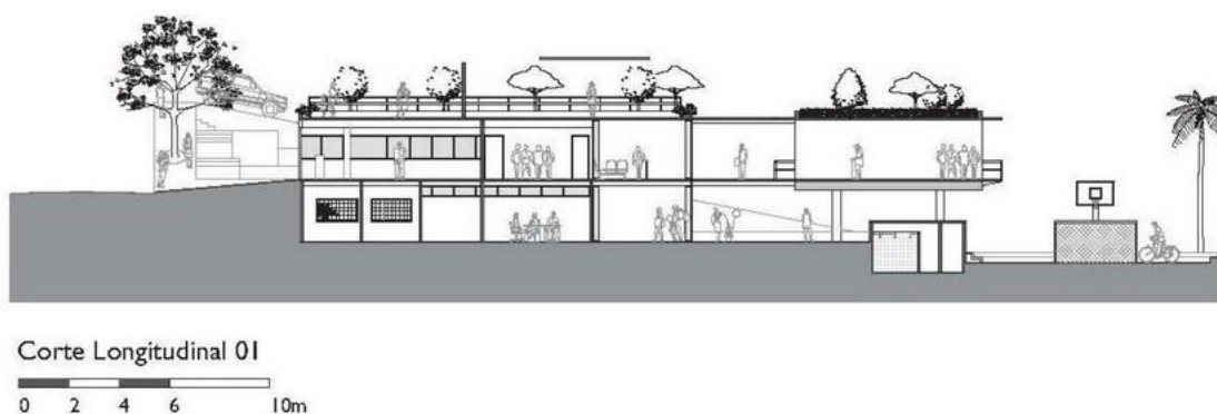
Figura 11: Corte Longitudinal 02. Fonte: Fundação Rogelio Salmona (ArchDaily)
