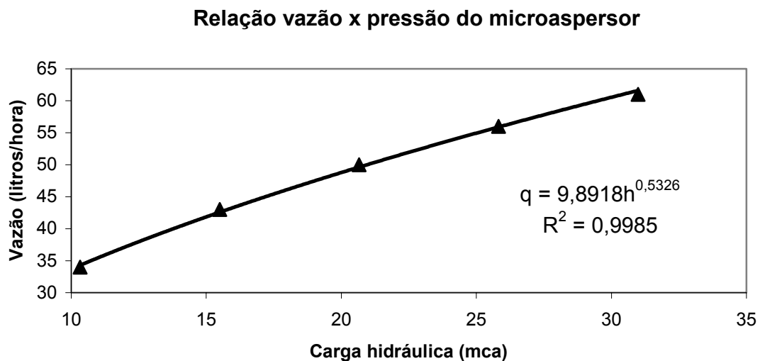
Figura 1. Relação entre vazão e pressão para o microaspersor considerado.
