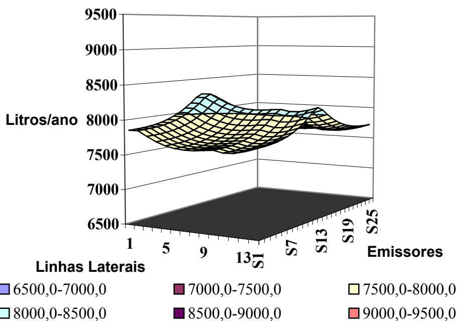
Figura 7. Distribuição da vazão na unidade operacional, com 92% de UE, declividade de 3% e lâmina correspondente a aplicação de um volume de 7,74 m 3 /ano.
