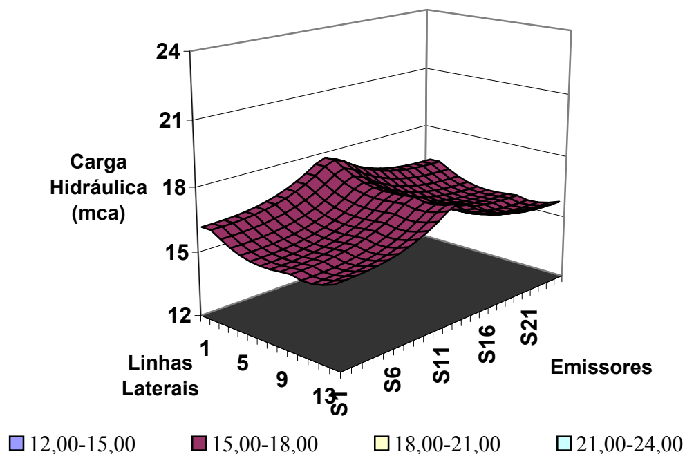
Figura 3. Distribuição da pressão nas linhas laterais da unidade operacional, com 92% de EU calculada e declividade de 3%.
