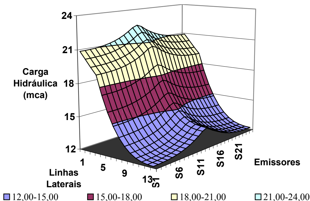
Figura 2. Distribuição da pressão nas linhas laterais da unidade operacional, com 80% de EU calculada e declividade de 0%.
