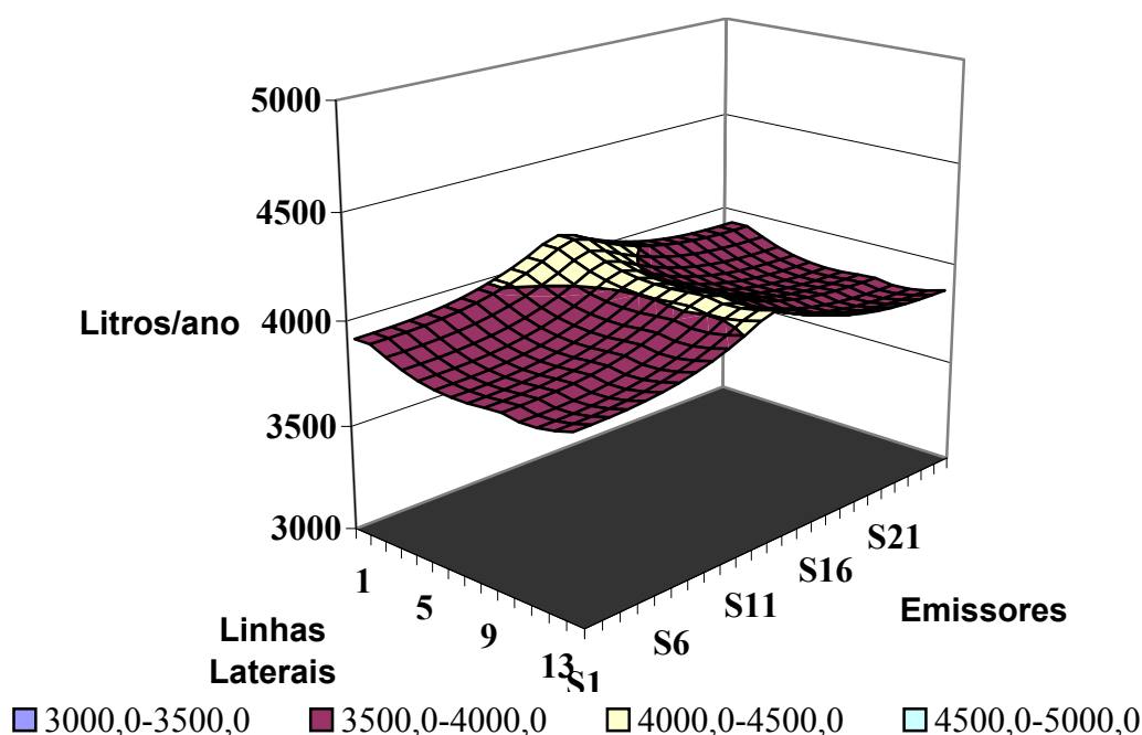
Figura 5. Distribuição da vazão na unidade operacional, com 92% de UE, declividade de 3% e lâmina correspondente a aplicação de um volume de 3,87 \text{ m}^3/\text{ano} .
