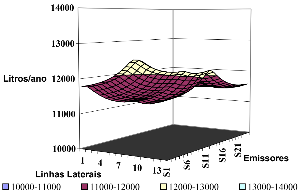
Figura 8. Distribuição da vazão na unidade operacional, com 80% de UE, declividade de 0% e lâmina correspondente a aplicação de um volume de 11,61 \text{ m}^3/\text{ano} .
