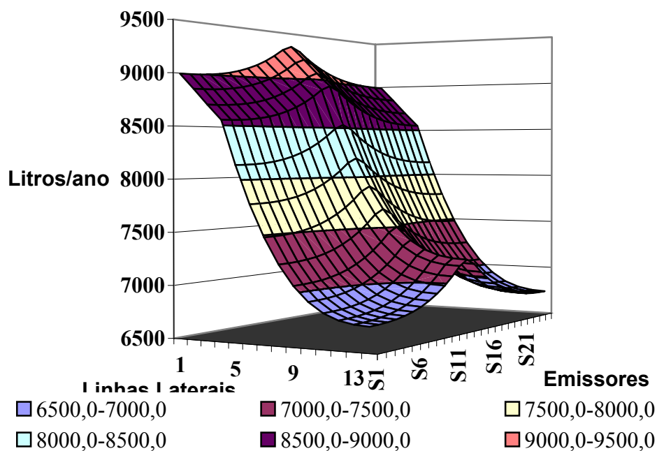
Figura 6. Distribuição da vazão na unidade operacional, com 80% de UE, declividade de 0% e lâmina correspondente a aplicação de um volume de 7,74 m 3 /ano.
