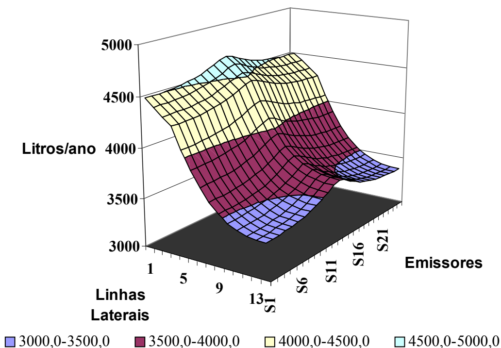
Figura 4. Distribuição da vazão na unidade operacional, com 80% de UE, declividade de 0% e lâmina correspondente a aplicação de um volume de 3,87 \text{ m}^3/\text{ano} .
