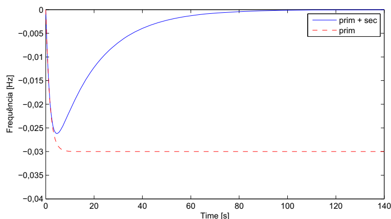
Figura 2.7: Curva de resposta em frequência.
