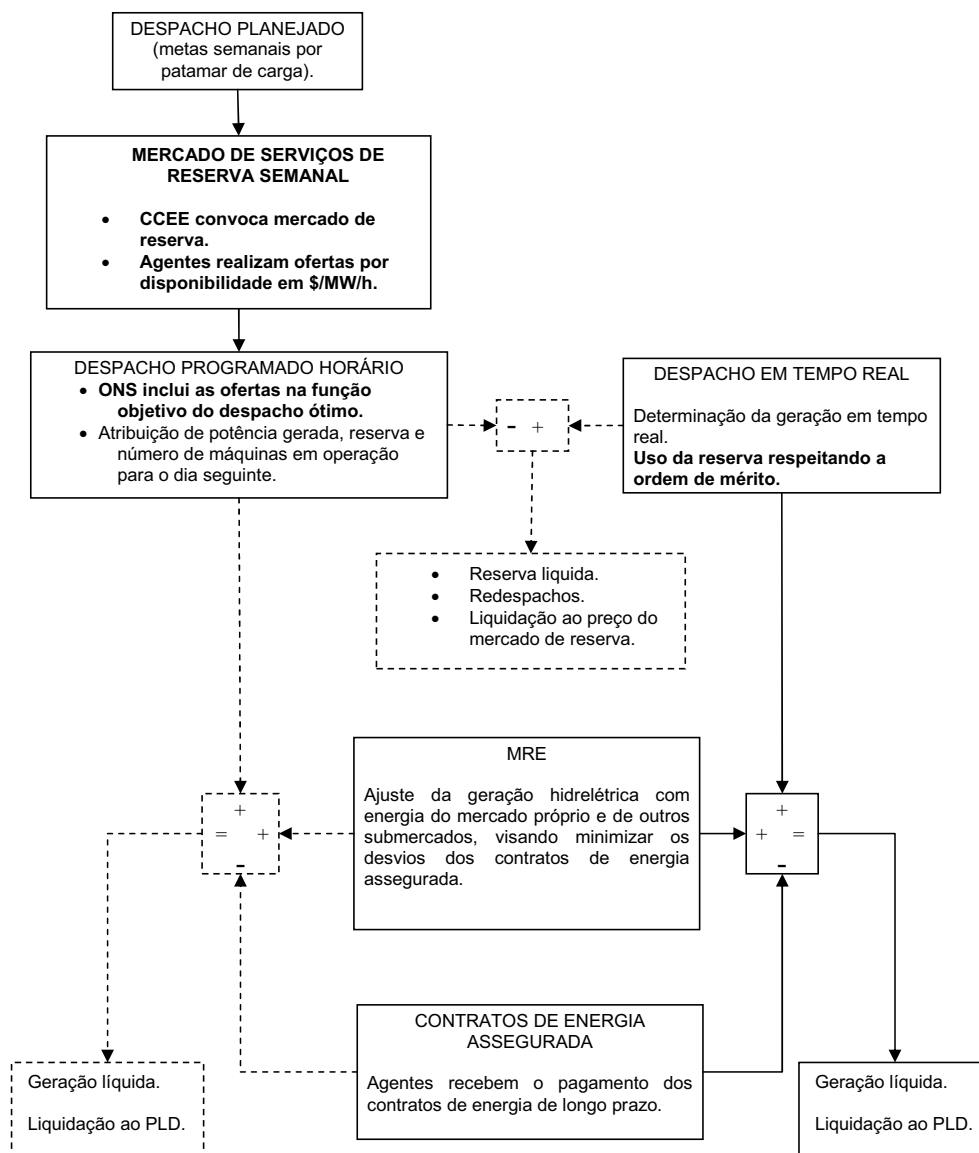
Figura 6.2: Sequência do despacho proposto.
