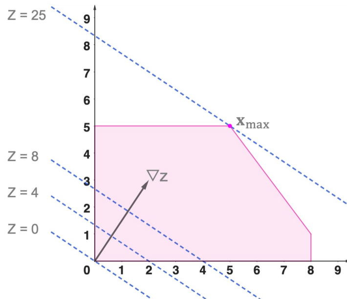
Figura 3 – Solução ótima para o problema - Exemplo 1
