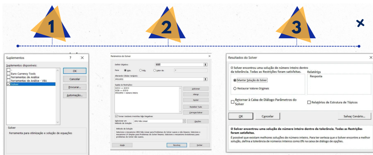
Figura 31 – Slide apresentado por um dos grupos - Solver Excel
