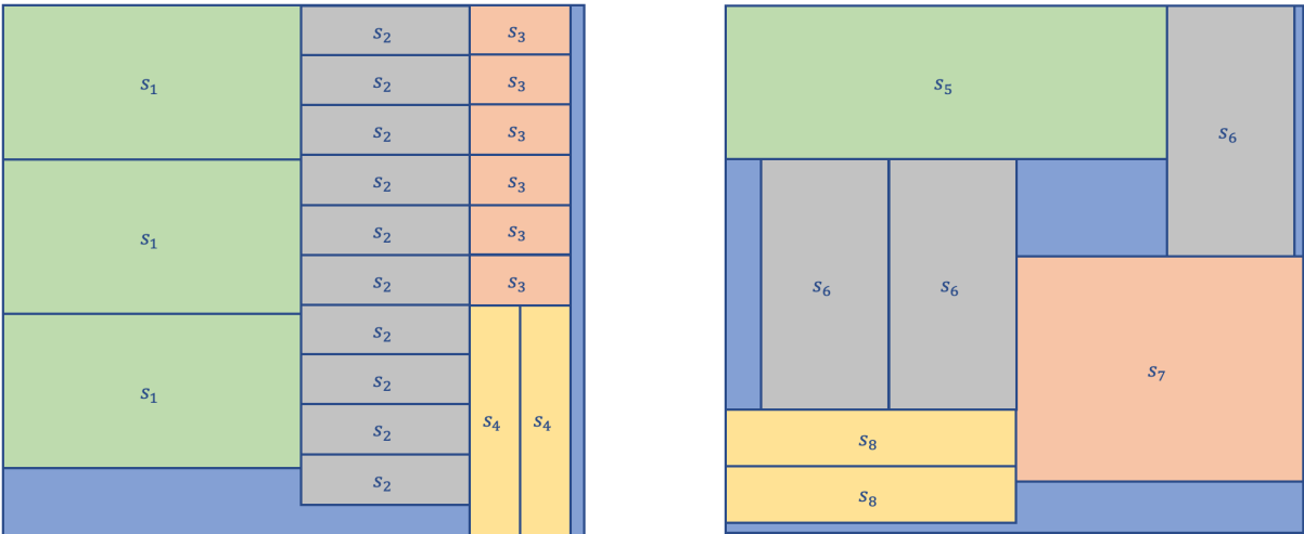
(a) Regular guilhotinado.
