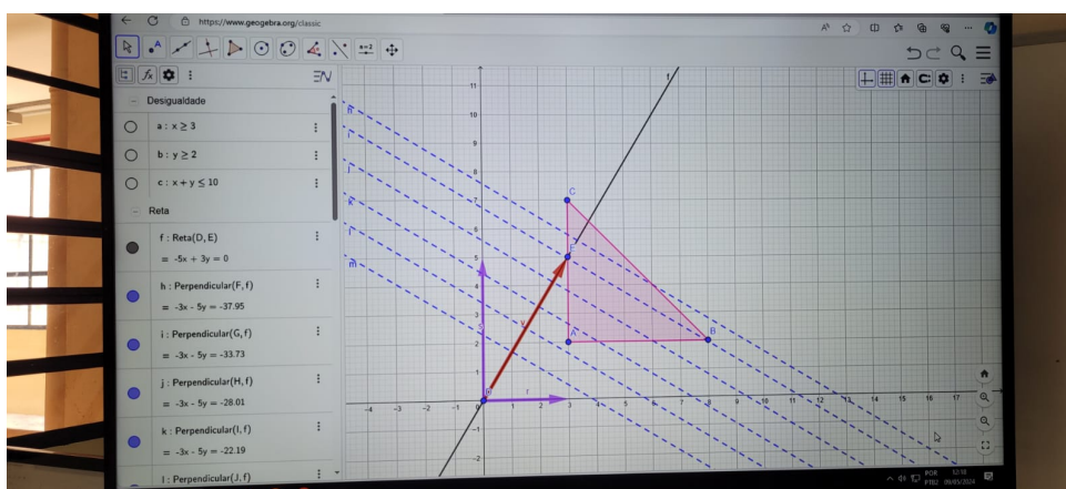
Figura 36 – Discussão Região Factível GeoGebra
