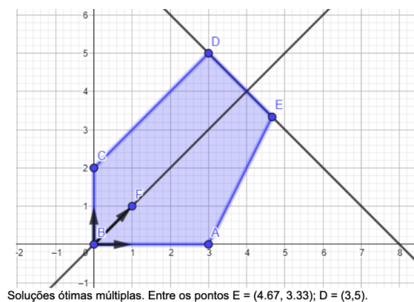
Figura 40 – Atividade realizada por um dos alunos - resolução gráfica soluções múltiplas
