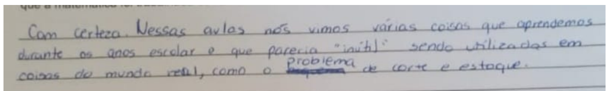
Figura 22 – Resposta do aluno A para a questão 1.
