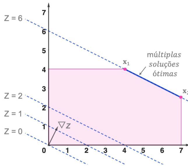
Figura 6 – Múltiplas soluções ótimas para o problema - Exemplo 2.
