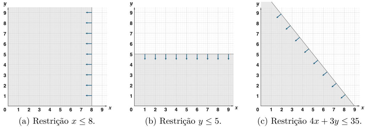
Figura 1 – Passos para a construção da região factível.
