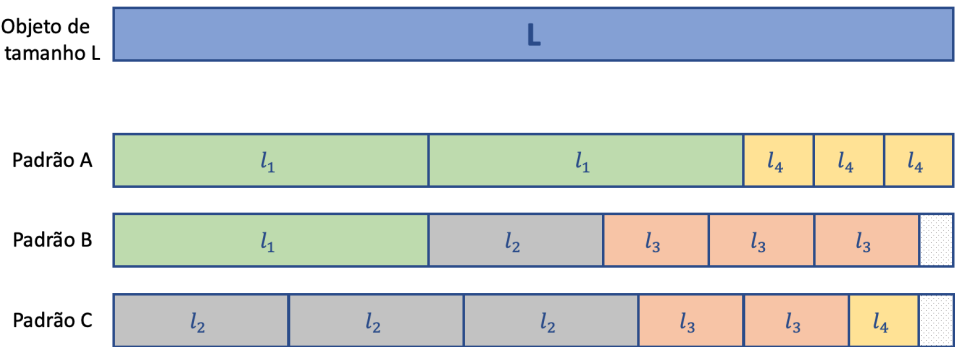
Figura 7 – Padrões de corte unidimensional para um objeto de comprimento L .
