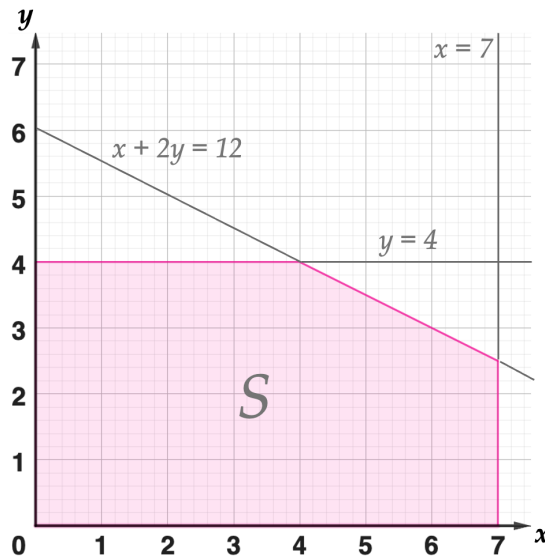
Figura 5 – Região factível para o problema - Exemplo 2.
