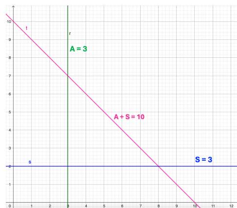
Figura 34 – Construção da região factível do problema do agricultor
