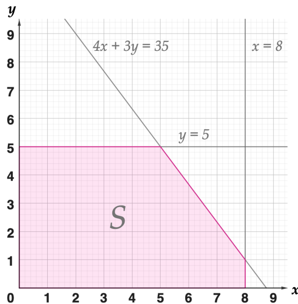
Figura 2 – Região factível do problema - Exemplo 1.
