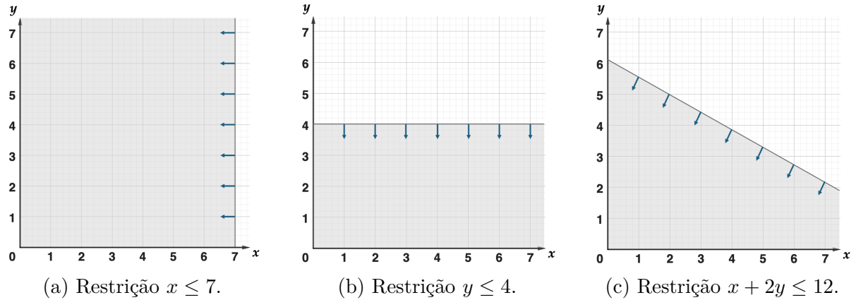
Figura 4 – Passos para a construção da região factível.
