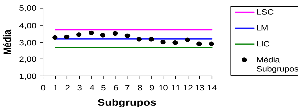
Figura 11.1 – Gráfico da Média e determinação dos limites de controle para o resíduo, atributo cinza. Recálculo.
