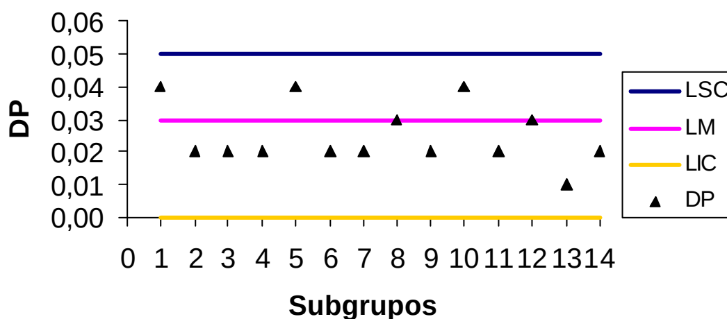
Figura 24.1 – Gráfico do Desvio padrão e determinação dos limites de controle para água, atributo proteína. Recálculo.
