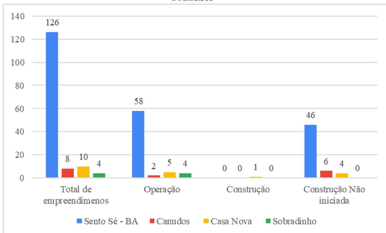
Gráfico 7: Número de Empreendimentos de Energia eólica no Sertão do São Francisco
