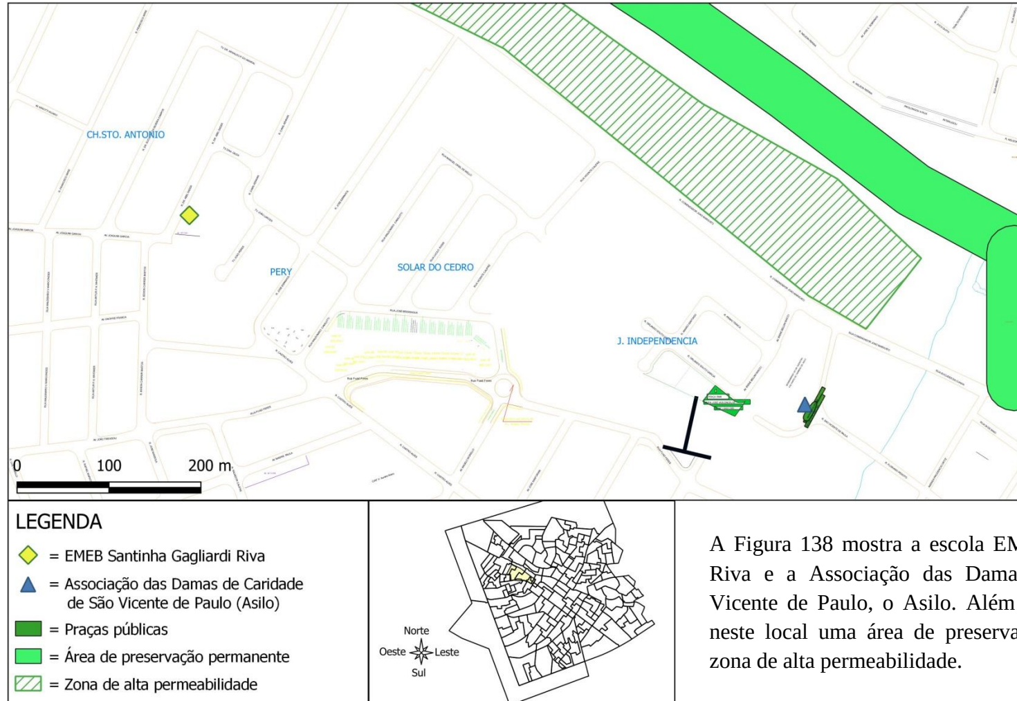
Bairro Alto, Santo Antônio, Pery, Solar do Cedro e Jardim Independência, 2024
