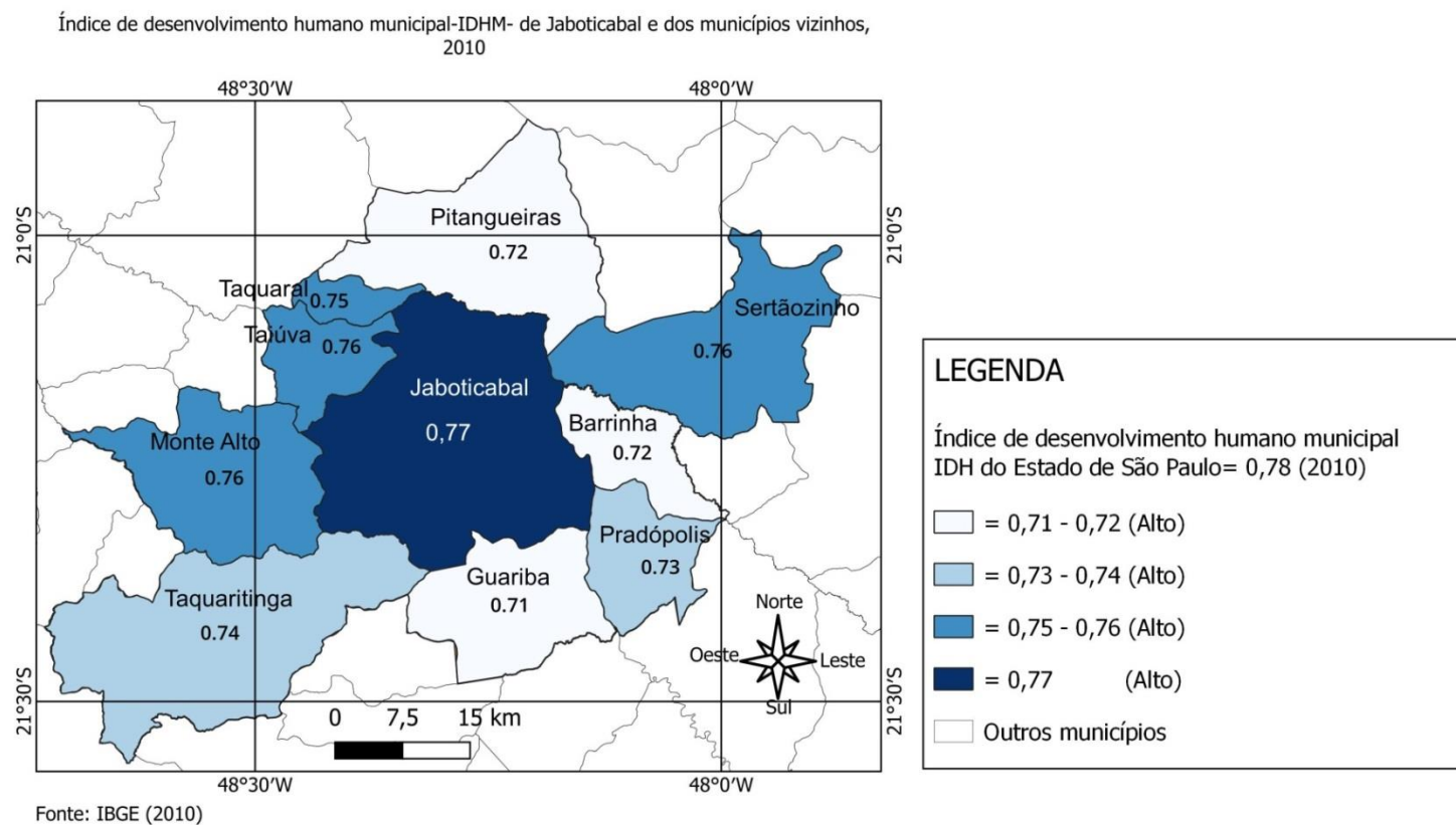
Fig. 96. Índice de desenvolvimento humano municipal –IDHM- de Jaboticabal e nos municípios vizinhos, 2010
