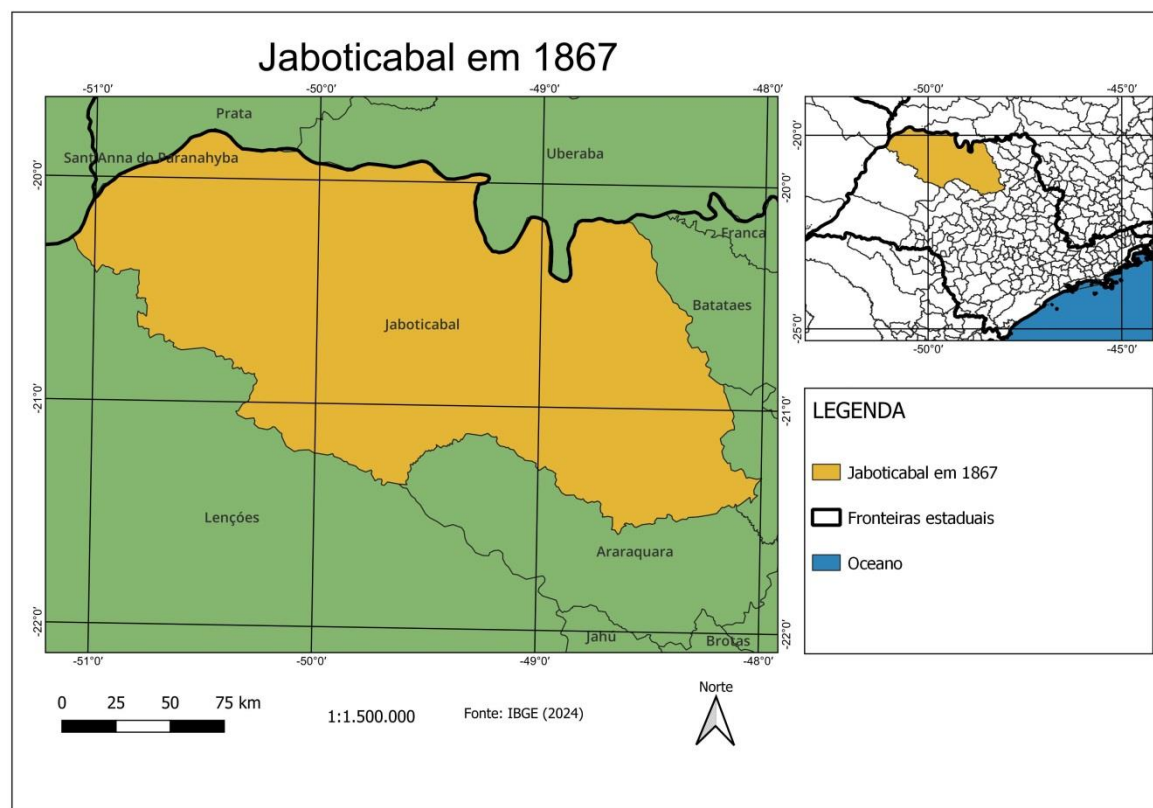
Fig. 66. Evolução do território de Jaboticabal de 1867 a 2010
