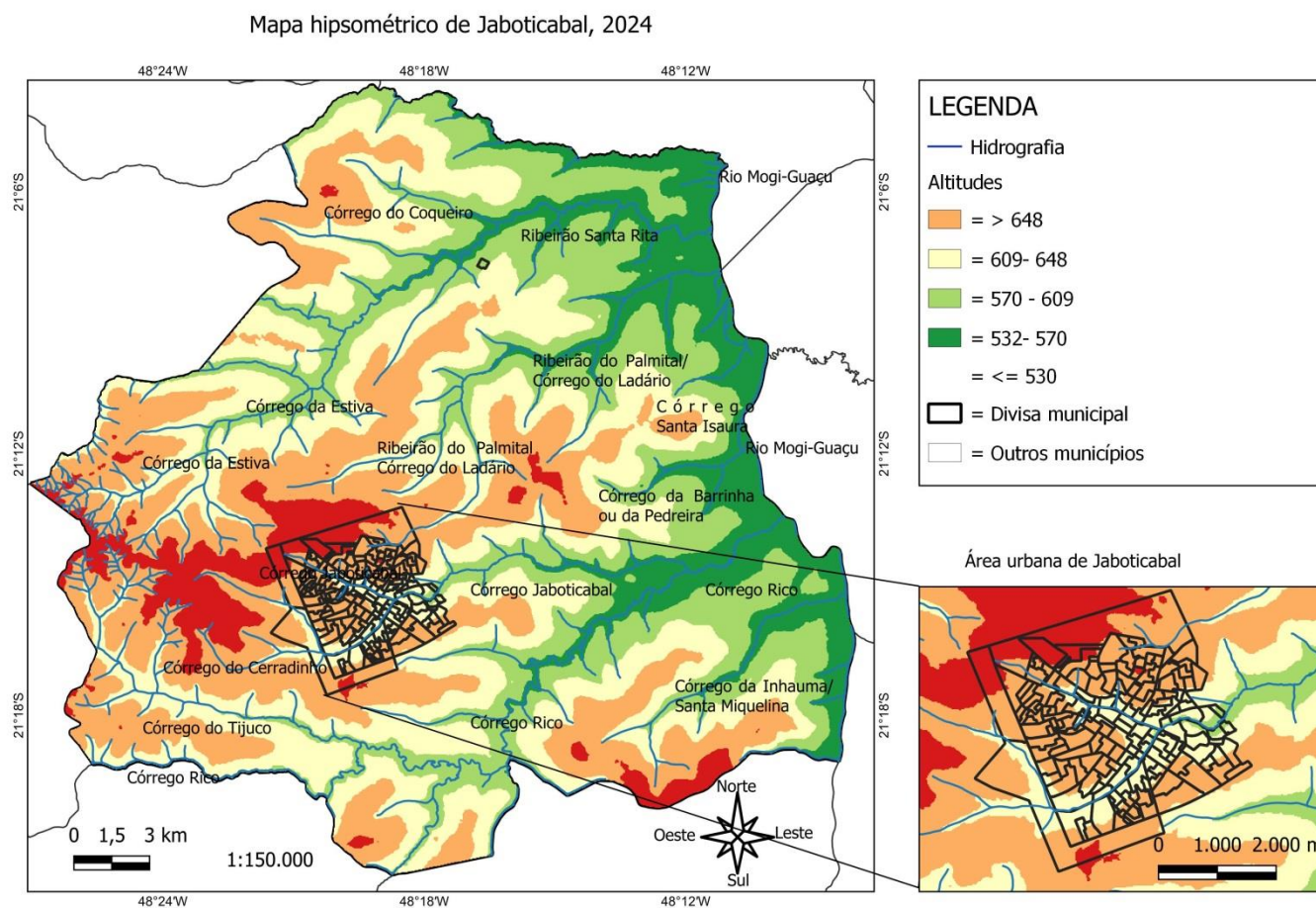
Fig. 7 b. Mapa hipsométrico de Jaboticabal, 2024
