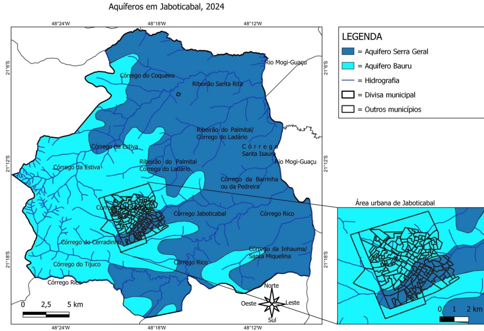
Fig. 118. Aquíferos em Jaboticabal, 2024
