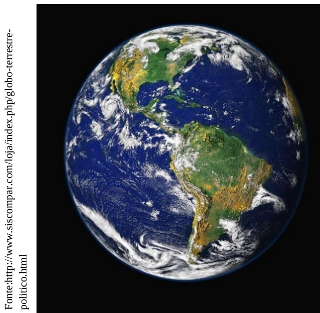
Fig. 11. A Terra vista do espaço
