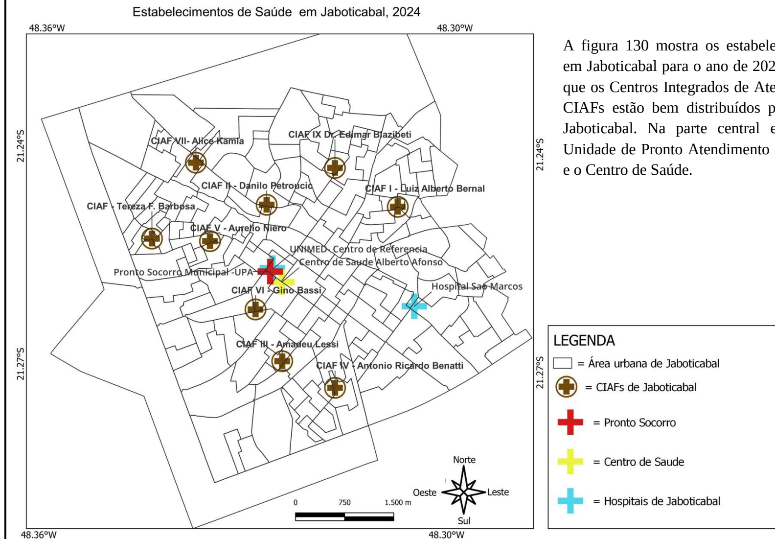
Fig. 130. Estabelecimentos de Saúde em Jaboticabal, 2024
