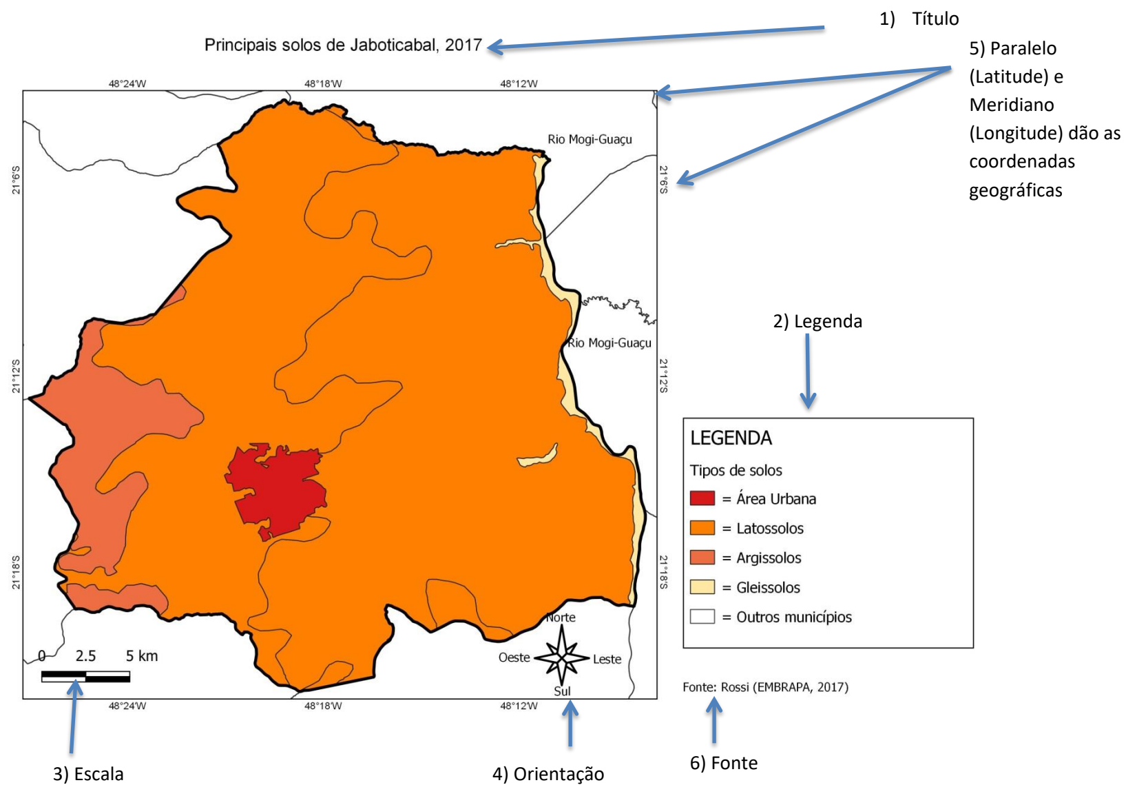
Fig.10. Elementos de um mapa
