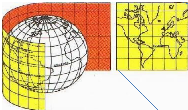
Fig. 13a. O cilindro envolvendo o globo terrestre. A Terra (esférica) transformada em um plano (mapa).
