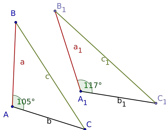
Figura 26 – Explorando LAL
