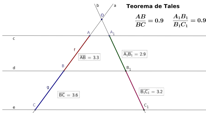
Figura 36 – Explorando homotetia
