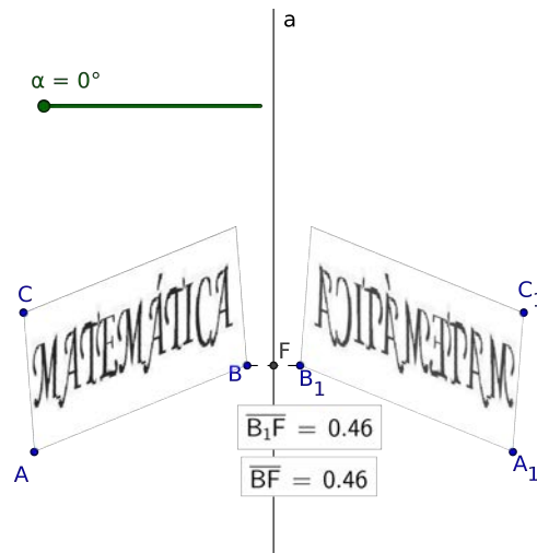
Figura 33 – Explorando rotação
