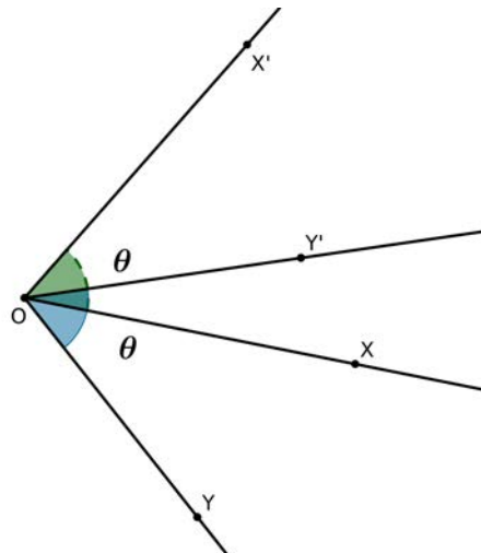
Figura 16 – Rotação de um ângulo \theta
