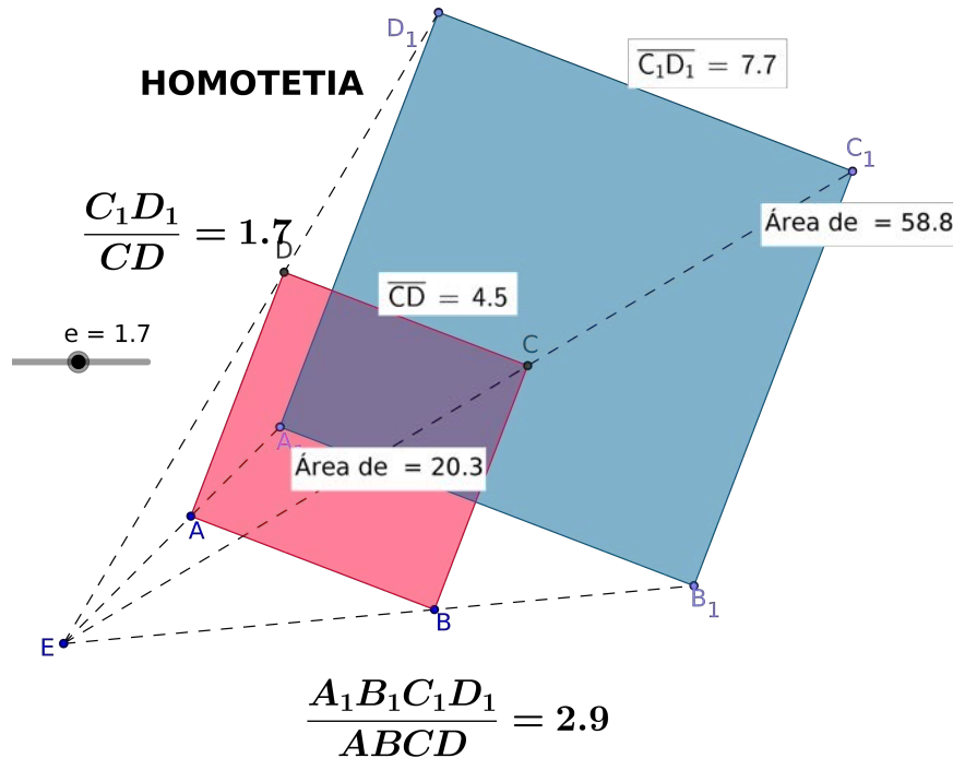
Figura 34 – Explorando homotetia
