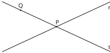
Figura 3.10: Postulado da Existência
