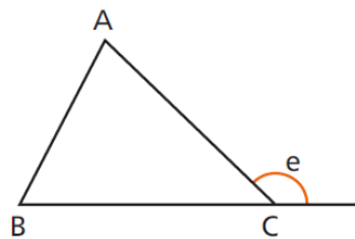
Figura 3.100: Ângulo Externo no Triângulo
