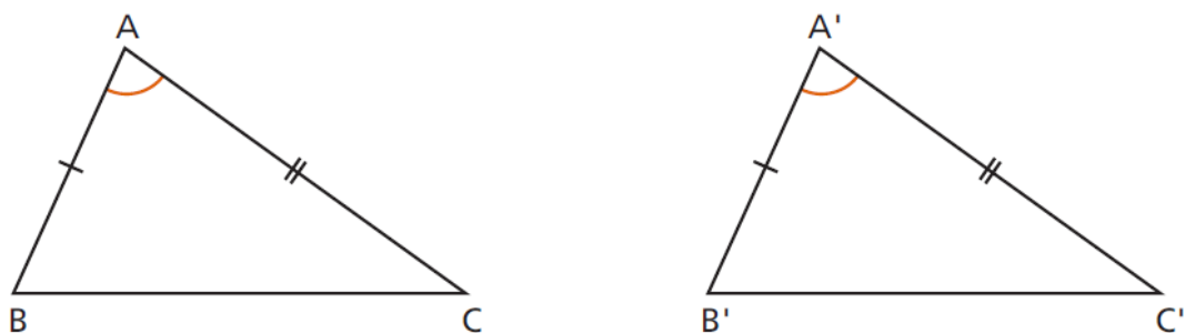
Figura 3.64: Congruência de Triângulos LAL
