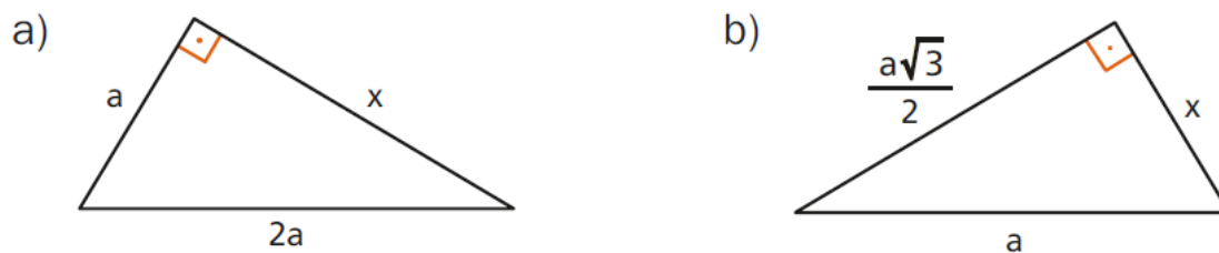
Figura 4.76: Exercício 2 Teorema de Pitágoras
