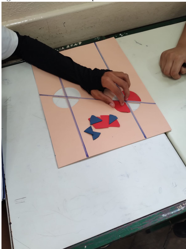
Figura 4.44: Material Manipulativo de Retas Paralelas 1
