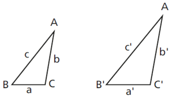
Figura 3.116: Esquema Caso de Semelhança AA
