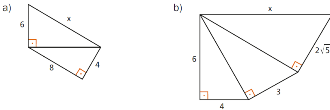
Figura 4.78: Exercício 4 Teorema de Pitágoras
