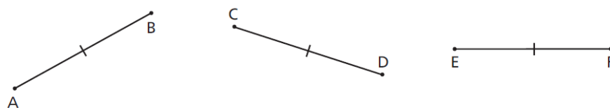
Figura 3.25: Congruência de Segmentos
