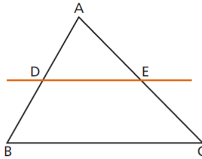
Figura 3.112: Teorema Semelhança de Triângulos - Ângulos Congruentes
