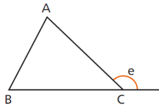
Figura 3.73: Ângulo Externo de um Triângulo
