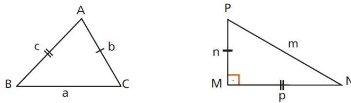
Figura 3.121: Recíproca do Teorema de Pitágoras
