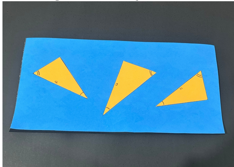
Figura 4.54: Construção caso ALA
