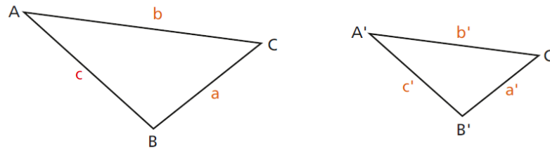
Figura 3.119: Caso de Semelhança LLL - Esquema
