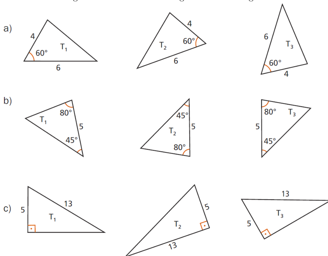
Figura 4.60: Exercício 3 congruência de triângulos
