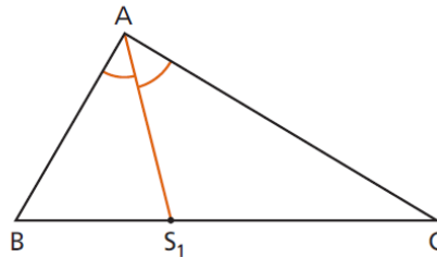
Figura 3.72: Bissetriz Interna de um Triângulo
