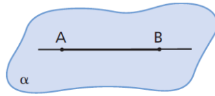
Figura 3.34: Região Convexa - Plano
