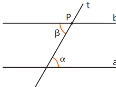
Figura 3.97: Unicidade das Paralelas
