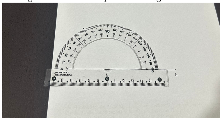
Figura 4.18: Construção de um ângulo de 120^\circ
