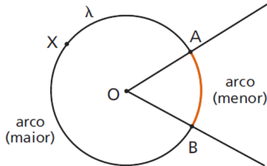
Figura 3.124: Arco de Circunferência
