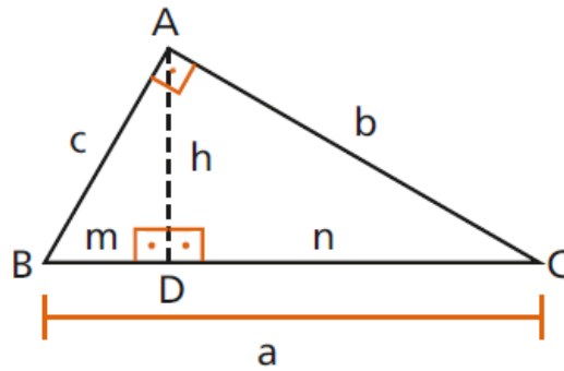
Figura 3.120: Teorema de Pitágoras
