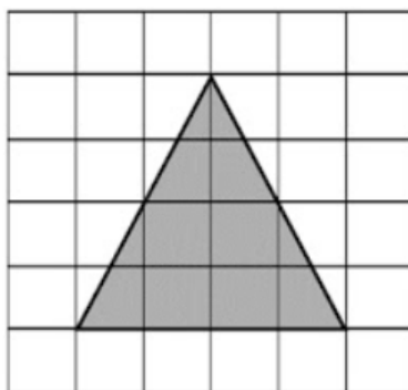
Figura 4.29: Exercício 5 ampliação redução
