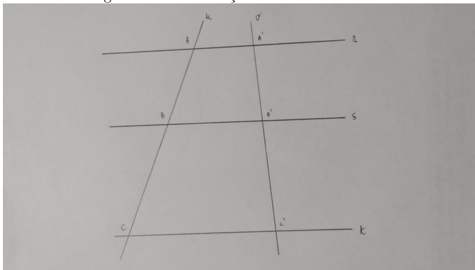
Figura 4.63: Construção do Teorema de Tales
