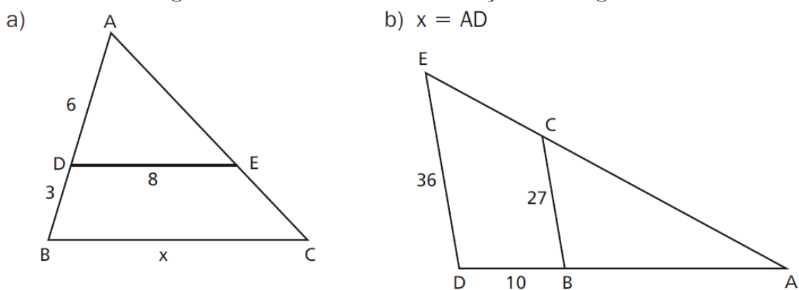
Figura 4.72: Exercício 4 Semelhança de Triângulos
