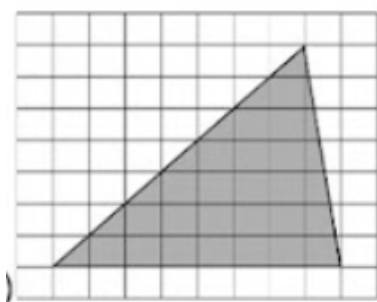
Figura 4.33: Exercício 5d ampliação redução
