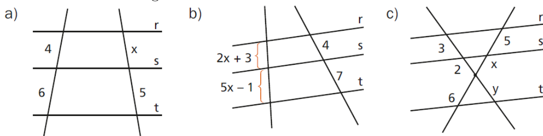
Figura 4.65: Exercício 2 teorema de tales
