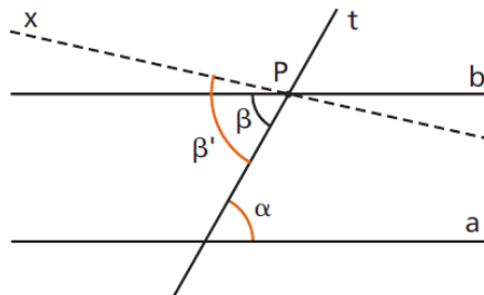
Figura 3.98: Unicidade das Paralelas 1
