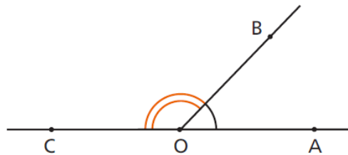
Figura 3.52: Ângulo Suplementar Adjacente
