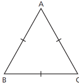
Figura 3.78: Exemplo Triângulo Equilátero
