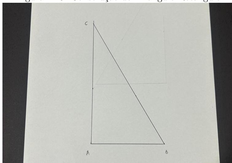
Figura 4.16: Construção do Triângulo Retângulo
