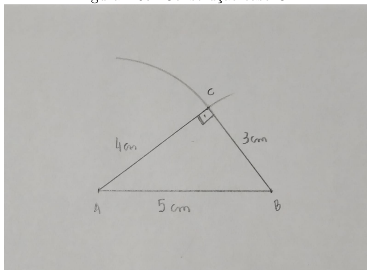
Figura 4.57: Construção caso CH
