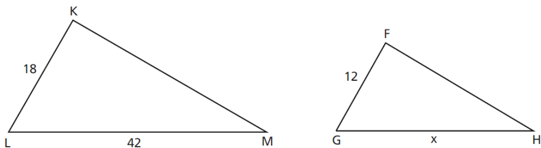
Figura 4.71: Exercício 3 Semelhança de Triângulos
