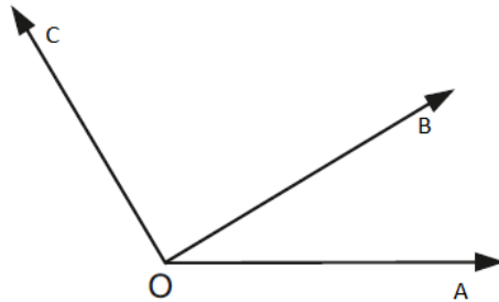
Figura 3.47: Adição de Ângulos
