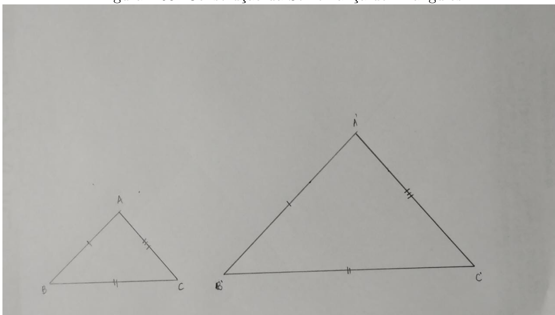
Figura 4.68: Construção da Semelhança de Triângulos
