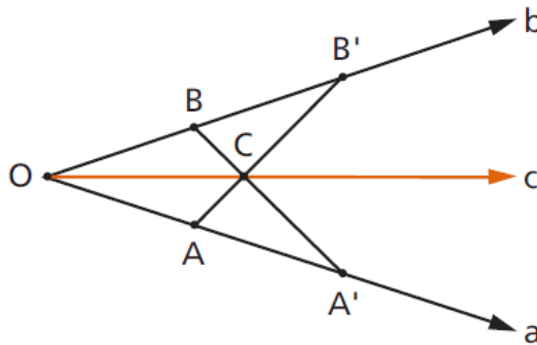
Figura 3.70: Existência do Bissetriz
