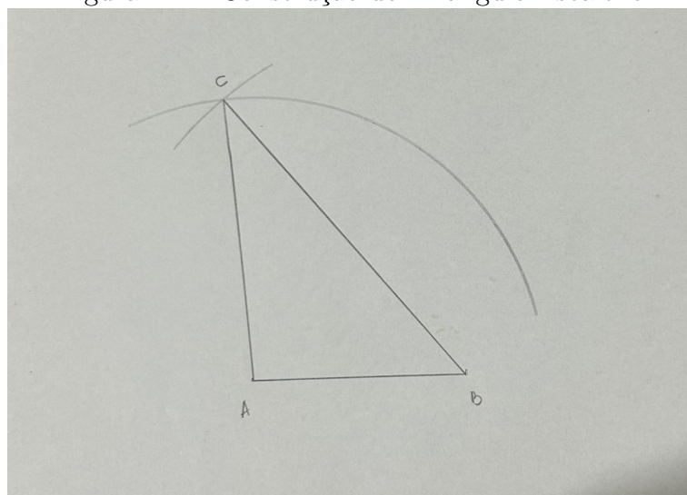
Figura 4.12: Construção do Triângulo Escaleno
