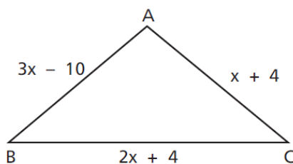
Figura 3.79: Exemplo Triângulo Isósceles
