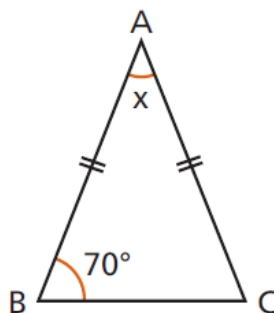
Figura 4.40: Exercício 3a soma dos ângulos internos do triângulo
