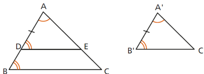
Figura 3.115: Caso de Semelhança AA
