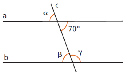
Figura 4.50: Exercício 3 ângulos formados por retas paralelas
