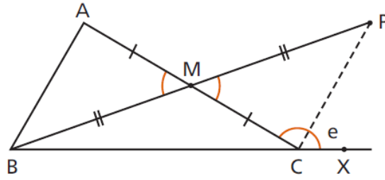
Figura 3.74: Demonstração Ângulo Externo
