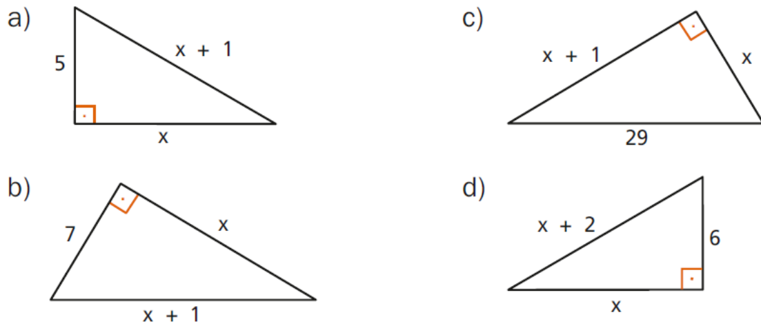
Figura 4.77: Exercício 3 Teorema de Pitágoras
