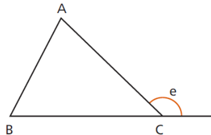
Figura 3.102: Soma dos Ângulos Internos do Triângulo
