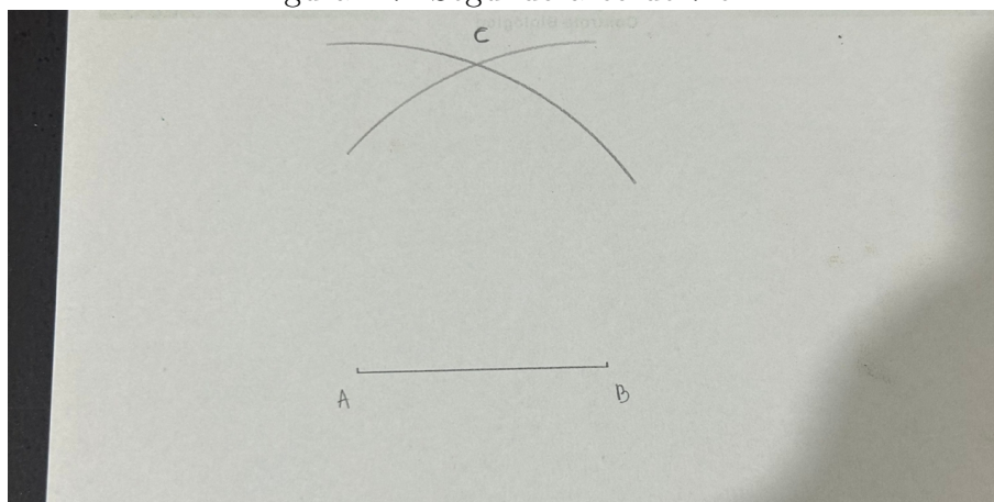
Figura 4.7: Segundo arco de 7 cm
