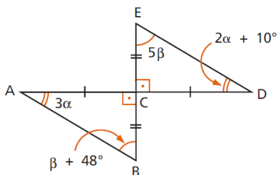
Figura 4.61: Exercício 4 congruência de triângulos
