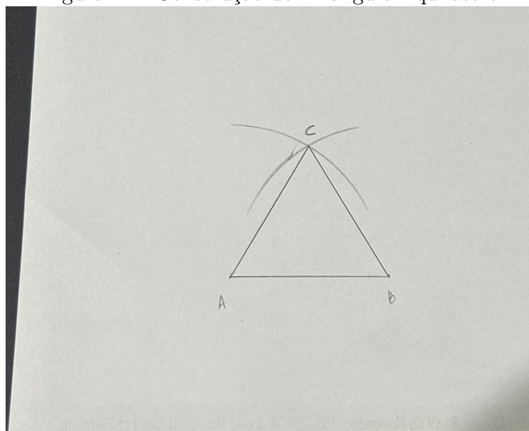
Figura 4.4: Construção do Triângulo Equilátero
