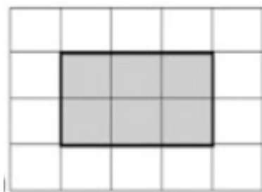
Figura 4.25: Exercício 2c ampliação redução
