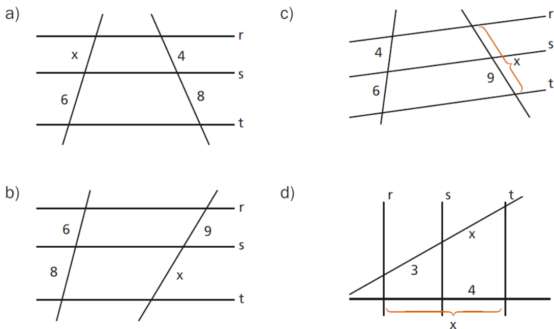
Figura 4.64: Exercício 1 teorema de tales
