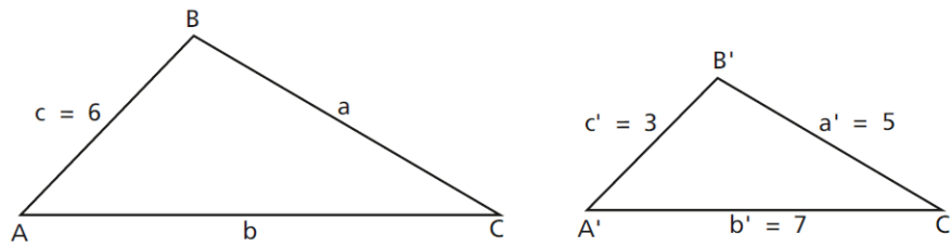
Figura 3.111: Exemplo Semelhança de Triângulos
