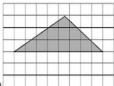
Figura 4.31: Exercício 5b ampliação redução
