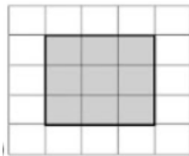
Figura 4.24: Exercício 2b ampliação redução
