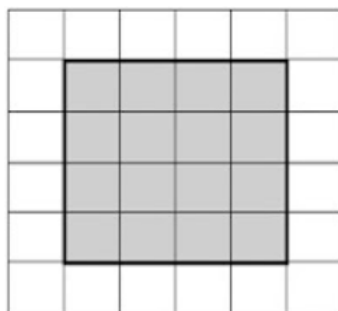
Figura 4.22: Exercício 2 ampliação redução
