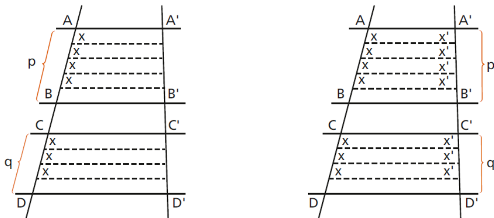
Figura 3.108: Demonstração do Teorema de Tales - Parte 1
