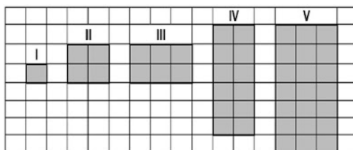
Figura 4.21: Exercício 1 ampliação redução
