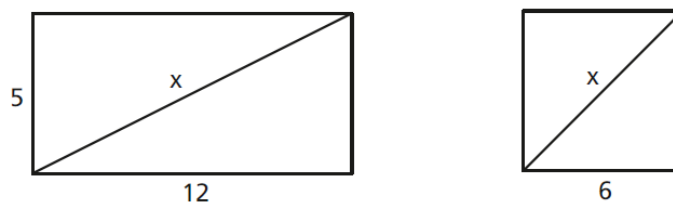
Figura 4.79: Exercício 5 Teorema de Pitágoras a) retângulo b) quadrado
