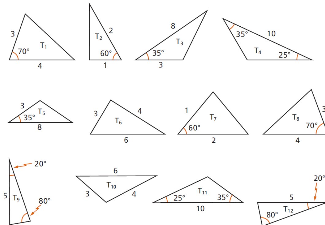
Figura 4.58: Exercício 1 congruência de triângulos
