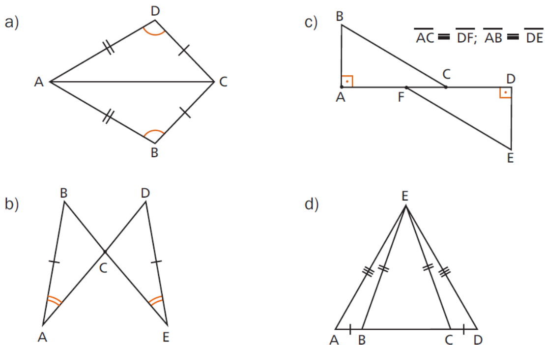
Figura 4.62: Exercício 5 congruência de triângulos
