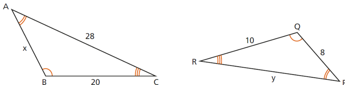
Figura 4.70: Exercício 2 Semelhança de Triângulos
