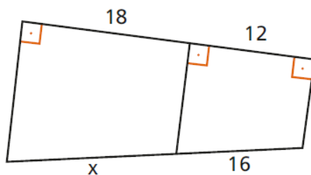
Figura 4.66: Exercício 3 teorema de tales
