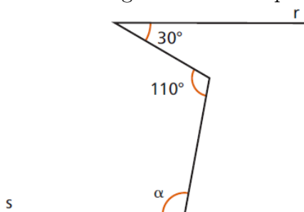
Figura 4.52: Exercício 5 ângulos formados por retas paralelas
