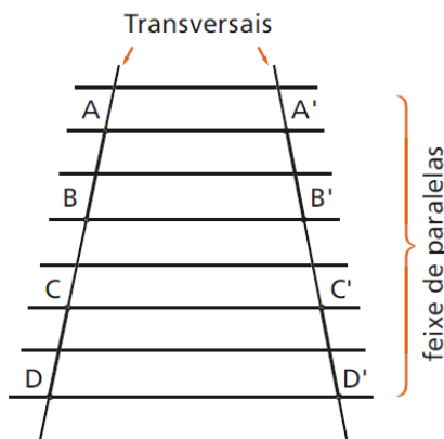
Figura 3.105: Teorema de Tales
