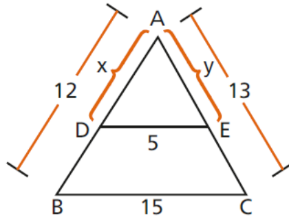
Figura 3.114: Exemplo 3.45 Teorema Fundamental da Semelhança
