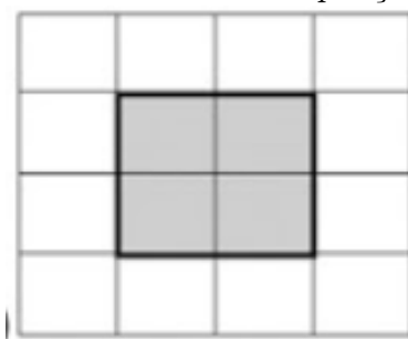
Figura 4.23: Exercício 2a ampliação redução
