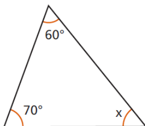
Figura 4.36: Exercício 1a soma dos ângulos internos do triângulo
