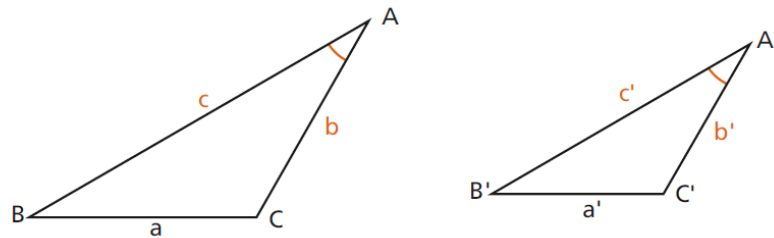
Figura 3.118: Caso de Semelhança LAL - Esquema
