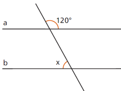
Figura 4.47: Exercício 1b ângulos formados por retas paralelas
