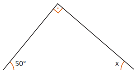
Figura 4.37: Exercício 1b soma dos ângulos internos do triângulo
