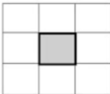
Figura 4.26: Exercício 2d ampliação redução
