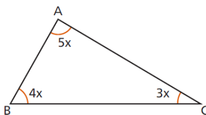
Figura 4.43: Exercício 4 soma dos ângulos internos do triângulo
