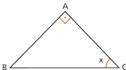
Figura 4.42: Exercício 3c soma dos ângulos internos do triângulo
