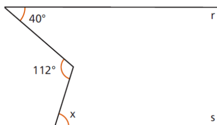
Figura 4.51: Exercício 4 ângulos formados por retas paralelas
