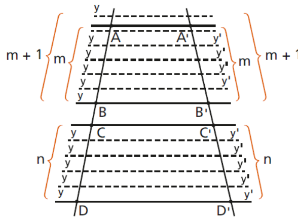
Figura 3.109: Demonstração do Teorema de Tales - Parte 2
