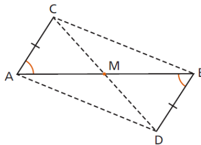
Figura 3.69: Existência do Ponto Médio
