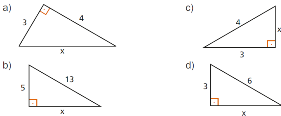
Figura 4.75: Exercício 1 Teorema de Pitágoras
