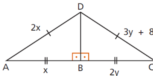
Figura 4.59: Exercício 2 congruência de triângulos
