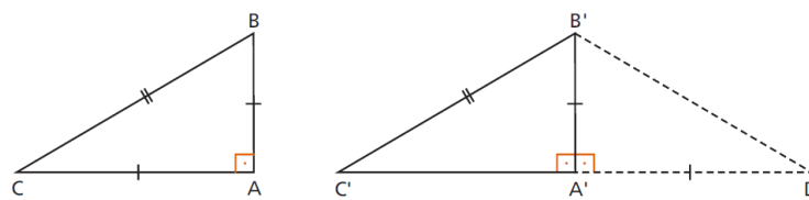
Figura 3.76: Congruência no Triângulo Retângulo
