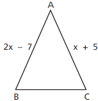
Figura 3.77: Exemplo Triângulo Isósceles
