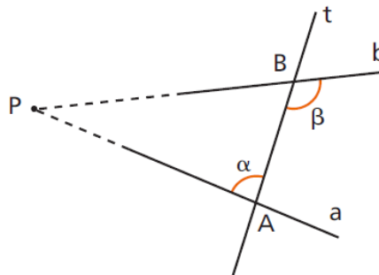
Figura 3.96: Existência da Paralela Triângulo ABP 2
