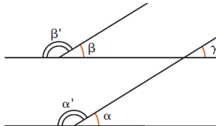
Figura 3.103: Ângulos de Lados Paralelos
