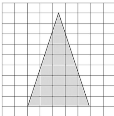
Figura 4.28: Exercício 4 ampliação redução
