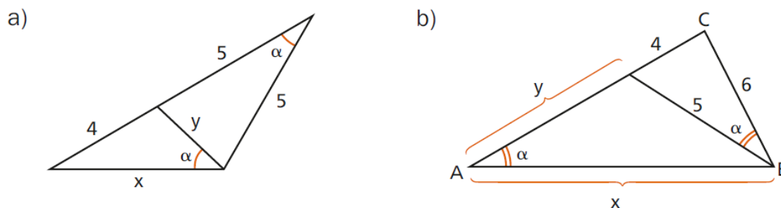
Figura 4.73: Exercício 5 Semelhança de Triângulos
