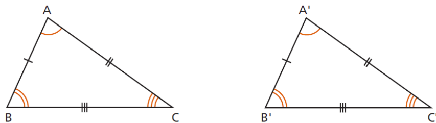
Figura 3.63: Congruência de Triângulos
