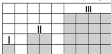
Figura 4.27: Exercício 3 ampliação redução
