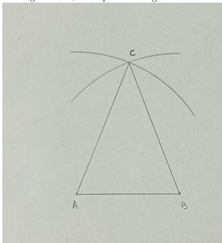
Figura 4.8: Construção do Triângulo Isósceles
