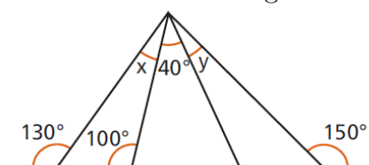
Figura 4.39: Exercício 2b soma dos ângulos internos do triângulo
