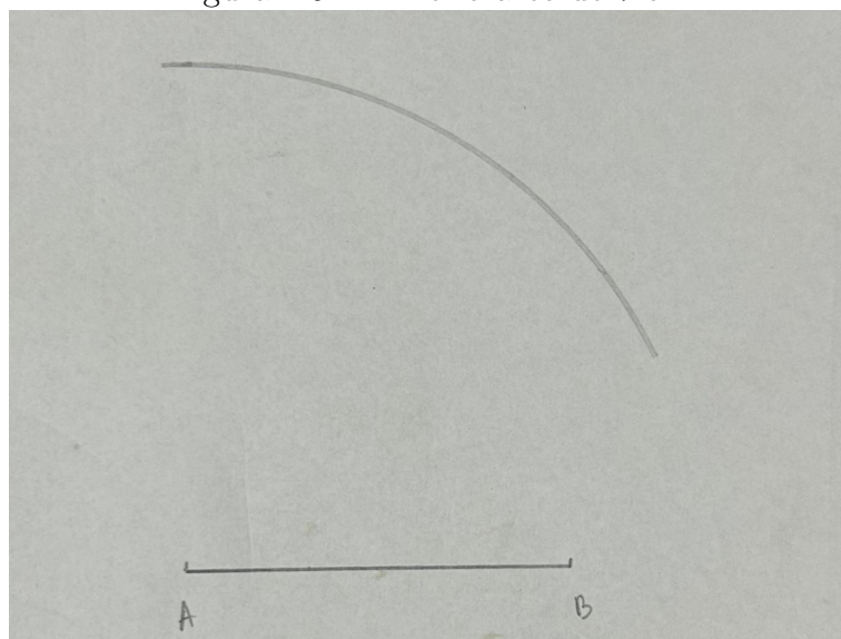
Figura 4.6: Primeiro arco de 7 cm
