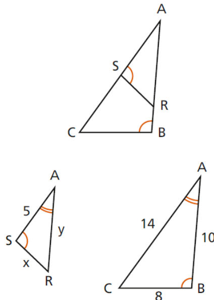
Figura 3.117: Exemplo 3.46 Caso de Semelhança AA
