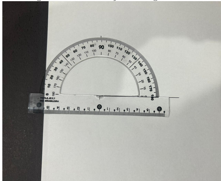
Figura 4.14: Construção do Ângulo de 90^\circ
