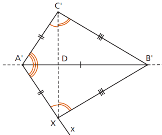
Figura 3.68: Demonstração Congruência de Triângulos LLL
