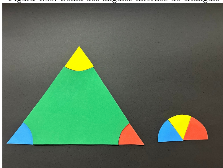
Figura 4.35: Soma dos ângulos internos do triângulo
