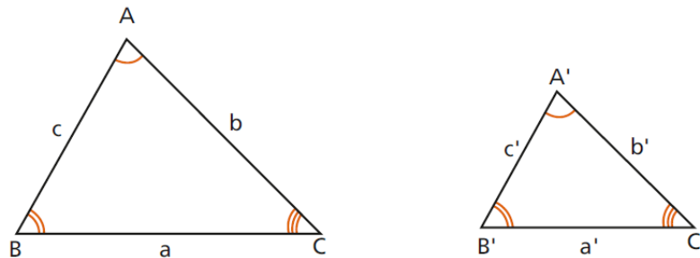
Figura 3.110: Semelhança de Triângulos
