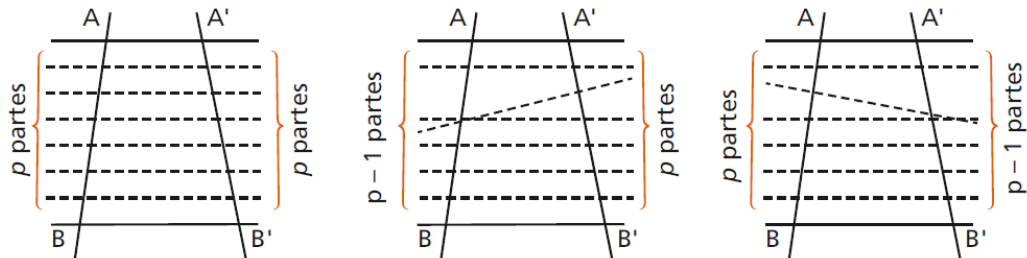
Figura 3.106: Demonstração da Propriedade 3.39 - Parte 1
