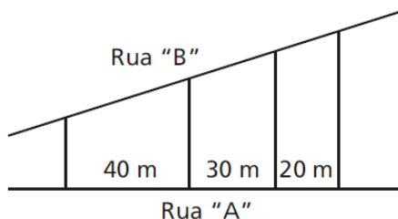
Figura 4.67: Exercício 4 teorema de Tales
