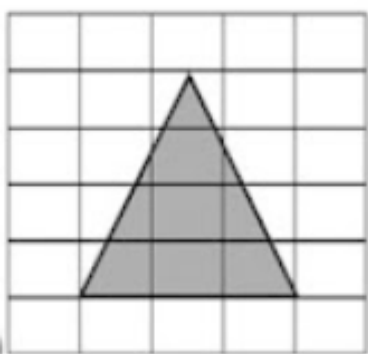
Figura 4.30: Exercício 5a ampliação redução
