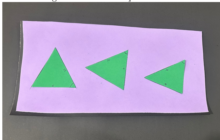
Figura 4.56: Construção caso LAL
