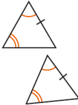
Figura 3.85: Exemplo Triângulo Congruência 6
