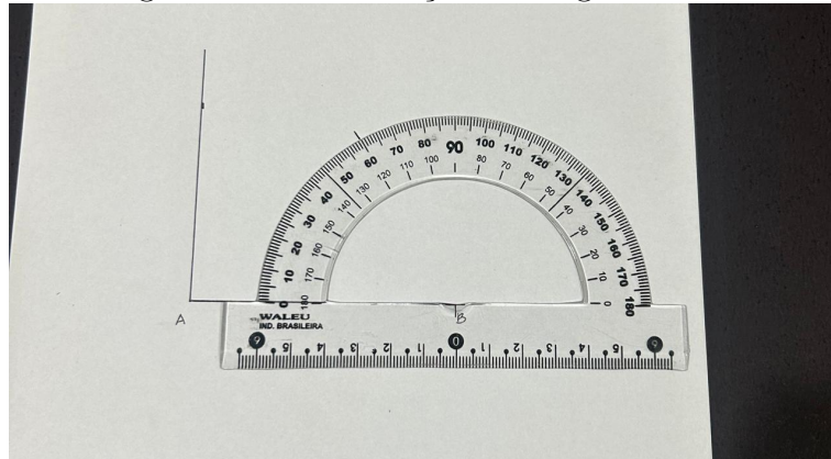
Figura 4.15: Construção do Ângulo de 60^\circ
