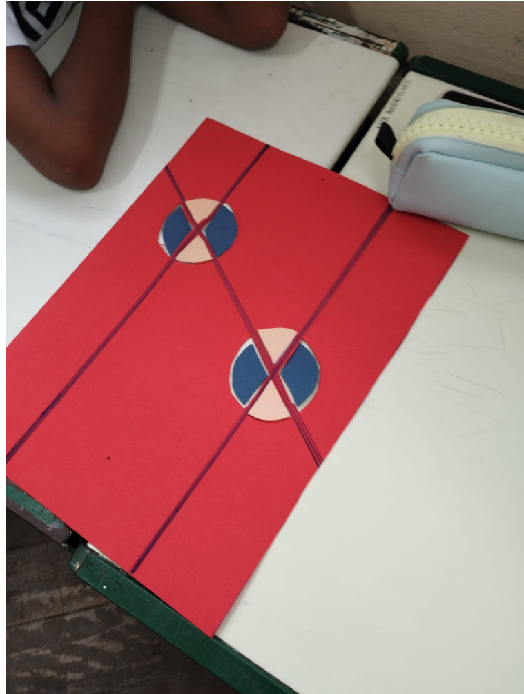
Figura 4.45: Material Manipulativo de Retas Paralelas 2
