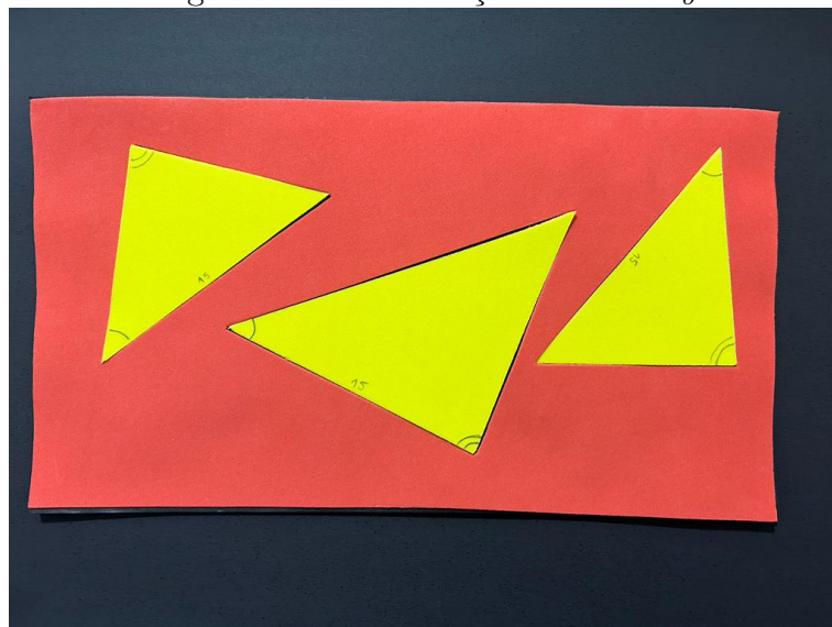
Figura 4.55: Construção caso LAA_o
