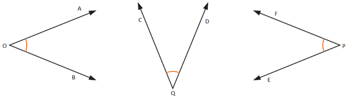
Figura 3.44: Congruência entre ângulos
