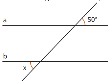
Figura 4.46: Exercício 1a ângulos formados por retas paralelas
