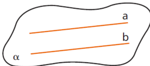
Figura 3.91: Retas Paralelas Distintas
