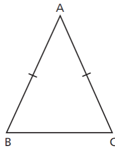
Figura 3.65: Congruência de Triângulos Isósceles
