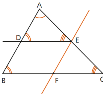
Figura 3.113: Teorema Semelhança de Triângulos - Lados Proporcionais
