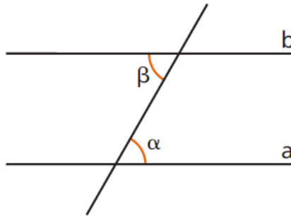
Figura 3.99: Ângulos formados por duas Retas Paralelas e uma transversal
