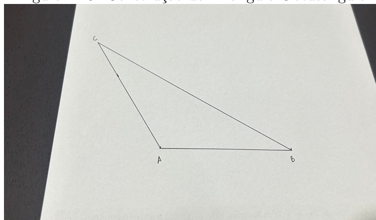
Figura 4.19: Construção do Triângulo Obtusângulo
