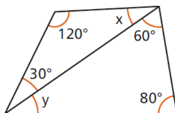
Figura 4.38: Exercício 2a soma dos ângulos internos do triângulo
