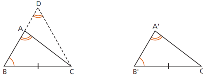
Figura 3.75: Congruência Lado, Ângulo e Ângulo Oposto
