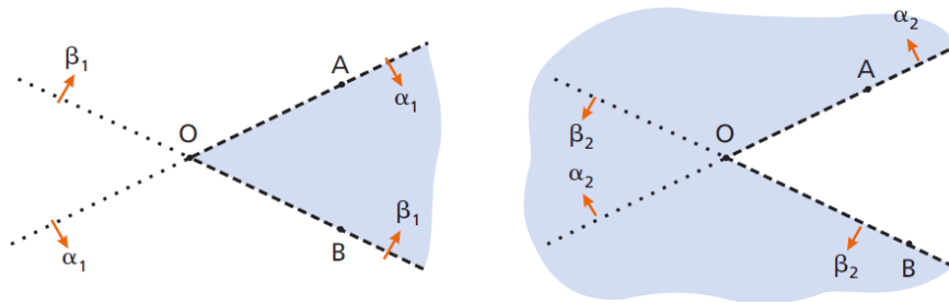
Figura 3.40: Interior e Exterior do Ângulo
