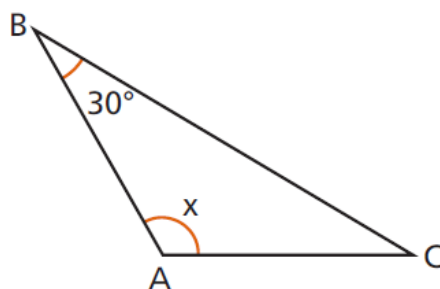
Figura 4.41: Exercício 3b soma dos ângulos internos do triângulo
