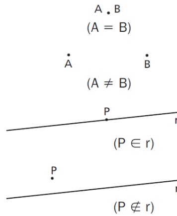
Figura 3.5: Retas e Pontos
