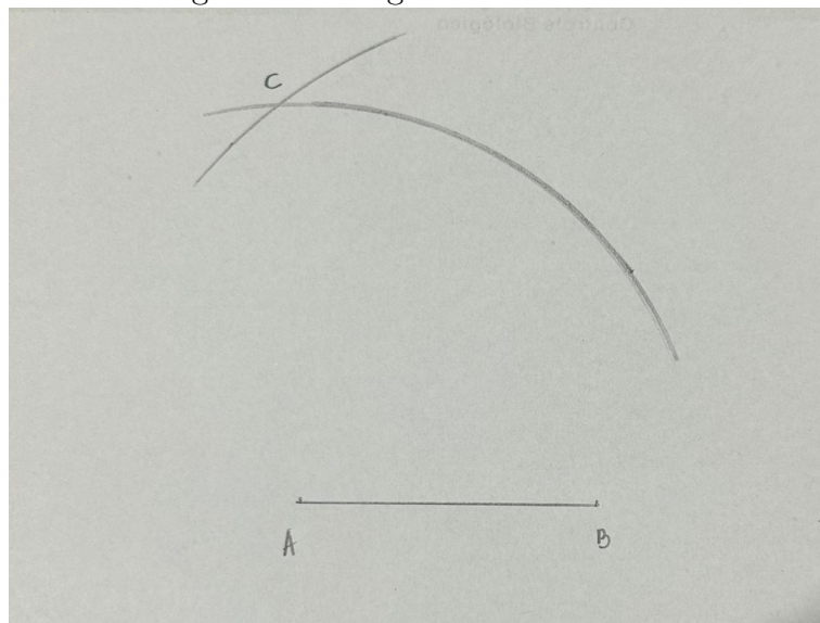
Figura 4.11: Segundo arco de 9 cm
