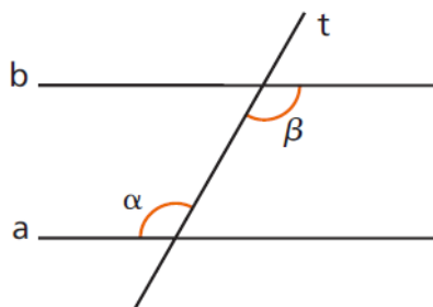
Figura 3.94: Existência da Paralela
