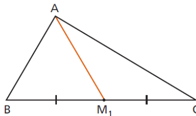
Figura 3.71: Mediana de um Triângulo
