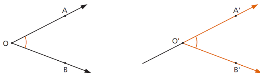
Figura 3.45: Transporte de Ângulos
