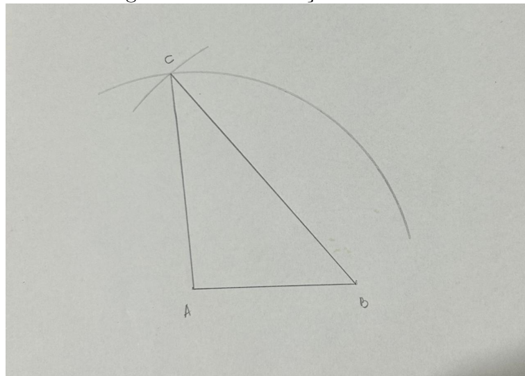
Figura 4.53: Construção caso LLL
