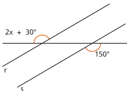
Figura 4.48: Exercício 2a ângulos formados por retas paralelas
