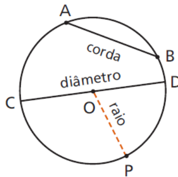
Figura 3.123: Elementos da Circunferência
