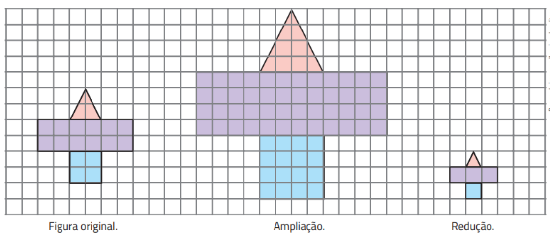
Figura 4.20: Ampliação e Redução de Figuras
