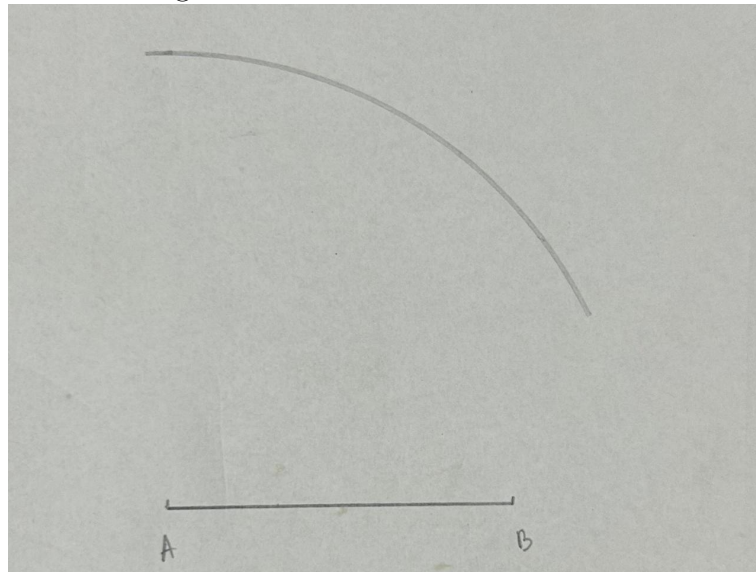
Figura 4.10: Primeiro arco de 7 cm
