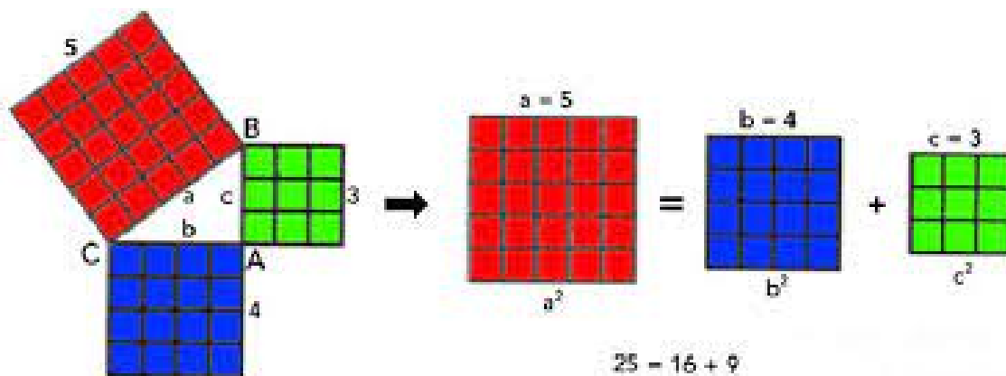
Figura 4.74: Construção do Teorema de Pitágoras
