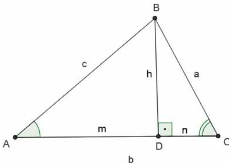
Figura 31: Triângulo ABC com altura \overline{BD} .
