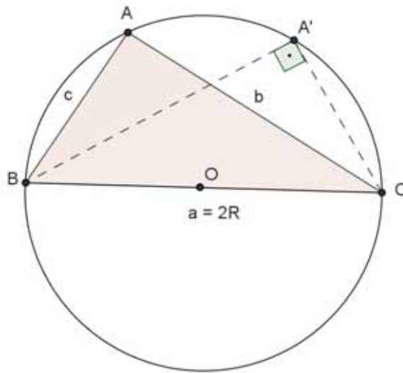
Figura 30: Triângulo ABC retângulo.
