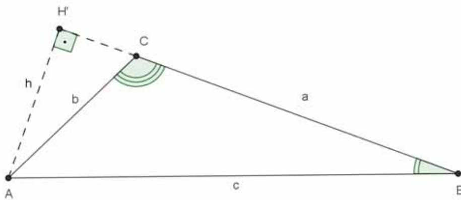
Figura 26: Triângulo ABC obtusângulo em C e com altura \overline{AH} .
