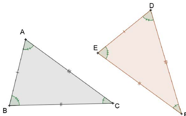
Figura 12: Triângulos congruentes. Extraído de COSTA (2012, p. 15)
