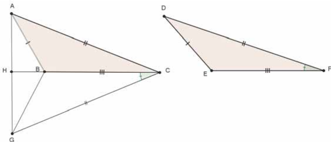
Figura 23: Demonstração do Caso LLL.
