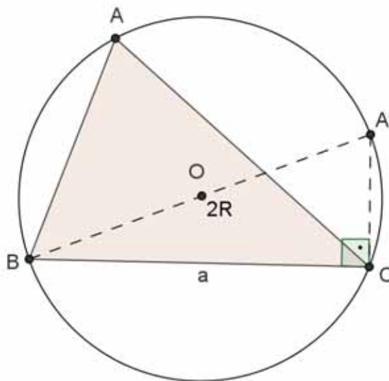
Figura 27: Triângulo ABC inscrito em uma circunferência.
