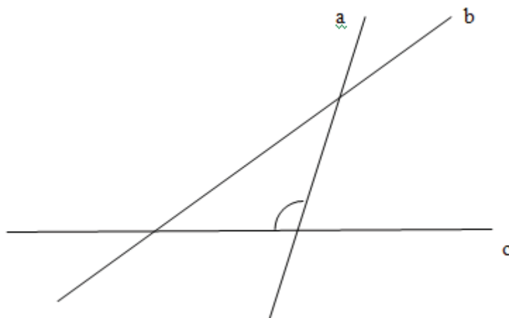
Figura 9: Um triângulo descrito por Euclides.
