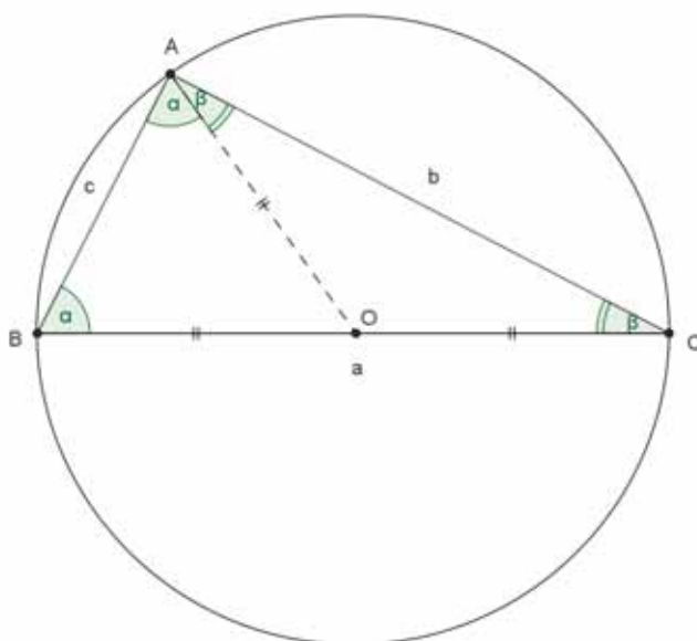
Figura 24: triângulo ABC inscrito em uma circunferência.
