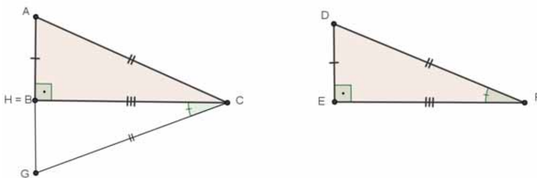
Figura 22: Configuração para o caso quando B e H coincidem.
