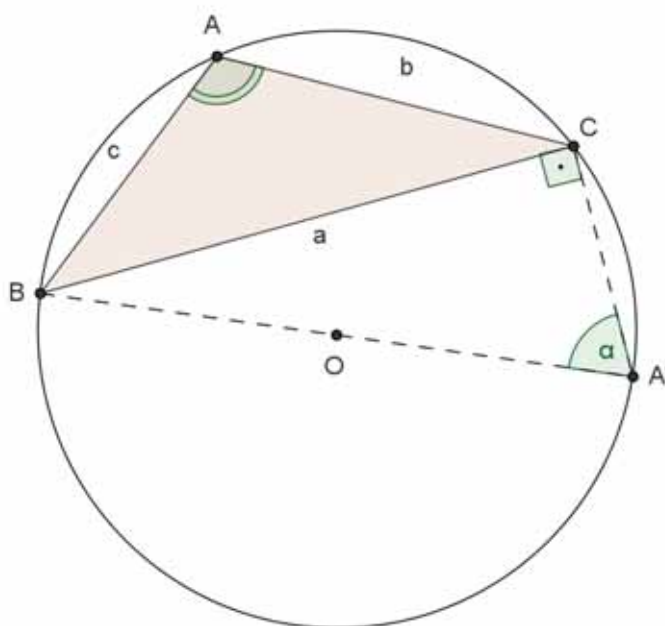
Figura 29: Triângulo ABC obtusângulo.
