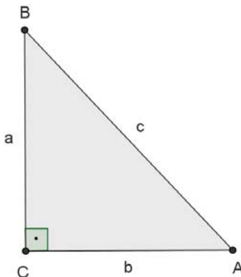
Figura 34: Triângulo ABC retângulo em \hat{C} .
