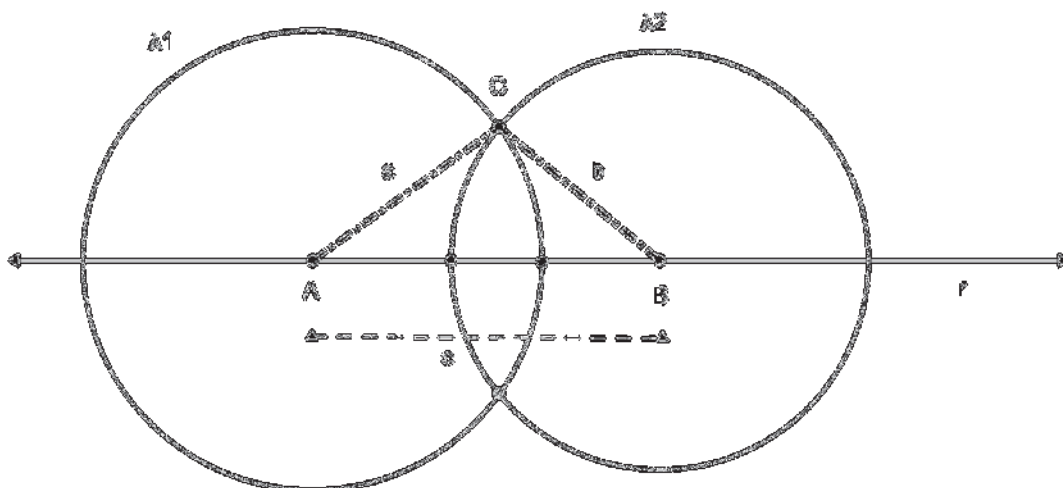
Figura 17: Triângulo ABC , formado pela intersecção das circunferências.
