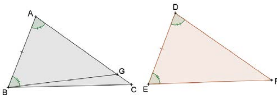
Figura 20: Representação dos triângulos ABC e DEF com os dados. Extraído de Costa (2012, p. 16)
