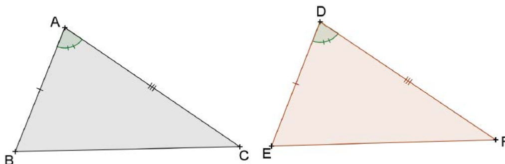
Figura 18: Triângulos congruentes pelo caso LAL. Extraído de Costa (2012, p. 15)
