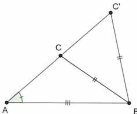
Figura 19: Triângulos ABC e ABC' não congruentes.
