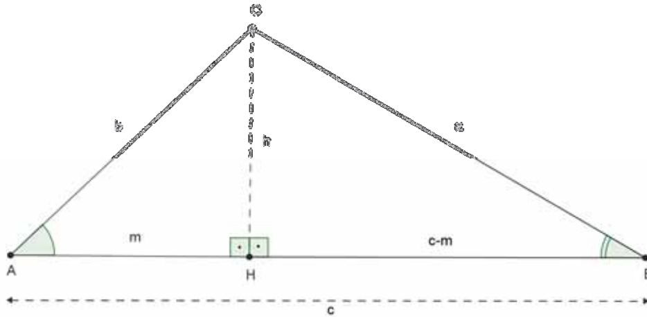
Figura 25: Triângulo ABC com altura \overline{CH} .
