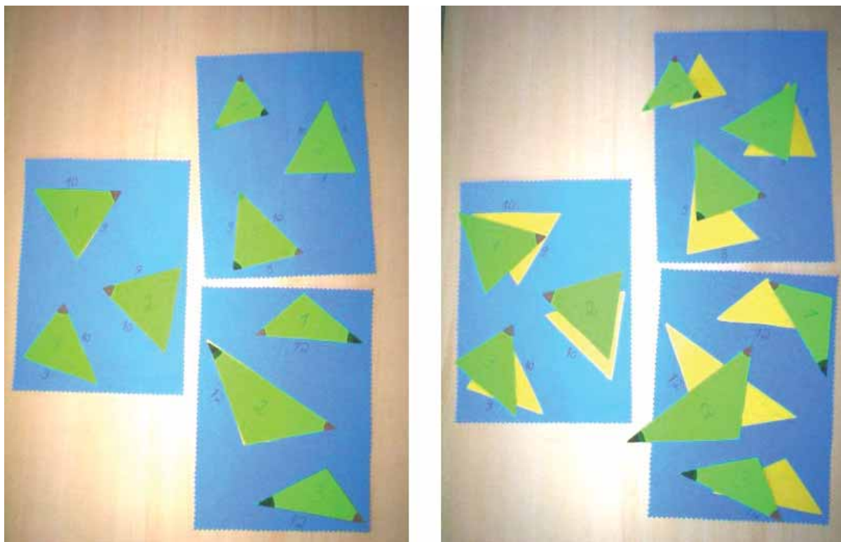
Figura 14 : Modelo dos Casos de Congruência de triângulos. Extraído de LAMAS (2006)
