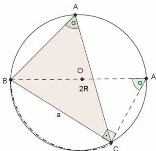
Figura 28: Triângulo ABC acutângulo.
