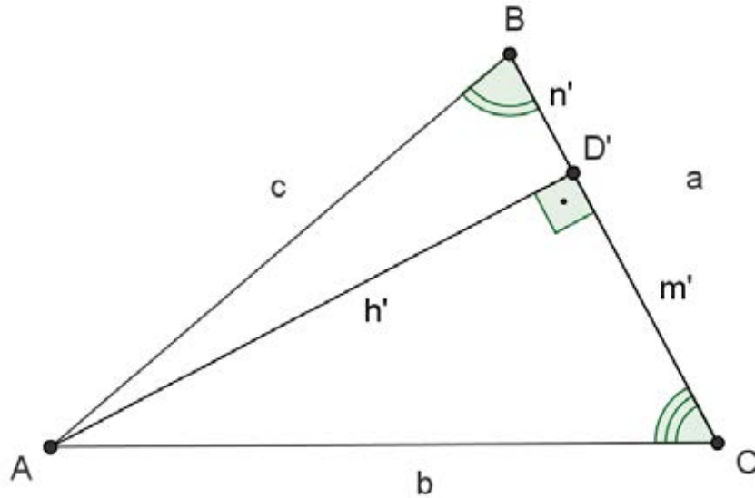
Figura 32: Triângulo ABC com altura \overline{AD'} .
