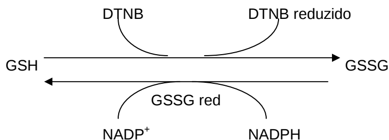
Figura 11. Esquema das reações que ocorrem na determinação do conteúdo de glutathiona total nas amostras de cólon.
