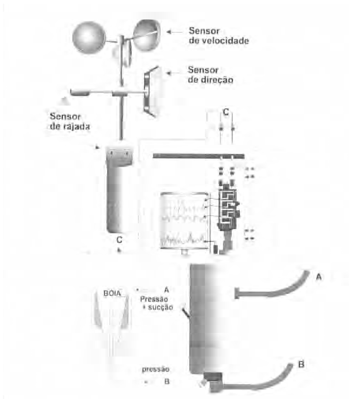
Figura 2.5 – Anemógrafo universal, (VAREJÃO-SILVA ,2005).
