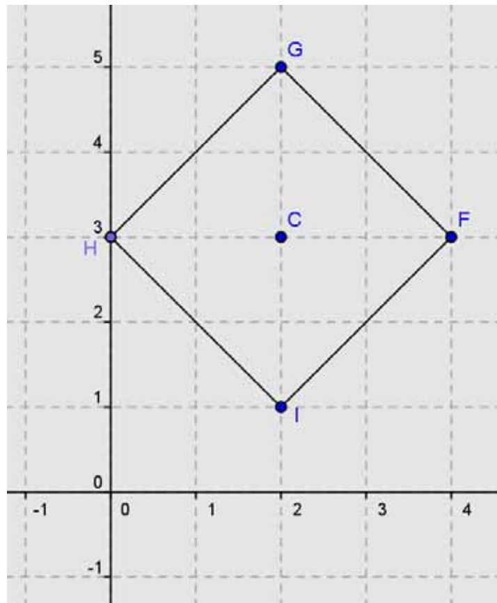
Figura 16: Quadrado FGHI
