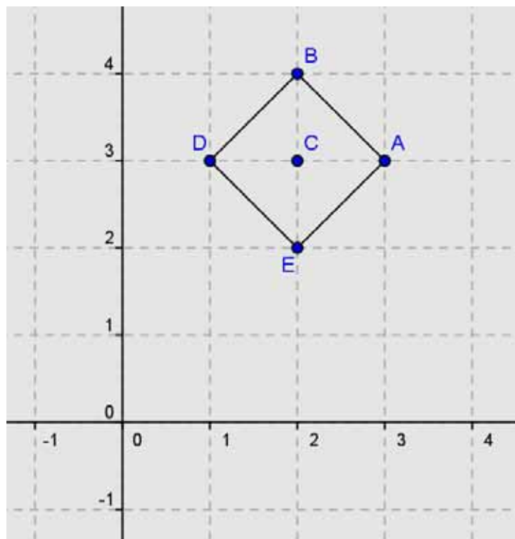
Figura 15: Quadrado ABDE
