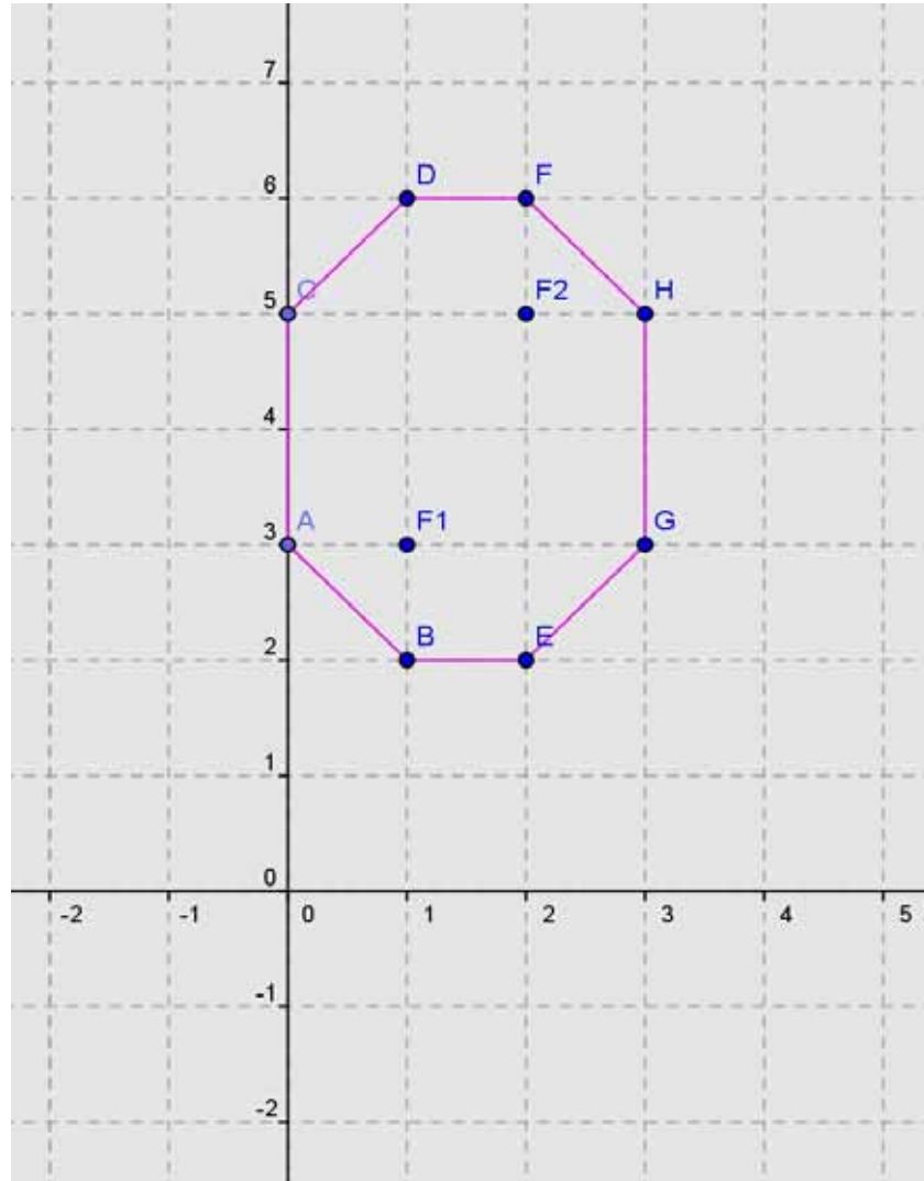
Figura 17: Octógono ABCDEFGH
