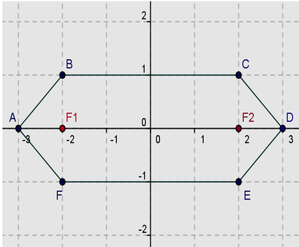
Figura 18: Hexágono ABCDEF
