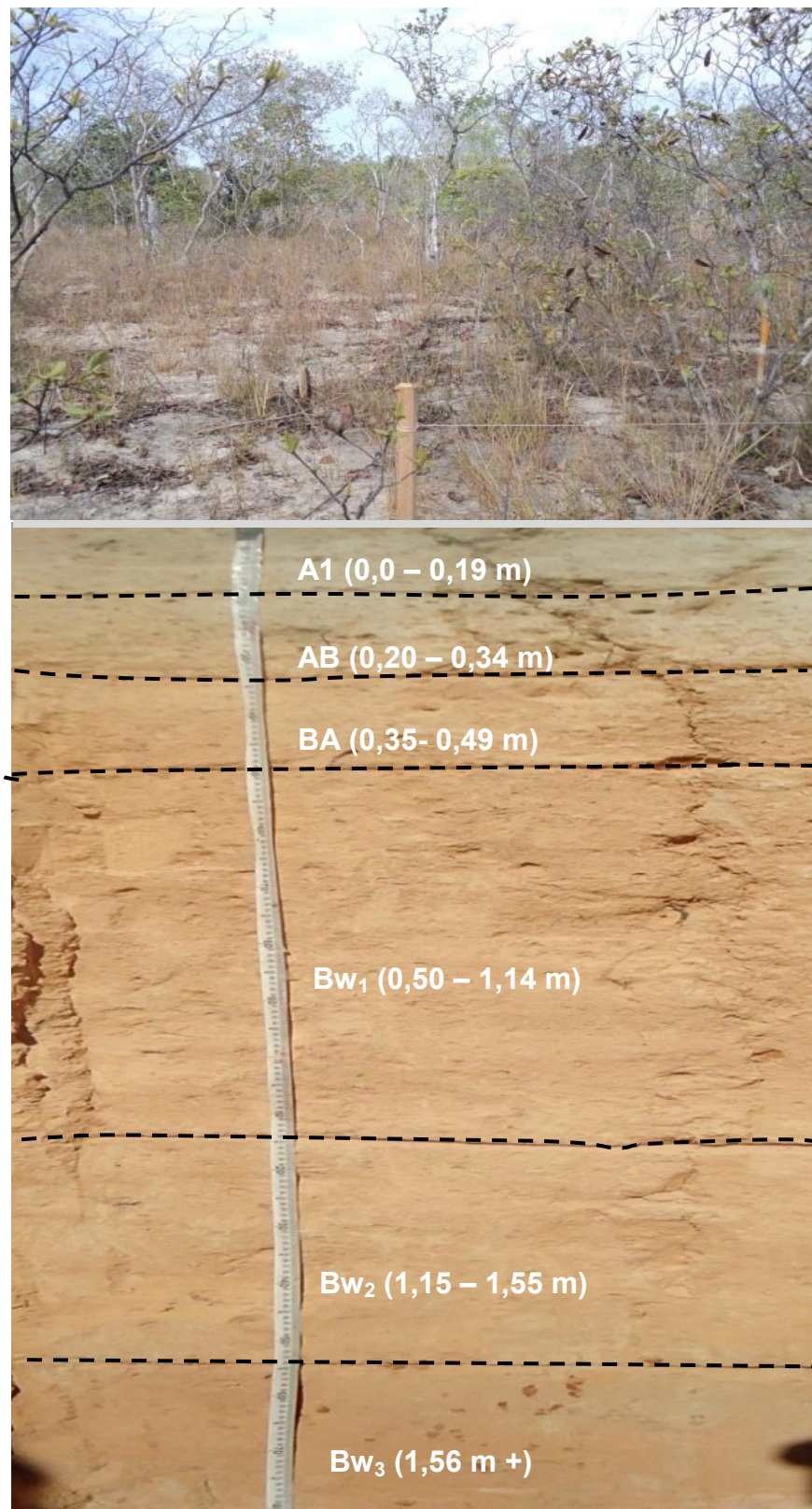
Figura 5. Perfil de LATOSSOLO AMARELO Distrófico típico do ambiente A1 (Campo limpo de Cerrado), localizado em um domínio de Cerrado à Nordeste do Estado do Maranhão.
