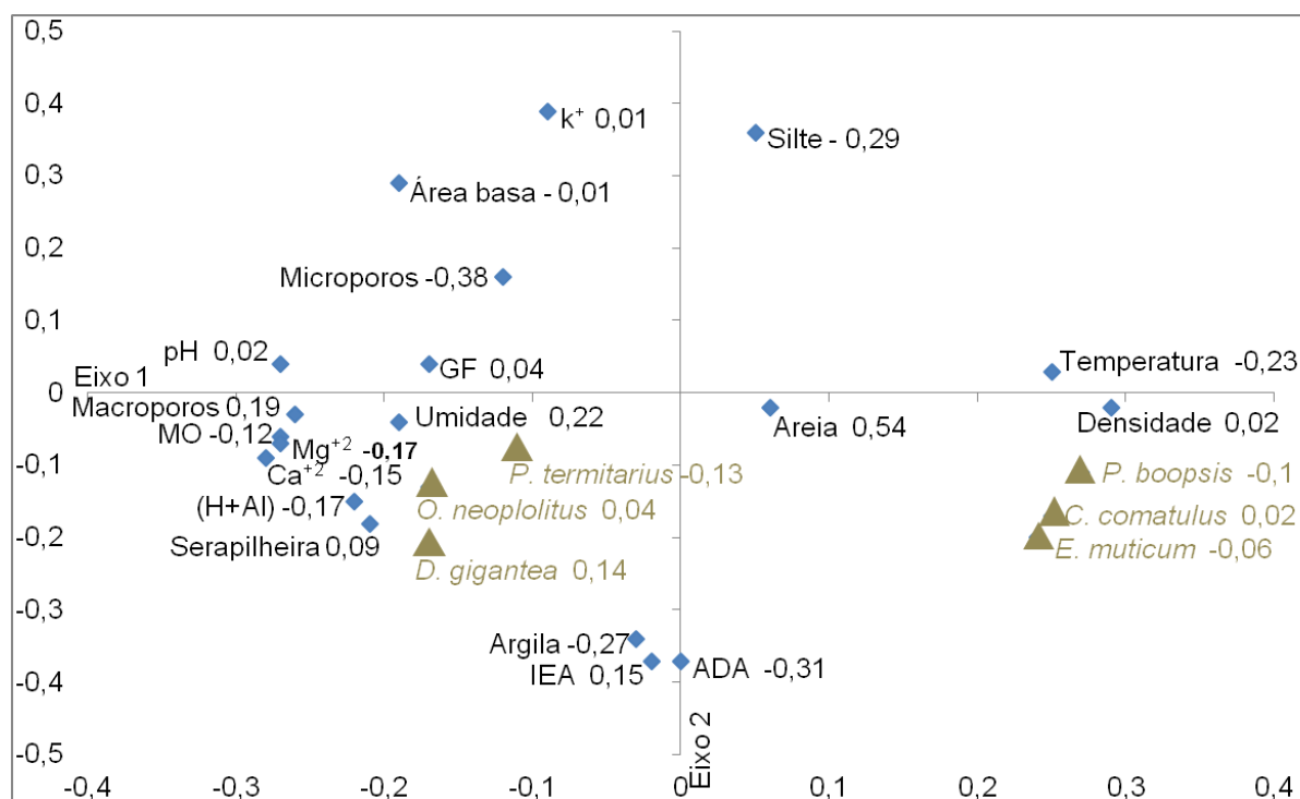
Figura 11. Análise de componentes principais de variáveis do solo, da vegetação e do clima, relacionadas com a ocorrência das espécies de formigas C. comatulus , E. muticum , Pseudomyrmex boopsis , P. termitarius e Dinoponera gigantea coletadas em seis fitofisionomias de Cerrado à Nordeste do Estado do Maranhão.
