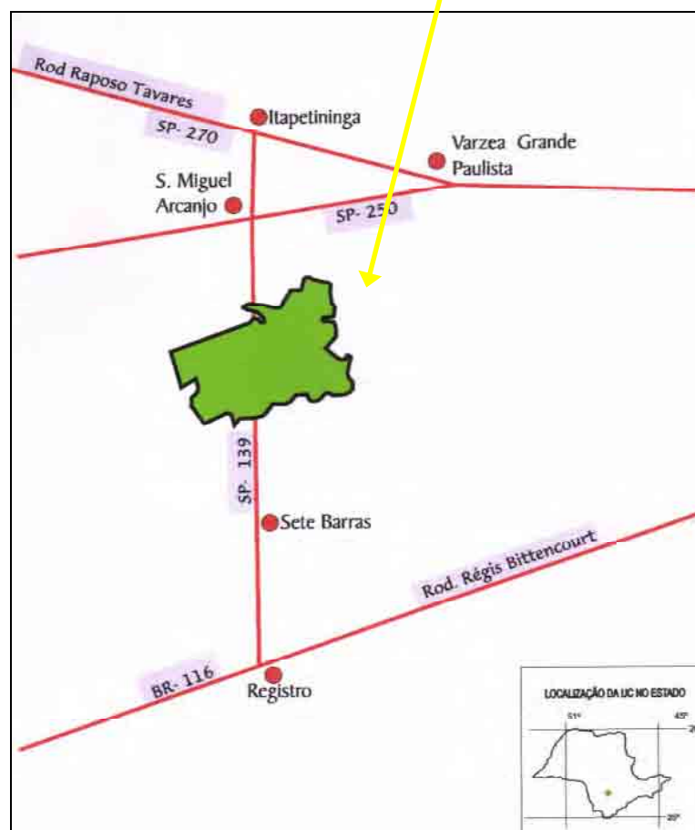
Figura 2 – Localização geográfica do continuum ecológico de Paranapiacaba, SP onde se encontra o Parque Estadual Carlos Botelho (Imagem TM/Landsat de 18 de julho de 1994) (A) e principais acessos para o Parque Estadual Carlos Botelho. Fonte: Instituto Florestal do Estado de São Paulo (B).
