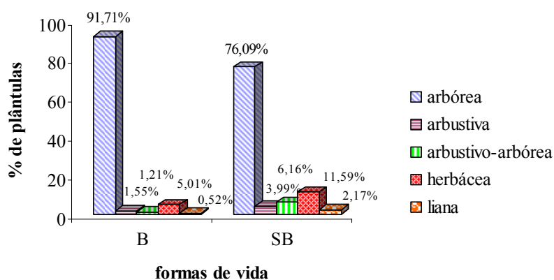
Figura 15 - Porcentagem (%) de plântulas para as formas de vida: arbórea, arbustivo-arbórea, arbustiva, herbácea e lianescente nos ambientes com (B) e sem bambu (SB).
