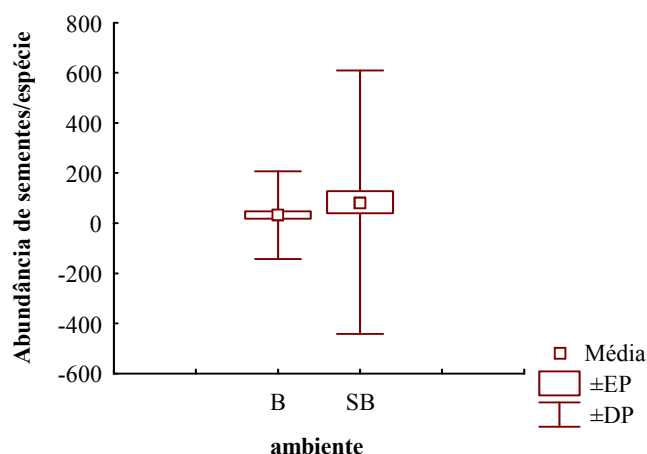
Figura 12 – Abundâncias de sementes por espécie entre os ambientes com (B) e sem bambu (SB).
