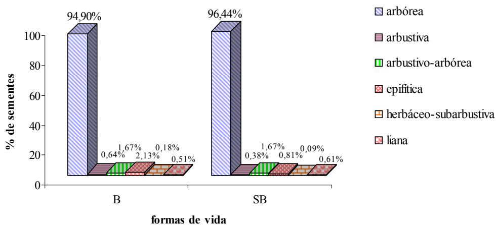
Figura 9 - Porcentagem (%) de sementes para as formas de vida: arbórea, arbustiva, arbustivo-arbórea, epifítica, herbáceo-subarbustiva e lianescente nos ambientes com (B) e sem bambu (SB).
