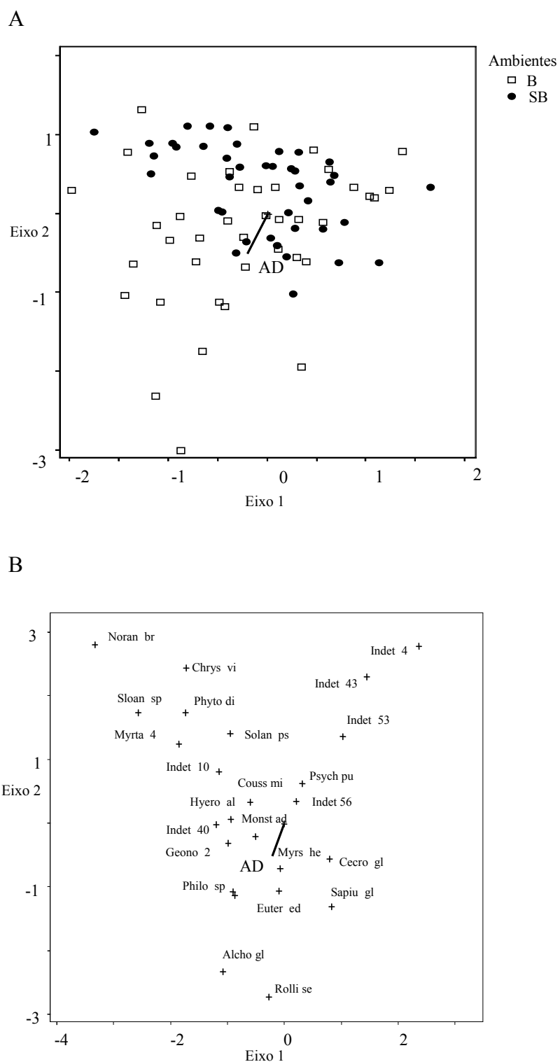
Figura 23 - Diagramas de ordenação nos dois primeiros eixos da análise de correspondência canônica (CCA) para coletores (A) e espécies (B). A análise foi baseada na distribuição do número de sementes de 25 espécies em 80 coletores no PECB e sua correlação com as características do microhabitat abertura de dossel (AD), número de indivíduos adultos (NI) e número de espécies (NE) para a chuva de sementes. Os nomes científicos completos das espécies encontram-se no Anexo 1.
