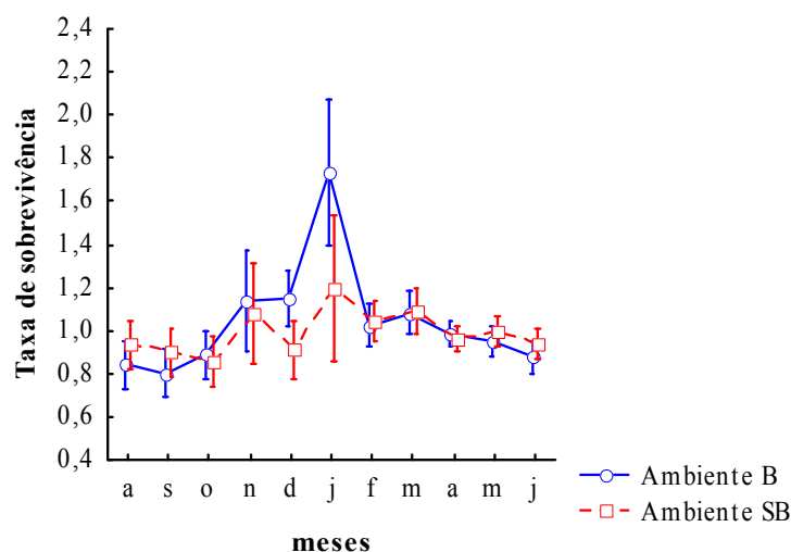
Figura 21 – Taxa de sobrevivência da comunidade de plântulas nos ambientes com (B) e sem bambu (SB) no período de agosto de 2004 a junho de 2005.
