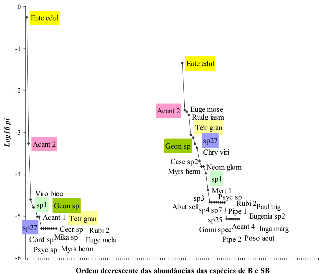
Figura 14 - Curva dominância-diversidade da comunidade de espécies de plântulas dos ambientes com (B) e sem bambu (SB). A abundância relativa de cada espécie de plântula foi ranqueada e plotada em escala logarítmica na base 10 ordenada de forma decrescente (Magurran 1988). Em cada ambiente estão indicadas as espécies mais abundantes na amostragem. Código das seis espécies destacadas na figura nos dois ambientes: Eute edul ( Euterpe edulis ), Acant 2 ( Acanthaceae2 ), Geon sp ( Geonoma sp.), Tetr gran ( Tetrastylidium grandifolium ), sp.1 (não identificada), sp.27 (não identificada). Os nomes científicos das demais espécies se encontram no Anexo 3.
