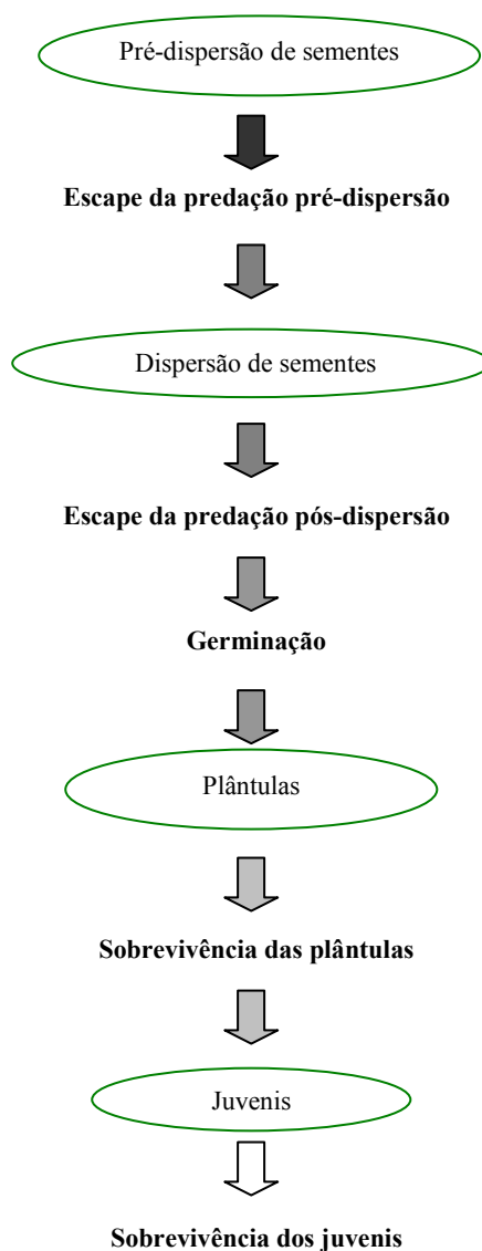
Figura 1 - Diagrama da regeneração natural desde a semente até o recrutamento dos juvenis (modificado de Rey & Alcántara 2000, Jordano et al. 2004).
