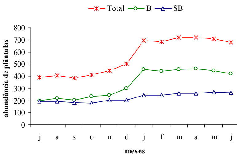
Figura 17 – Abundância total de plântulas por mês e para os ambientes com (B) e sem bambu (SB) referente ao período de julho de 2004 a junho de 2005.
