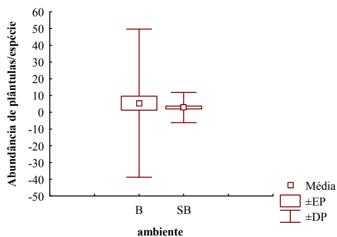
Figura 18 - Abundâncias de plântulas por espécie entre os ambientes com (B) e sem bambu (SB).
