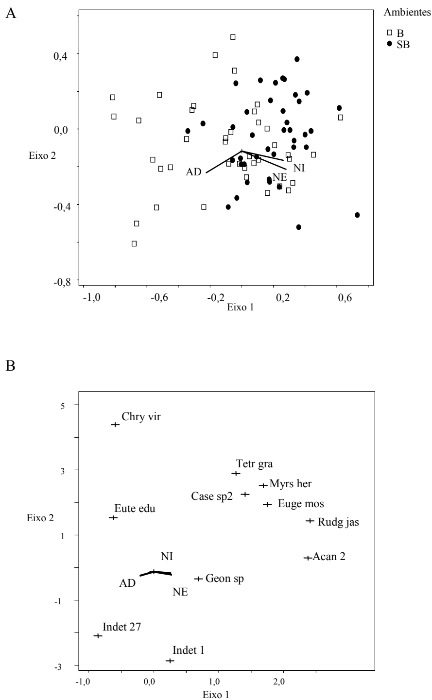
Figura 24 - Diagramas de ordenação nos dois primeiros eixos da análise de correspondência canônica (CCA) para parcelas (A) e espécies (B). A análise foi baseada na distribuição do número de plântulas de 11 espécies em 80 parcelas no PECB e sua correlação com as características do microhabitat abertura de dossel (AD), número de indivíduos adultos (NI) e número de espécies (NE) para as plântulas. Os nomes científicos completos das espécies encontram-se no Anexo 3.
