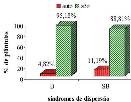
Figura 16 - Porcentagem (%) de plântulas para as categorias de síndrome de dispersão: autocórica (auto) e zoocórica (zôo) nos ambientes com (B) e sem bambu (SB).
