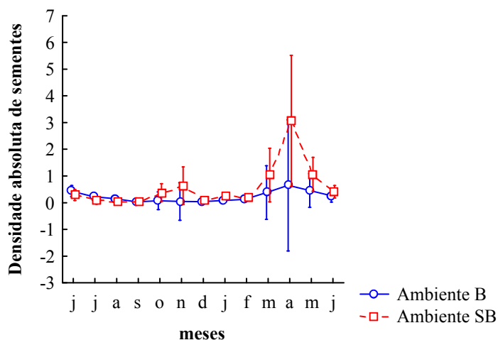
Figura 13 – Densidade absoluta de sementes nos ambientes com (B) e sem bambu (SB) no período de junho de 2004 a junho de 2005.
