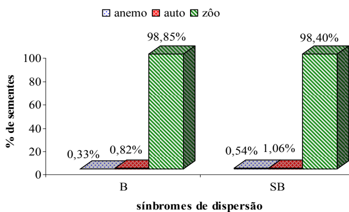
Figura 10 - Porcentagem (%) de sementes para as síndromes de dispersão: anemocórica (anemo), autocórica (auto) e zoocórica (zôo) nos ambientes com (B) e sem bambu (SB).
