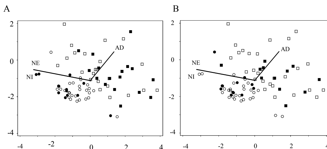
Figura 22 - Diagramas de ordenação nos dois primeiros eixos (eixo1-horizonta e eixo2-vertical) da análise de componentes principais (PCA) segundo as características do microhabitat abertura de dossel (AD), número de indivíduos adultos (NI) e número de espécies (NE). Os coletores e parcelas são classificados segundo as variáveis do ambiente nos diagramas A e B, respectivamente. Quadrados e círculos cheios em A representam coletores com abundância acima de 100 sementes e em B representam parcelas com abundância acima de 10 plântulas. Características do microhabitat são representadas por vetores. Ambiente B □ e Ambiente SB ○
