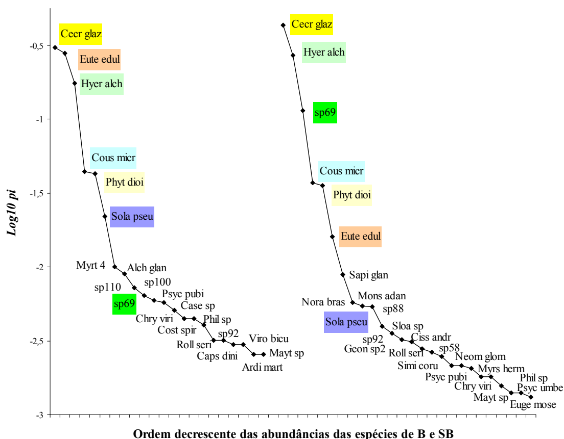
Figura 8 - Curva dominância-diversidade da comunidade de espécies de sementes dos ambientes com (B) e sem bambu (SB). A abundância relativa de cada espécie de semente foi ranqueada e plotada em escala logarítmica na base 10 ordenada de forma decrescente (Magurran 1988). Em cada ambiente estão indicadas as espécies mais abundantes na amostragem. Código das sete espécies destacadas nos dois ambientes: Cocr glaz ( Cecropia glaziovii ), Eute edul ( Euterpe edulis ), Hyer alch ( Hyeronima alchorneoides ), Cous micr ( Coussapoua microcarpa ), Sola pseu ( Solanum pseudoquina ), Phyt dioi ( Phytolacca dioica ) e sp.69 (não identificada). Os nomes científicos das demais espécies se encontram no Anexo 1.
