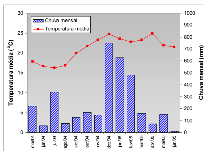
Figura 4 - Regime térmico e hídrico do PECB, em Sete Barras, SP, no período de maio de 2004 a junho de 2005.
