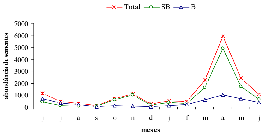
Figura 11 – Abundância total de sementes por mês e para os ambientes com (B) e sem bambu (SB) referente ao período de junho de 2004 a junho de 2005.
