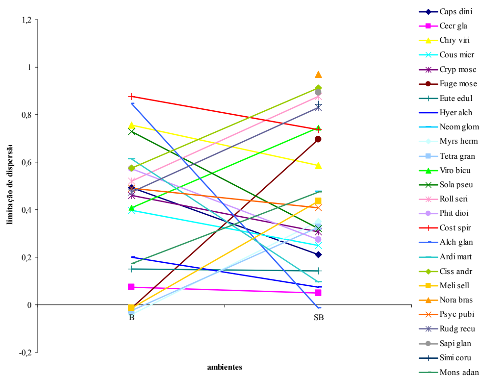
Figura 25 – Limitação de dispersão para 26 espécies registradas na chuva de sementes dos ambientes com (B) e sem bambu (SB). Valores próximos de 1,0 representam maior limitação. Os nomes completos das espécies estão no Anexo 1.
