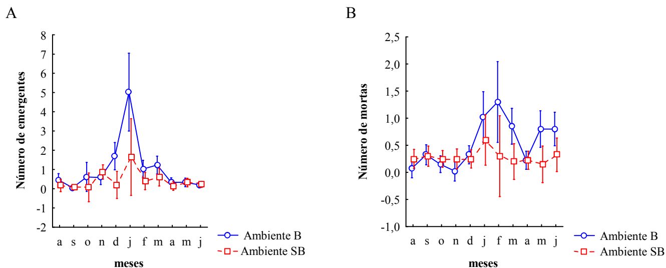
Figura 20 – Número de plântulas emergentes (A) e mortas (B) nos ambientes com (B) e sem bambu (SB) no período de agosto de 2004 a junho de 2005.
