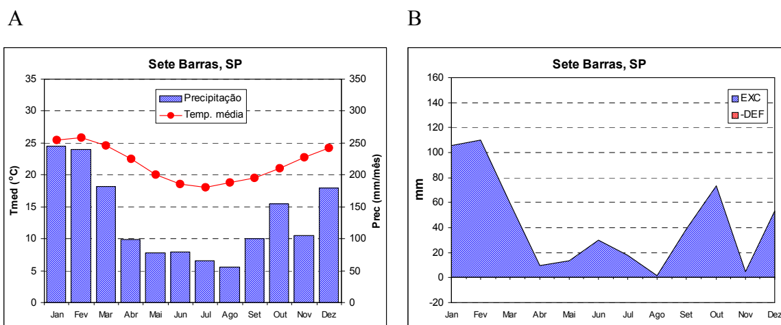
Figura 3 - Regime térmico e hídrico (A) e balanço hídrico (B) climatológico normal de Sete Barras, SP. Fonte: Departamento de Águas e Energia Elétrica.
