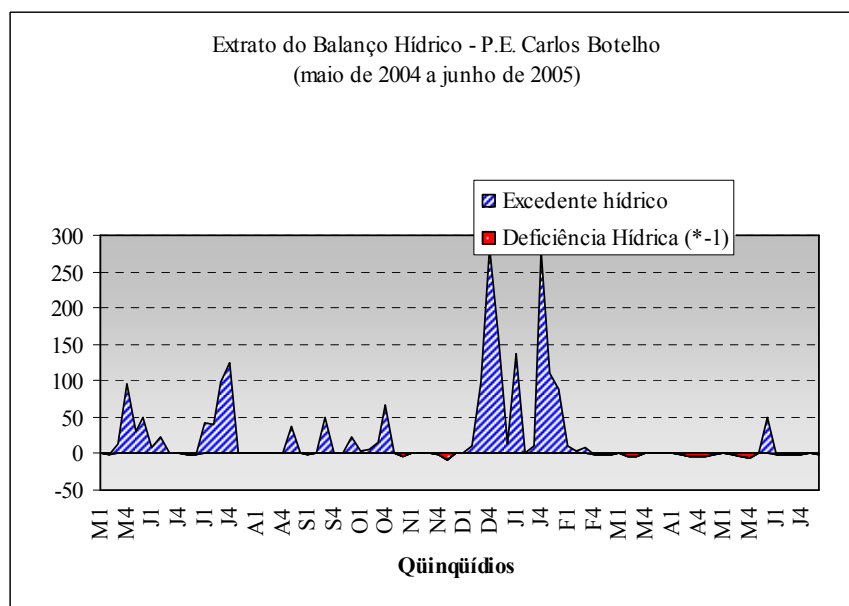
Figura 1 – Extrato do balanço hídrico para o período de maio de 2004 a junho de 2005 para o PECB.
