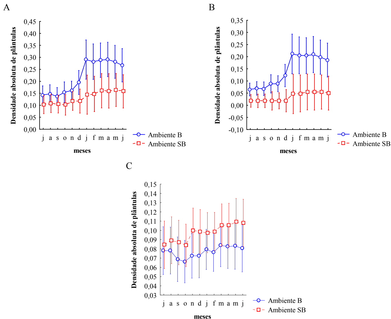
Figura 19 – Densidade absoluta de plântulas de TODAS as espécies (A), Euterpe edulis (B) e OUTRAS espécies (C) nos ambientes com (B) e sem bambu (SB) no período de julho de 2004 a junho de 2005.
