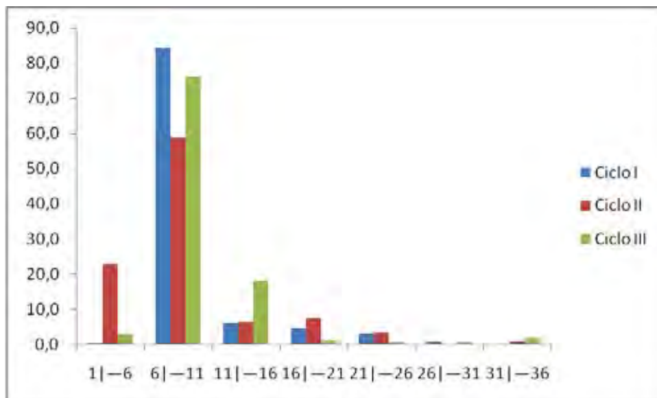
Figura 8: Frequência relativa (%) pela classe de comprimento padrão (cm) de captura de C. monocolus durante as coletas relacionadas ao estudo.
