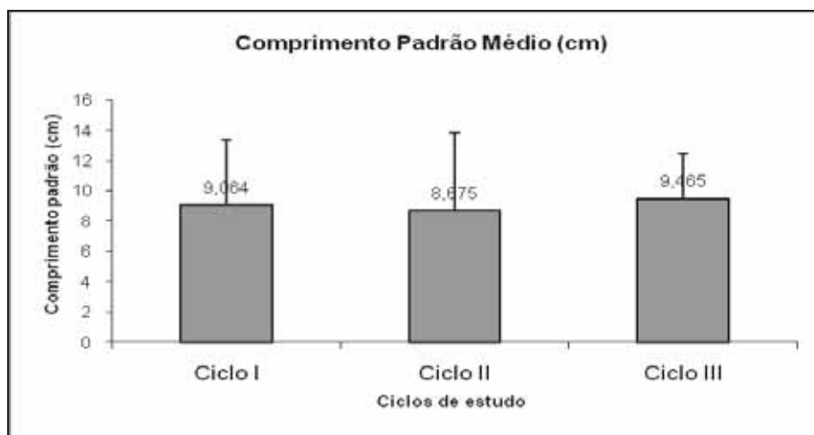
Figura 4: Comprimento padrão médio (cm) e desvio padrão dos espécimes de C. monoculus capturados durante o estudo.
