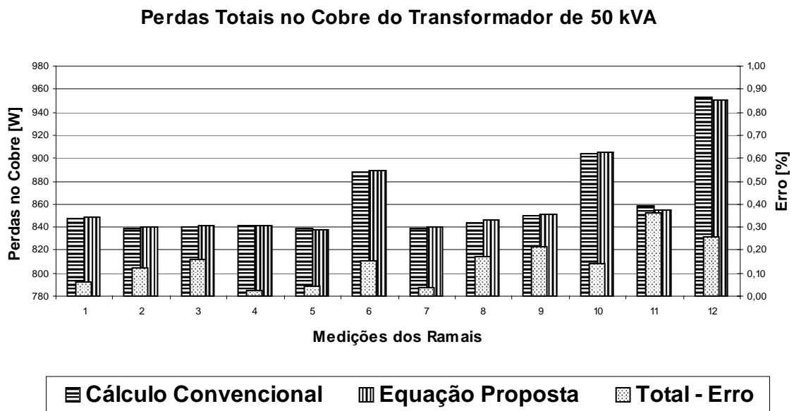
Figura 3.18 – Gráfico das Perdas No Cobre Transformador 50 kVA Utilizando as Equações Convencional e Proposta.
