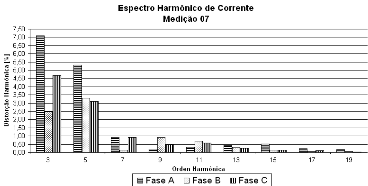
Figura 3.07 – Espectro harmônico de corrente da medição efetuada no período de 01/01/2004 (00:20) a 01/01/2004 (01:30) – quinta-feira.
