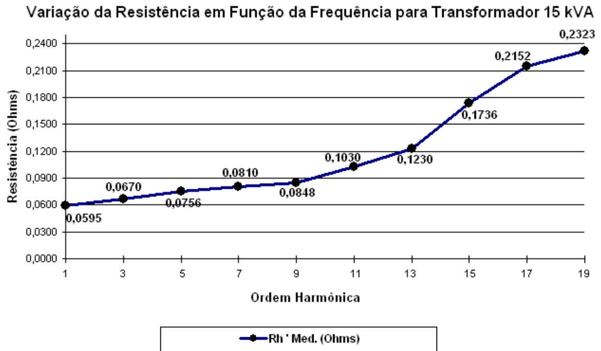
Figura 2.07 – Comportamento da resistência CA do transformador de 15 kVA em função da frequência.
