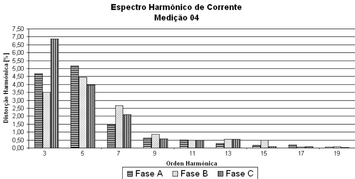
Figura 3.04 – Espectro harmônico de corrente da medição efetuada no período de 04/01/2004 (03:10) a 04/01/2004 (04:10) – domingo.
