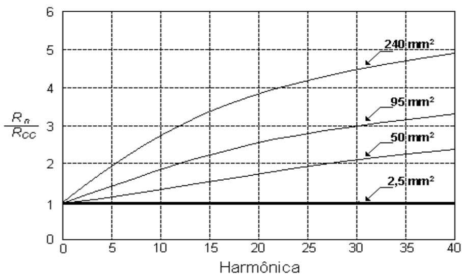
Figura 1.01 – Relação entre as resistências CA e CC em função da frequência harmônica para condutores de diferentes secções.
