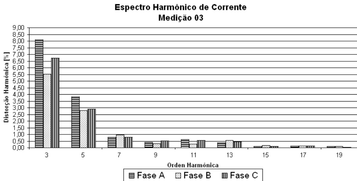
Figura 3.03 – Espectro harmônico de corrente da medição efetuada no período de 06/01/2004 (20:00) a 06/01/2004 (21:50) – terça-feira.
