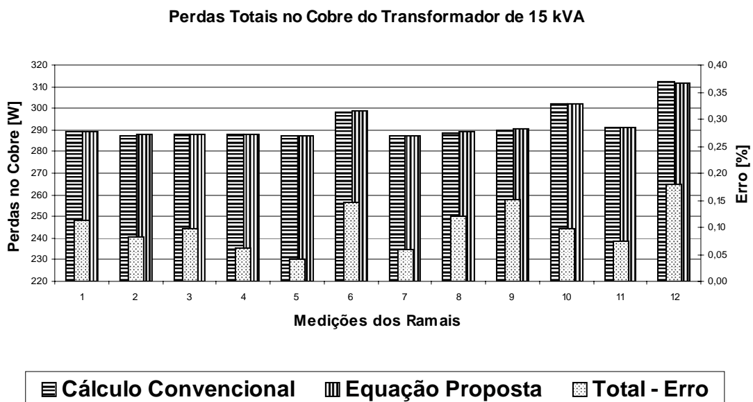
Figura 3.19 – Gráfico das Perdas No Cobre Transformador 15 kVA Utilizando as Equações Convencional e Proposta.
