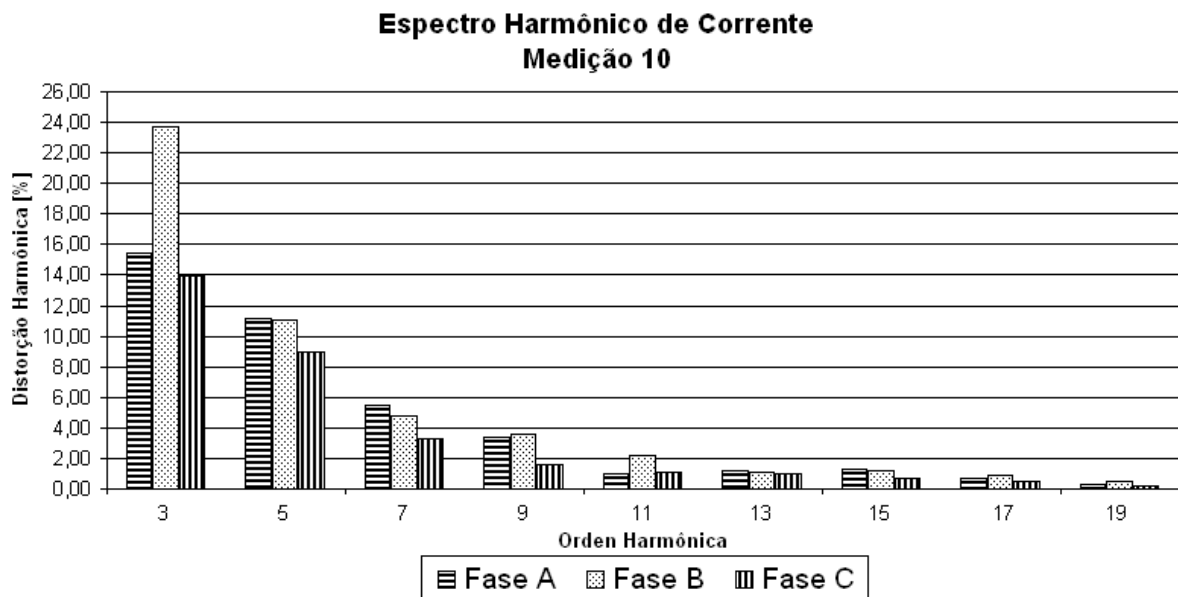
Figura 3.10 – Espectro harmônico de corrente da medição efetuada no período de 27/12/2003 (08:15) a 27/12/2003 (09:38) – sábado.
