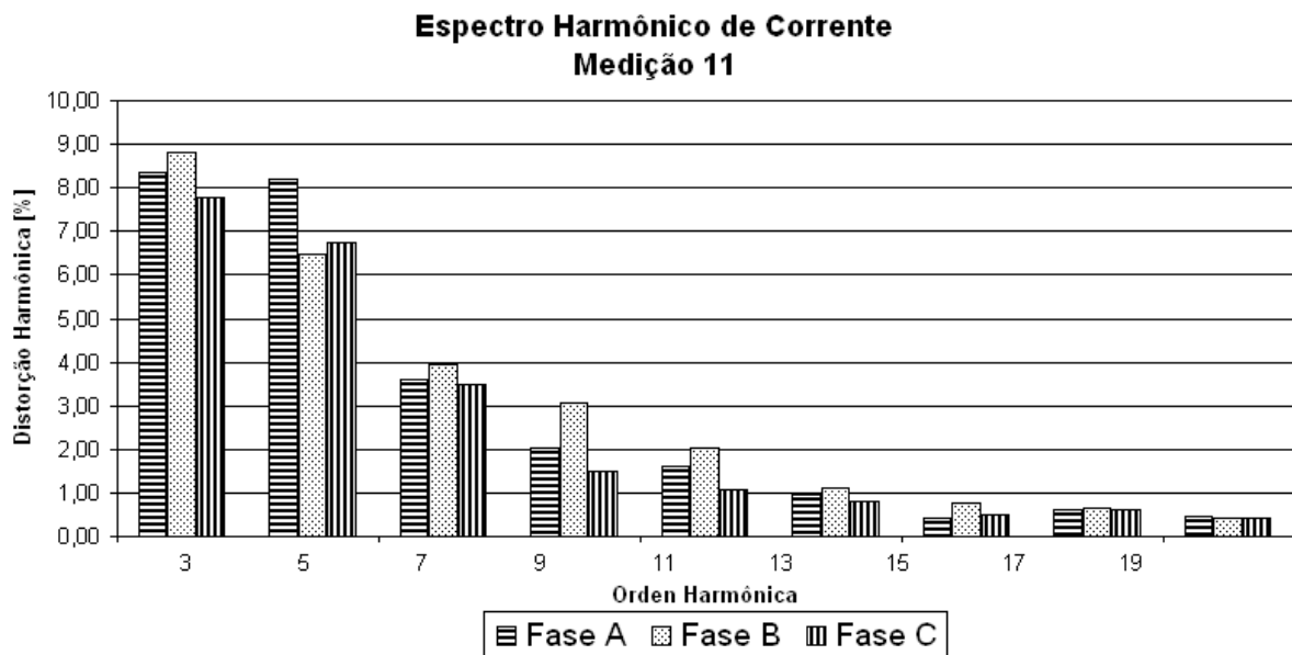
Figura 3.11 – Espectro harmônico de corrente da medição efetuada no período de 28/12/2003 (01:30) a 28/12/2003 (03:30) – sábado.
