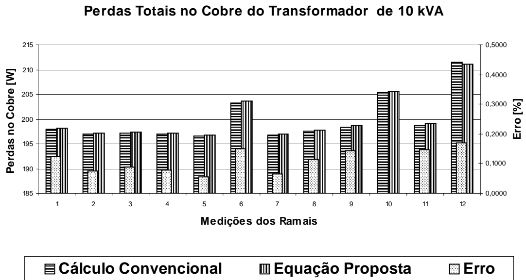
Figura 3.17 – Gráfico das Perdas No Cobre Transformador 10 kVA Utilizando as Equações Convencional e Proposta.
