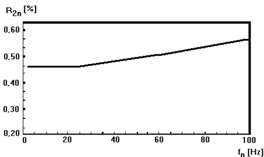
Figura 1.04 – Resistência do enrolamento de baixa tensão em função da frequência.
