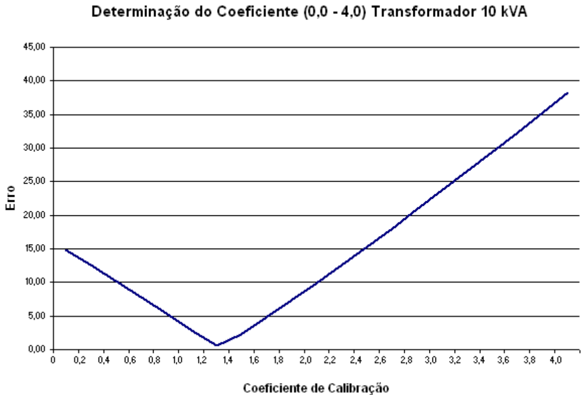
Figura 3.14 – Detalhe do Ponto de valor mínimo do erro quadrático em função do valor de a para a unidade transformadora de 10 kVA (intervalo (0,0 a 4,0)).
