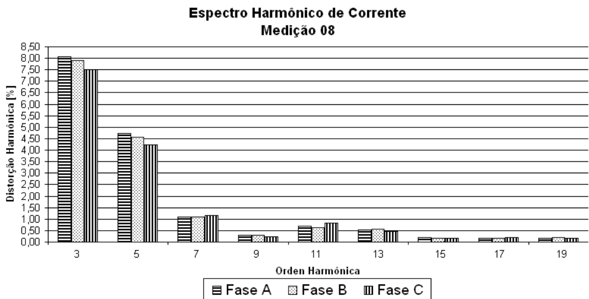
Figura 3.08 – Espectro harmônico de corrente da medição efetuada no período de 03/01/2004 (13:20) a 03/01/2004 (17:20) – sábado.
