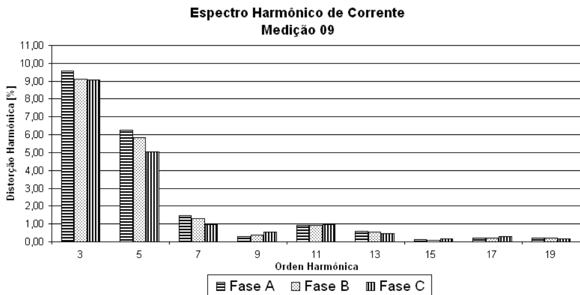
Figura 3.09 – Espectro harmônico de corrente da medição efetuada no período de 04/01/2004 (13:30) a 04/01/2004 (17:30) – domingo.
