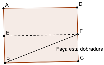
Figura 2.29: Pentágono regular - passo 3
