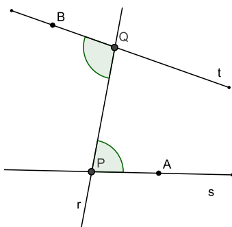
Figura 1.20: Ângulos Alternos Internos
