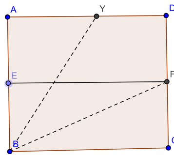
Figura 2.30: Pentágono regular - passo 4
