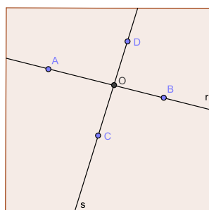
Figura 2.23: Congruência dos ângulos opostos pelo vértice - passo 3
