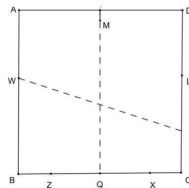
Figura 2.40: Pentágono regular - passo 14
