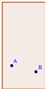
Figura 2.1: Reta por dois pontos - passo 1
