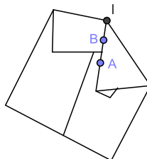
Figura 2.10: Bissetriz de um ângulo - passo 2
