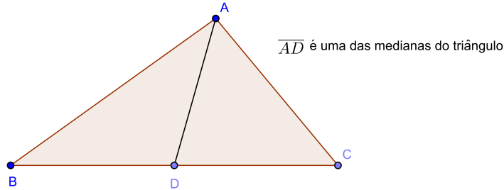
Figura 1.17: Mediana do triângulo
