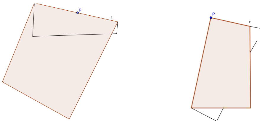
Figura 2.14: Reta perpendicular, P \in r - passo 3
