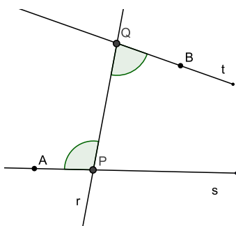
Figura 1.21: Ângulos Alternos Internos
