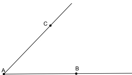
Figura 1.6: Ângulo \widehat{BAC}
