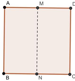
Figura 3.3: Divisão de um segmento de reta em 3 partes iguais - passo 1
