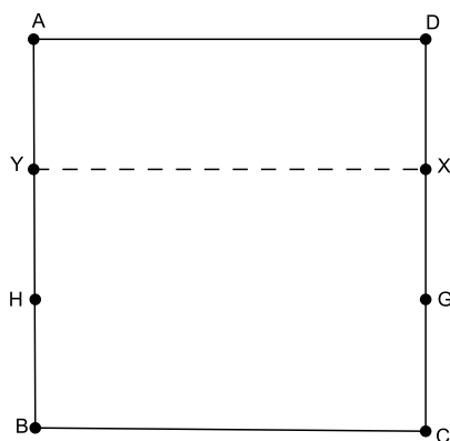
Figura 3.7: Divisão de um segmento de reta em 3 partes iguais - passo 5
