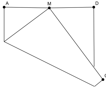
Figura 3.4: Divisão de um segmento de reta em 3 partes iguais - passo 2
