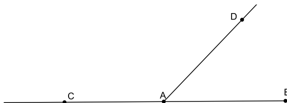
Figura 1.7: Par Linear
