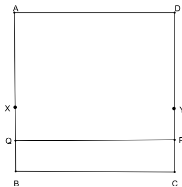
Figura 3.16: Divisão de um segmento de reta em 5 partes iguais - passo 8
