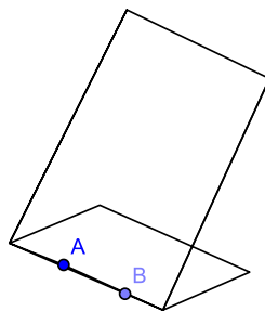
Figura 2.5: Mediatriz e ponto médio de um segmento de reta - passo 2
