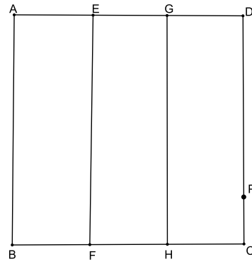
Figura 3.11: Divisão de um segmento de reta em 5 partes iguais - passo 3
