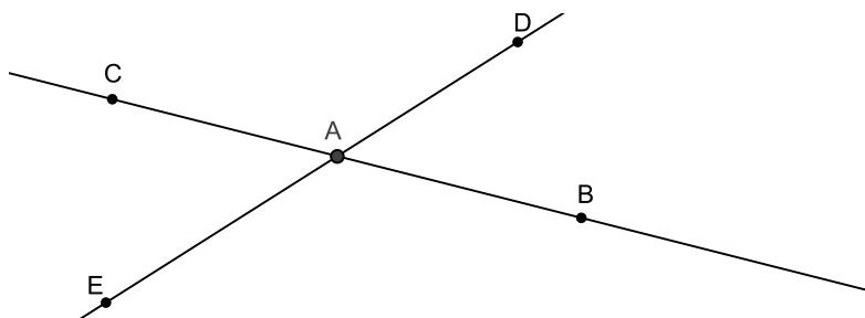
Figura 1.8: Ângulos Opostos pelo Vértice
