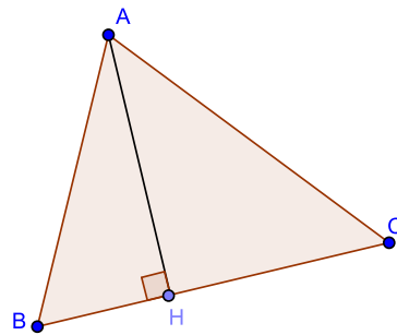
Figura 2.25: Soma dos ângulos internos de um triângulo - passo 1
