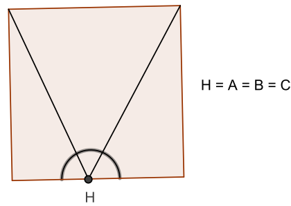
Figura 2.26: Soma dos ângulos internos de um triângulo - passo 2
