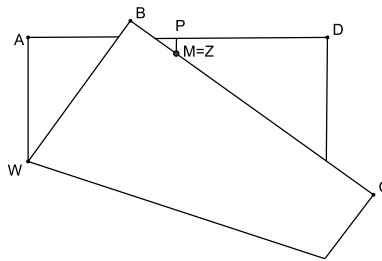
Figura 2.39: Pentágono regular - passo 13
