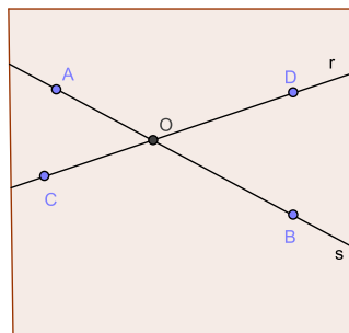
Figura 2.20: Ângulos opostos pelo vértice
