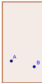
Figura 2.4: Mediatriz e ponto médio de um segmento de reta - passo 1
