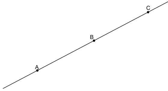
Figura 1.3: O ponto B está entre os pontos A e C
