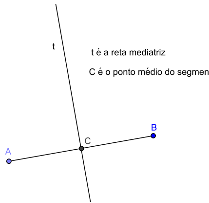
Figura 1.16: Mediatriz de \overline{AB}
