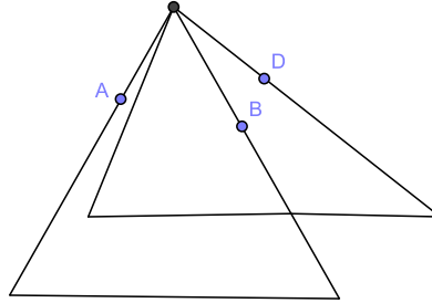
Figura 2.24: Congruência dos ângulos opostos pelo vértice - passo 4
