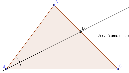
Figura 1.11: Bissetriz do triângulo
