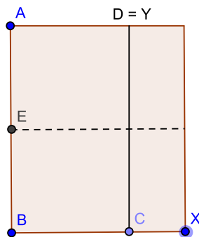
Figura 2.31: Pentágono regular - passo 5
