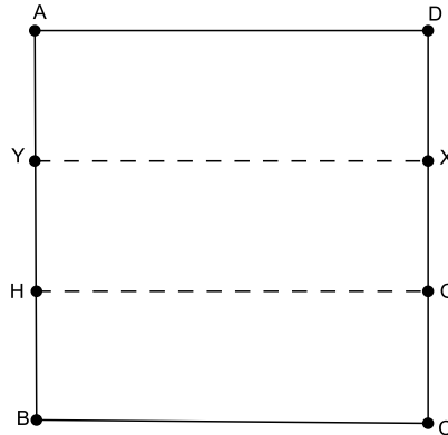
Figura 3.8: Divisão de um segmento de reta em 3 partes iguais - passo 6
