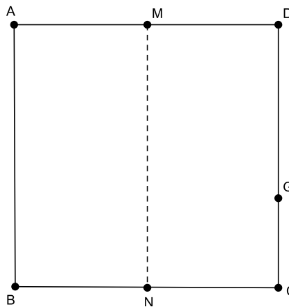
Figura 3.5: Divisão de um segmento de reta em 3 partes iguais - passo 3
