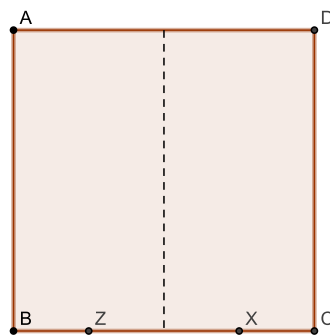
Figura 2.34: Pentágono regular - passo 8
