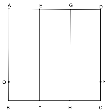
Figura 3.13: Divisão de um segmento de reta em 5 partes iguais - passo 5
