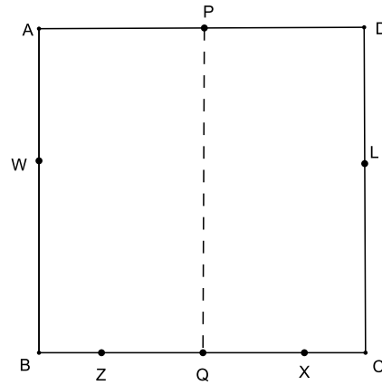
Figura 2.38: Pentágono regular - passo 12
