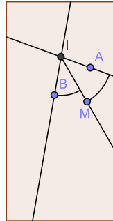
Figura 2.11: Bissetriz de um ângulo - passo 3
