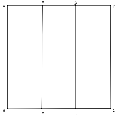
Figura 3.9: Divisão de um segmento de reta em 5 partes iguais - passo 1
