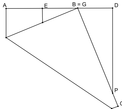
Figura 3.10: Divisão de um segmento de reta em 5 partes iguais - passo 2
