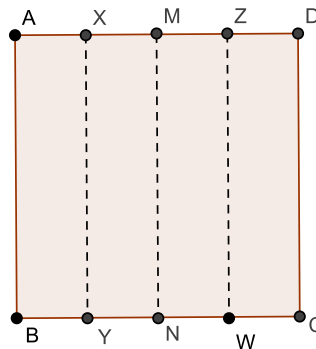
Figura 3.2: Divisão de um segmento de reta em 2^n partes iguais - passo 2
