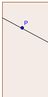
Figura 2.12: Reta perpendicular, P \in r - passo 1
