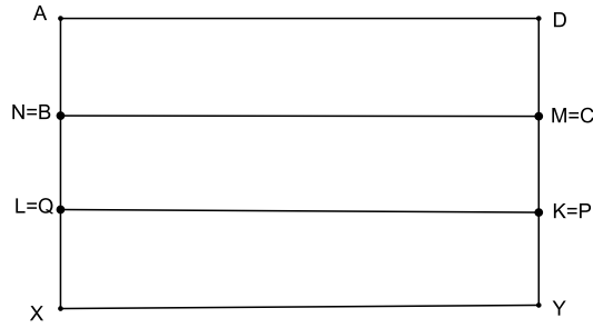
Figura 3.17: Divisão de um segmento de reta em 5 partes iguais - passo 9
