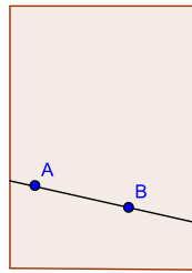
Figura 2.3: Reta por dois pontos - passo 3
