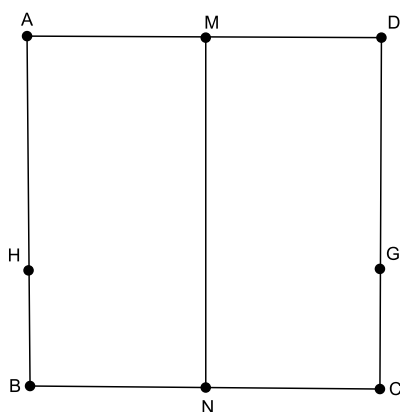
Figura 3.6: Divisão de um segmento de reta em 3 partes iguais - passo 4
