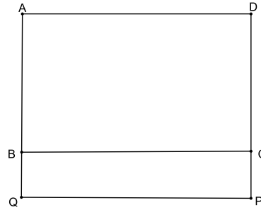
Figura 3.14: Divisão de um segmento de reta em 5 partes iguais - passo 6
