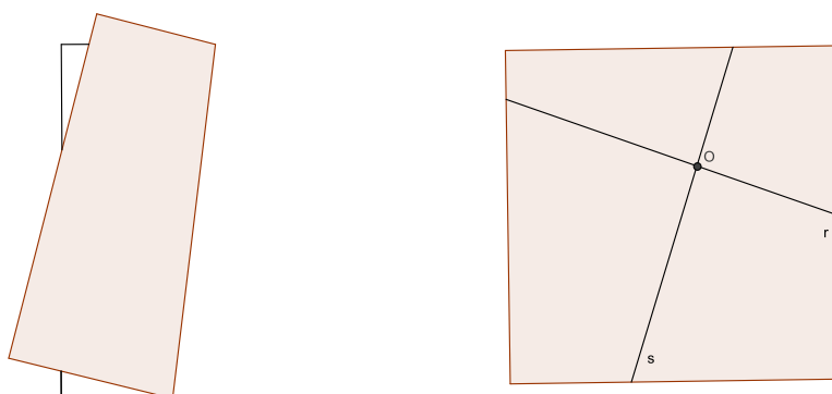
Figura 2.22: Congruência dos ângulos opostos pelo vértice - passo 2
