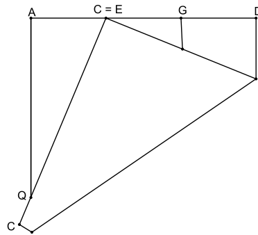
Figura 3.12: Divisão de um segmento de reta em 5 partes iguais - passo 4
