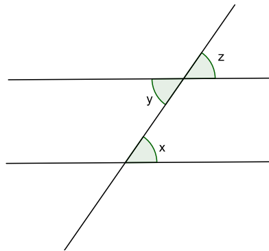
Figura 1.24: Ângulos Correspondentes
