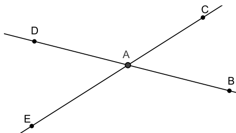
Figura 1.9: Ângulos opostos pelo vértice
