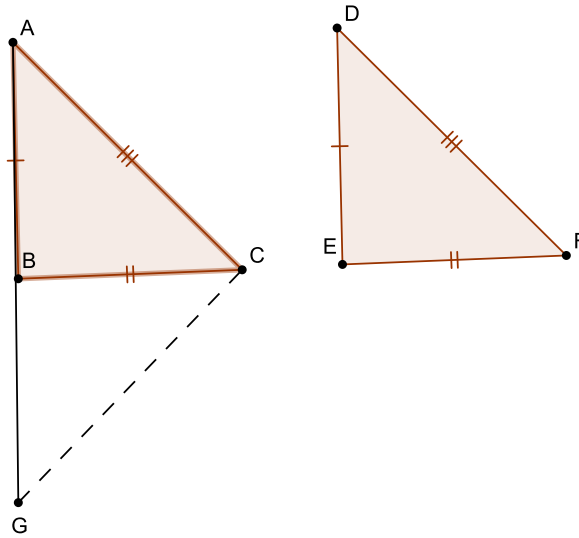
Figura 1.15: Terceiro caso de congruência de triângulos - H = B
