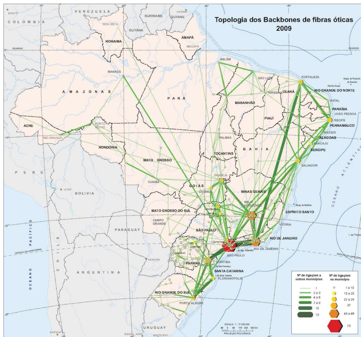
Mapa 8 – Topologia dos backbones de fibras óticas no Brasil, 2009.
