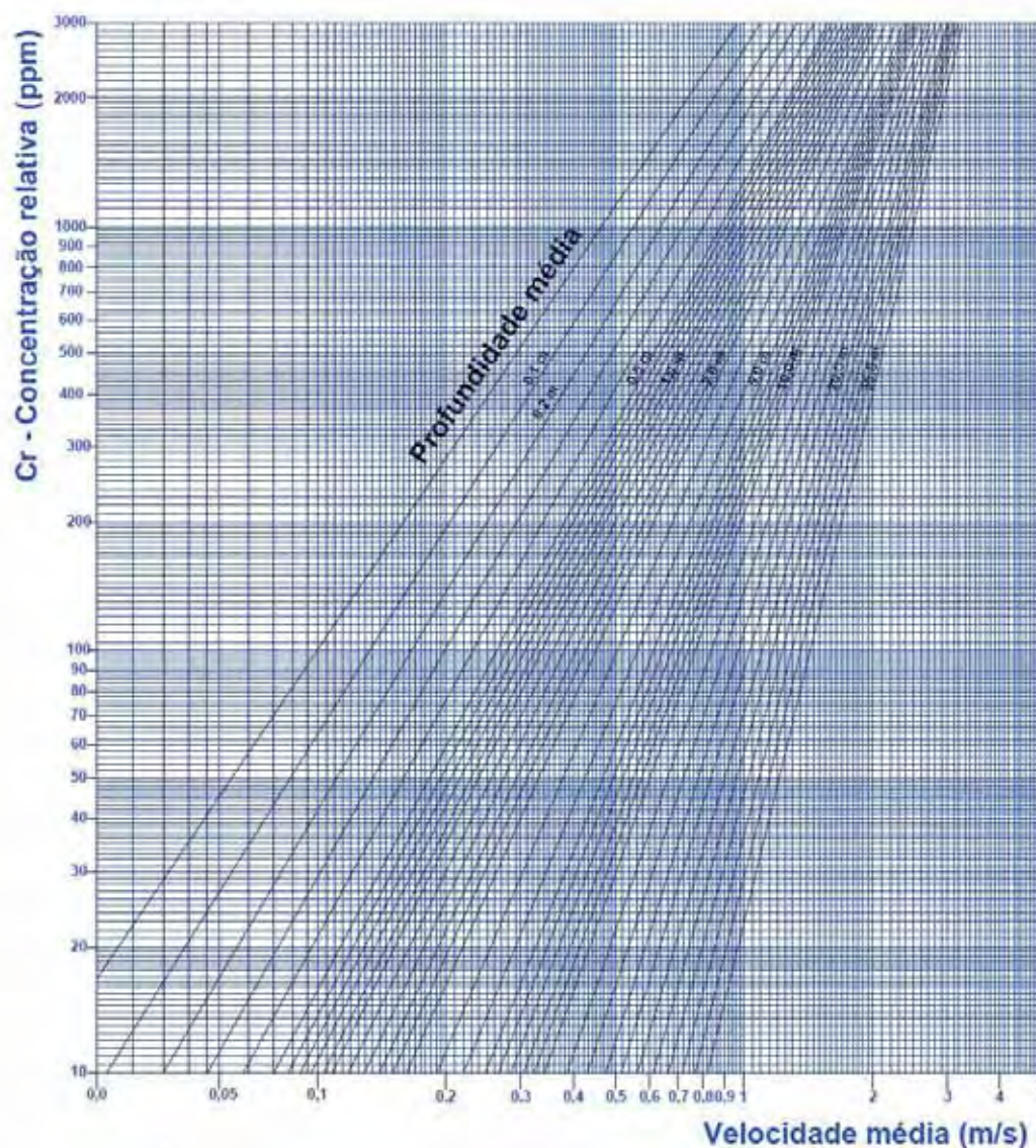
Figura 23 - Ábaco para a determinação da concentração relativa.
