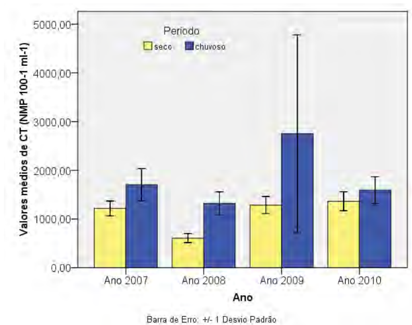
Figura 87 - Valores médios de coliformes totais por ano de amostragem, na microbacia do córrego do Coqueiro.
