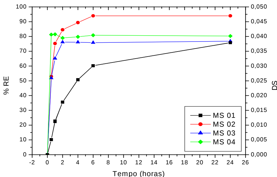
Figura 9. Perfis dos valores de RE (%) e DS em amido de mandioca salsa tratado com diferentes relações molares de hidróxido de sódio e monômero, em função do tempo.
