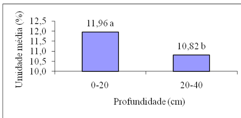
Figura 16. Umidade do solo em função da profundidade.
