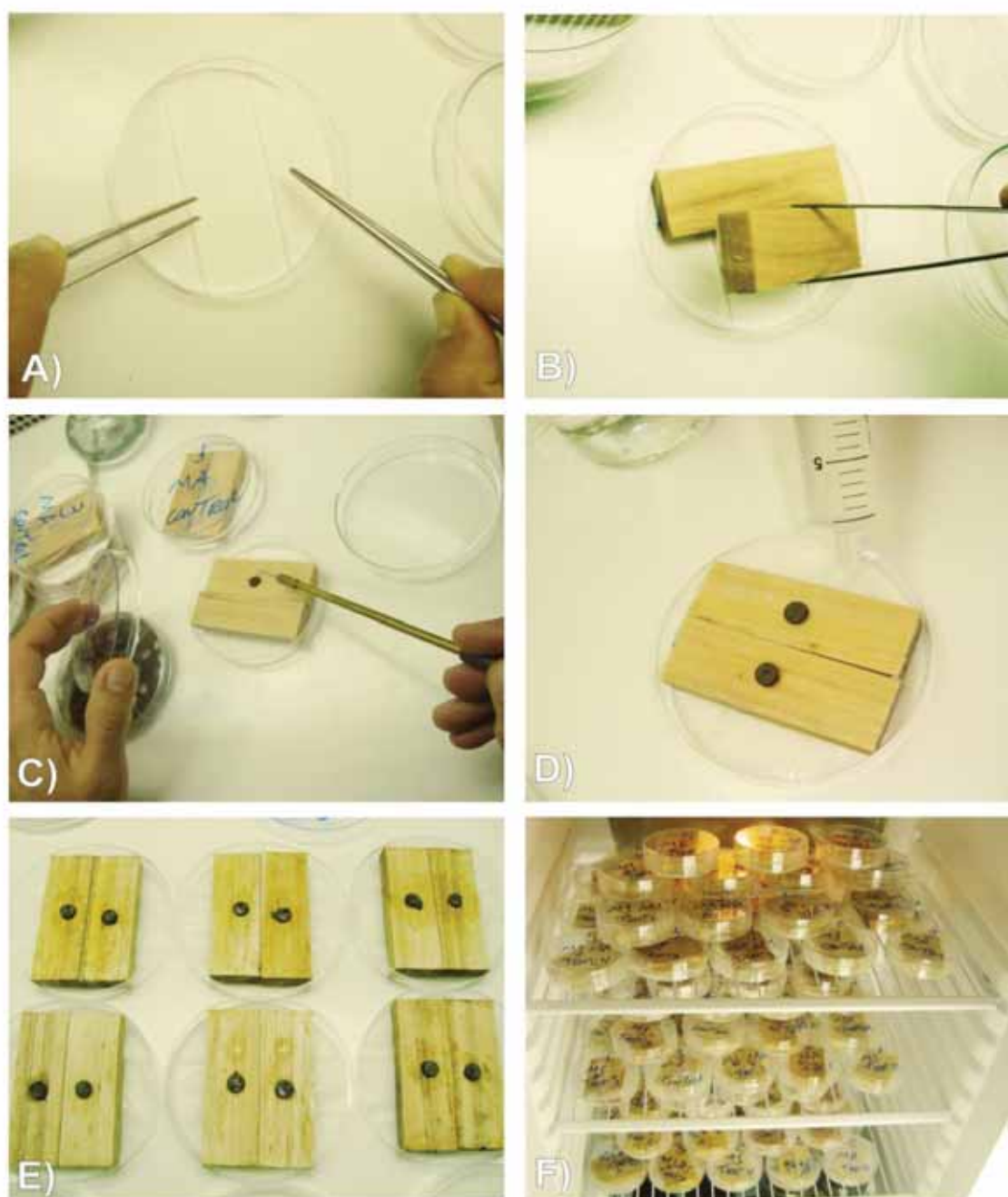
Figura 11. A) Disposição dos bastões de vidro sobre o papel filtro; B) Acomodações dos corpos de prova sobre os bastões de vidro; C) Inoculação do fungo manchador Botryodiplodia theobromae sobre a superfície da madeira; D) Umidecendo os papeis filtro com água destilada; E) Corpos de prova inoculados e E) Ensaio montado e acomodado dentro da BOD com as condições de umidade e temperatura controlada.
