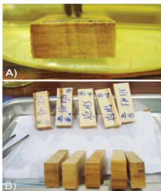
Figura 10. A) Detalhe do tratamento de imersão sobre o corpo de prova e B) Acomodação dos corpos de prova sobre a bandeija de alumínio a fim de retirar o excesso da solução.
