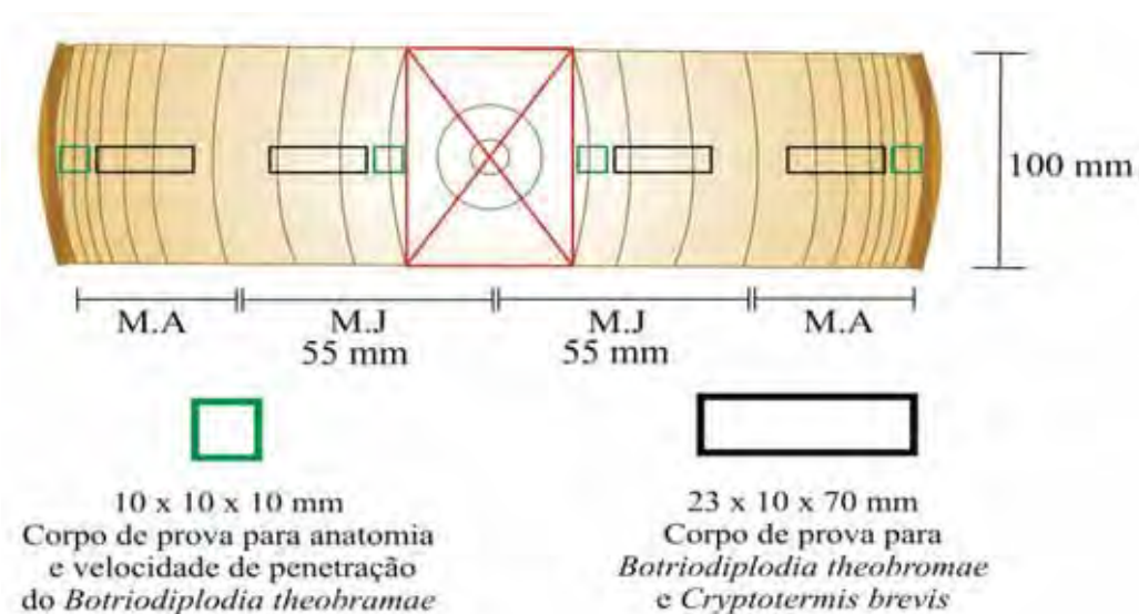
Figura 7. Esquema para a retirada dos corpos de prova para o material em estudo.
